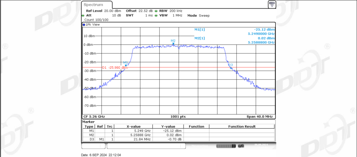
11AX20MIMO_Ant2_5260
