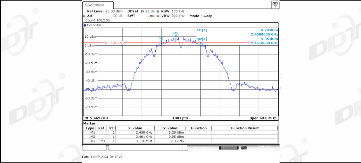
11B_Ant2_2462
