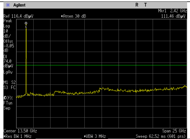
WIFI_2437MHz_20MHz_b-mode_Peak_Ant B
