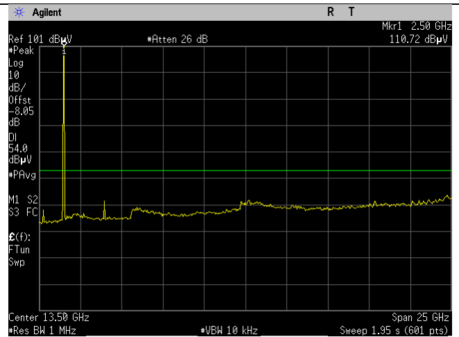
BLE_2480MHz_2MBit_1-26GHz_Avg_Ant BLE
