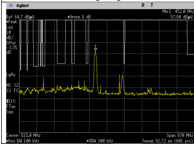
WIFI_2412MHz_20MHz_g-mode_15.209_30- 1000MHz_Peak_Ant A
