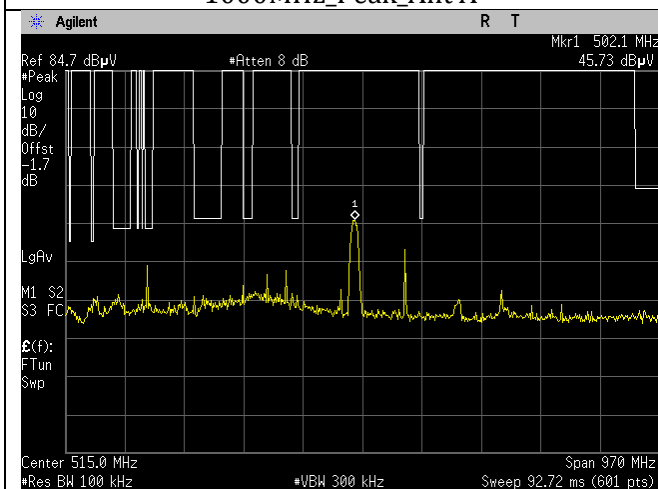
WIFI_2462MHz_20MHz_n-mode_15.209_30-1000MHz_Peak_Ant A
