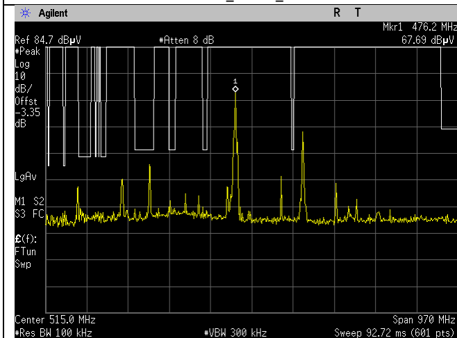
WIFI_2437MHz_20MHz_b-mode_15.209_30-1000MHz_Peak_Ant A
