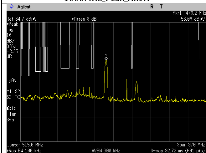
WIFI_2437MHz_20MHz_g-mode_15.209_30-1000MHz_Peak_Ant A
