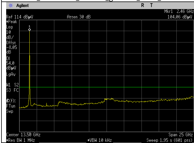
WIFI_2462MHz_20MHz_g-mode_Avg_Ant A
