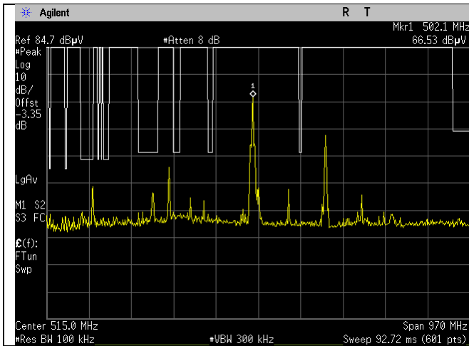
WIFI_2462MHz_20MHz_b-mode_15.209_30-1000MHz_Peak_Ant A
