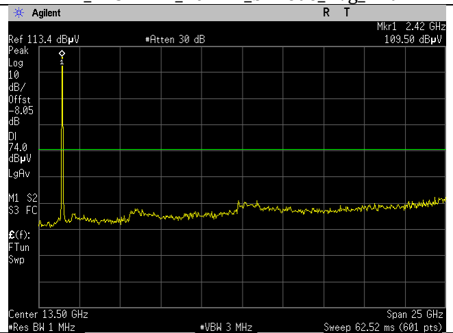
WIFI_2437MHz_20MHz_g-mode_Peak_Ant B
