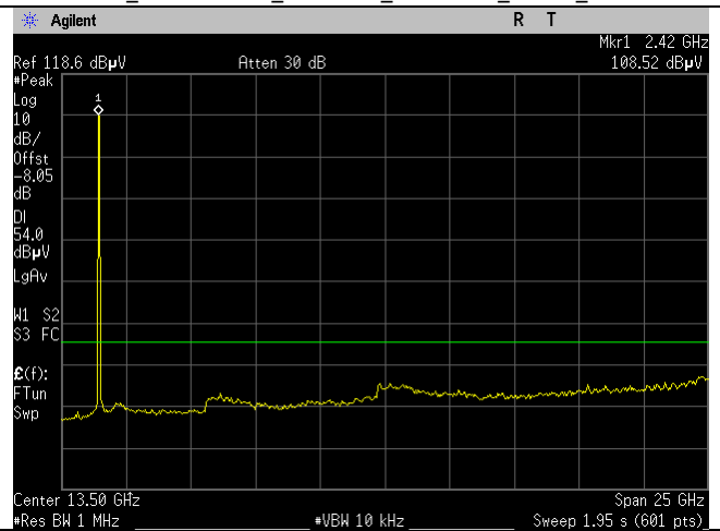
WIFI_2437MHz_20MHz_b-mode_Avg_Ant B
