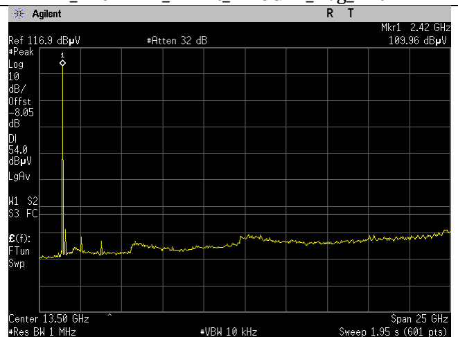
BLE_2402MHz_2MBit_1-26GHz_Avg_Ant BLE
