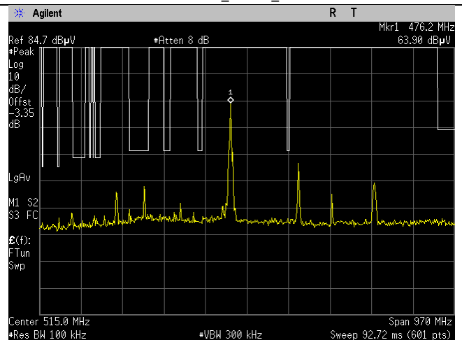
WIFI_2437MHz_20MHz_b-mode_15.209_30-1000MHz_Peak_Ant B
