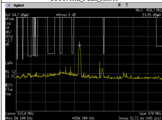
WIFI_2412MHz_20MHz_n-mode_15.209_30- 1000MHz_Peak_Ant A
