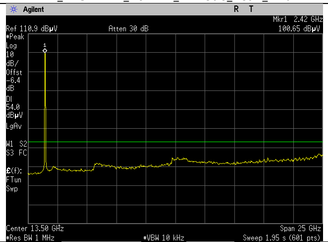
WIFI_2437MHz_20MHz_n-mode_Avg_Ant B
