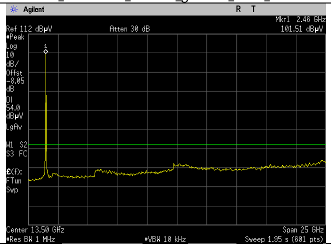
WIFI_2462MHz_20MHz_g-mode_Avg_Ant B
