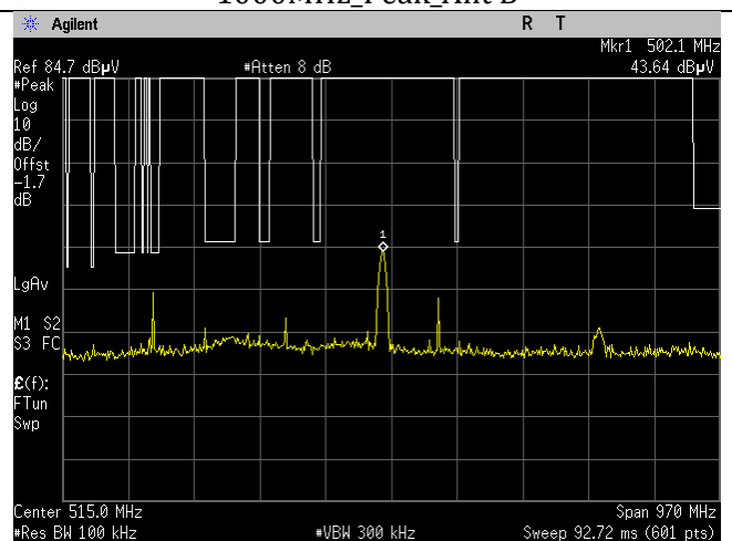
WIFI_2462MHz_20MHz_n-mode_15.209_30-1000MHz_Peak_Ant B
