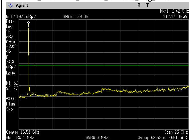
WIFI_2437MHz_20MHz_g-mode_Peak_Ant A
