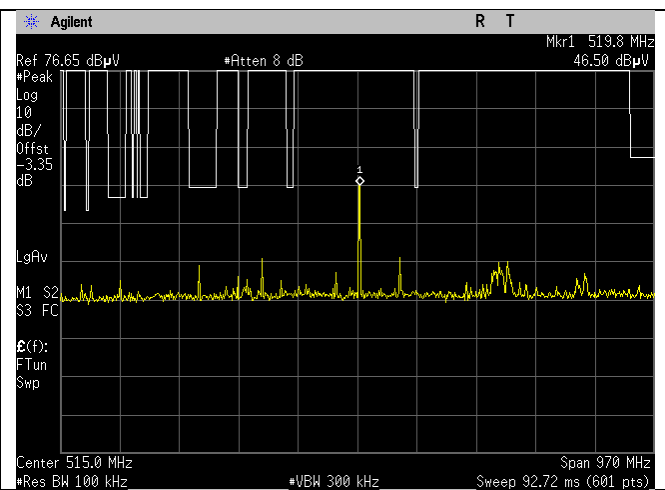
BLE_2480MHz_2MBit_30-1000MHz_Peak_Ant BLE
