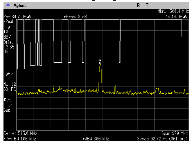
WIFI_2462MHz_20MHz_g-mode_15.209_30-1000MHz_Peak_Ant B
