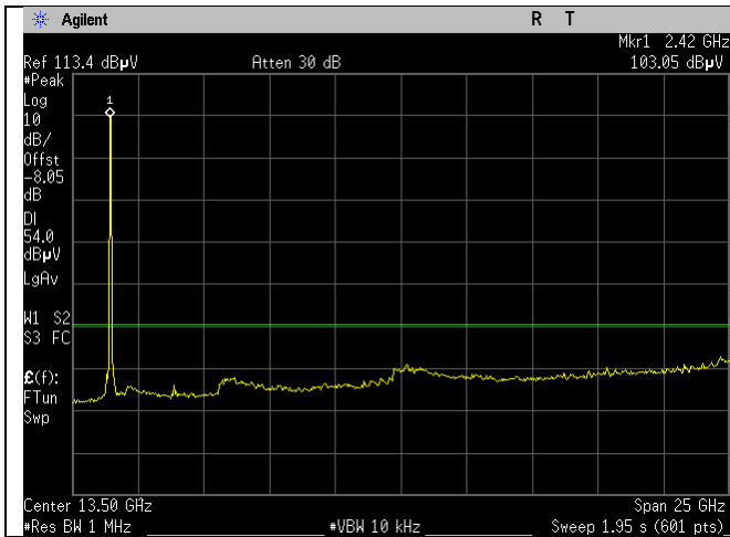
WIFI_2437MHz_20MHz_g-mode_Avg_Ant A
