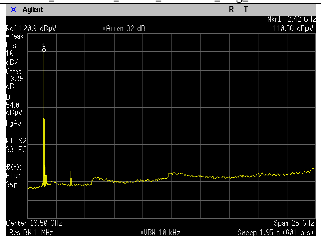
BLE_2402MHz_1MBit_1-26GHz_Avg_Ant BLE
