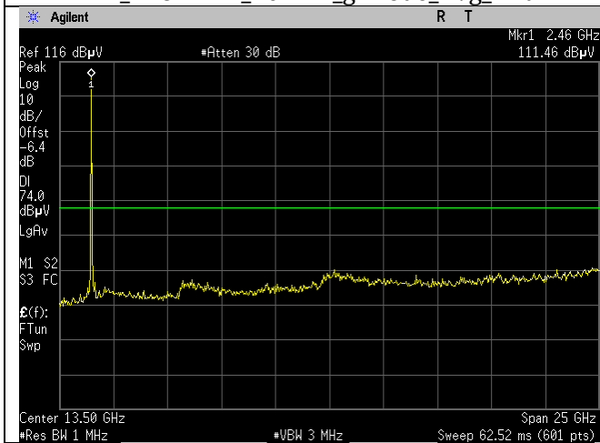
WIFI_2462MHz_20MHz_n-mode_Peak_Ant A
