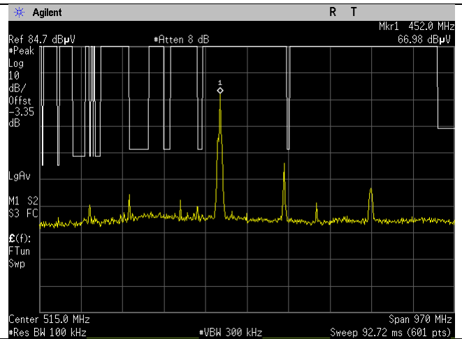
WIFI_2412MHz_20MHz_b-mode_15.209_30- 1000MHz_Peak_Ant B
