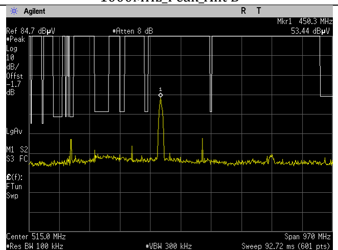
WIFI_2412MHz_20MHz_n-mode_15.209_30- 1000MHz_Peak_Ant B
