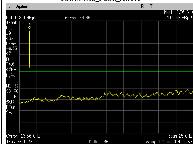
BLE_2480MHz_1MBit_1-26GHz_Peak_Ant BLE
