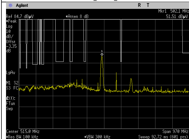
WIFI_2462MHz_20MHz_g-mode_15.209_30-1000MHz_Peak_Ant A
