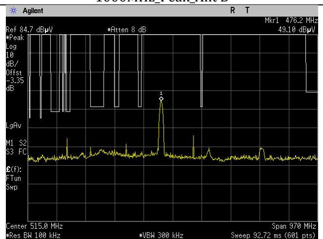
WIFI_2437MHz_20MHz_g-mode_15.209_30-1000MHz_Peak_Ant B
