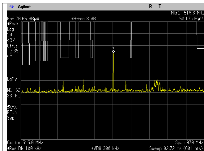
BLE_2480MHz_1MBit_30-1000MHz_Peak_Ant BLE
