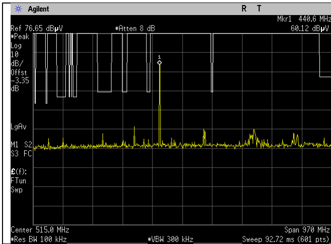
BLE_2402MHz_1MBit_30-1000MHz_Peak_Ant BLE
