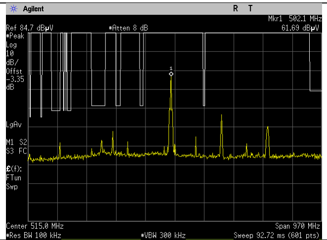
WIFI_2462MHz_20MHz_b-mode_15.209_30-1000MHz_Peak_Ant B
