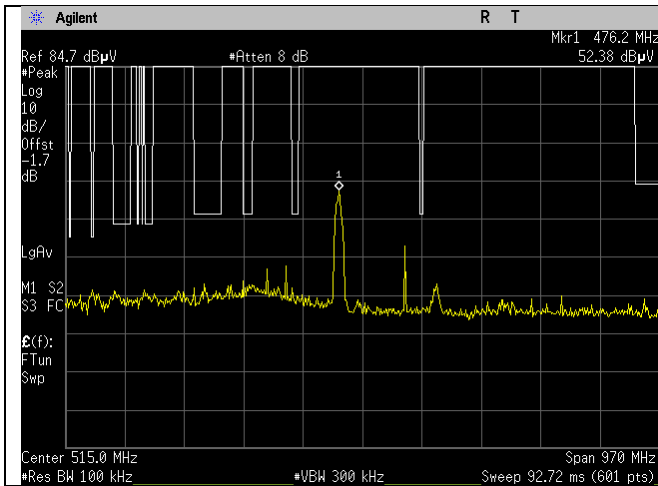
WIFI_2437MHz_20MHz_n-mode_15.209_30- 1000MHz_Peak_Ant A
