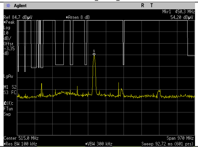
WIFI_2412MHz_20MHz_g-mode_15.209_30- 1000MHz_Peak_Ant B
