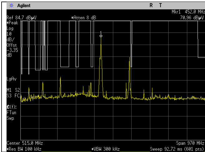
WIFI_2412MHz_20MHz_b-mode_15.209_30- 1000MHz_Peak_Ant A
