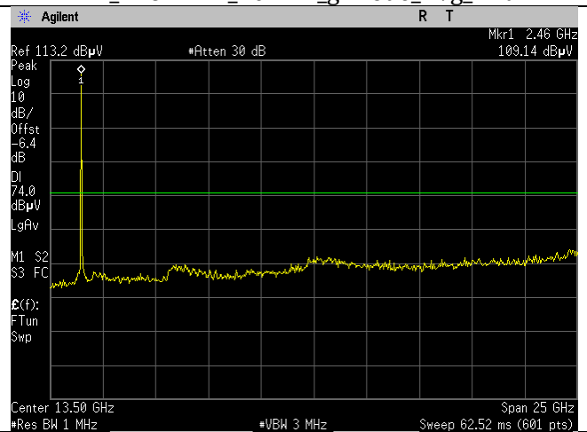
WIFI_2462MHz_20MHz_n-mode_Peak_Ant B
