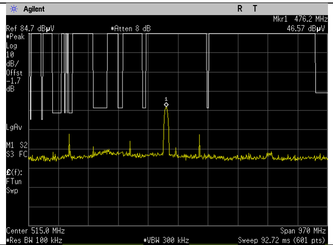
WIFI_2437MHz_20MHz_n-mode_15.209_30- 1000MHz_Peak_Ant B
