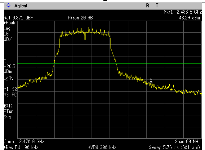
WIFI_2462MHz_20MHz_g-mode_Upper Band Edge_Ant B
