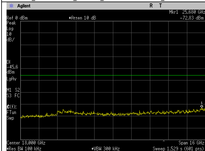
BLE_2402MHz_1MBit_10-26GHz_Ant BLE
