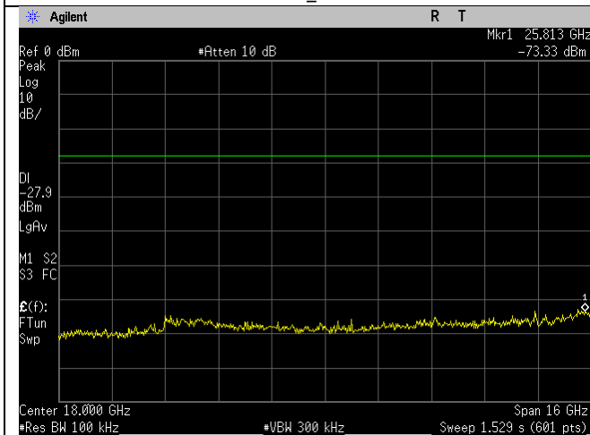
WIFI_2437MHz_20MHz_g-mode_10-26GHz_Ant A
