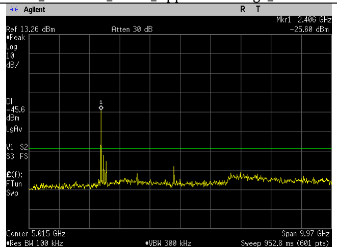
BLE_2402MHz_1MBit_30MHz-10GHz_Ant BLE
