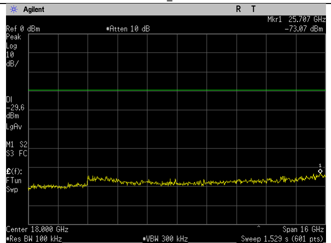
WIFI_2437MHz_20MHz_g-mode_10-26GHz_Ant B
