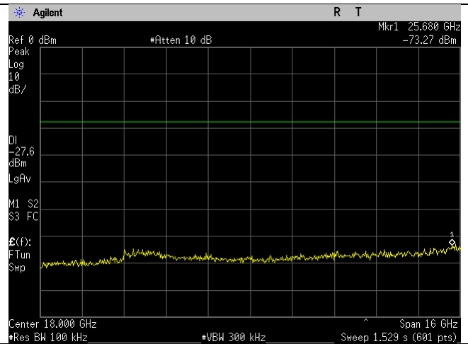
WIFI_2412MHz_20MHz_g-mode_10-26GHz_Ant B
