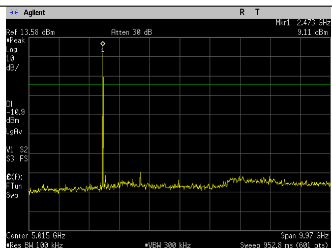
BLE_2480MHz_1MBit_30MHz-10GHz_Ant BLE
