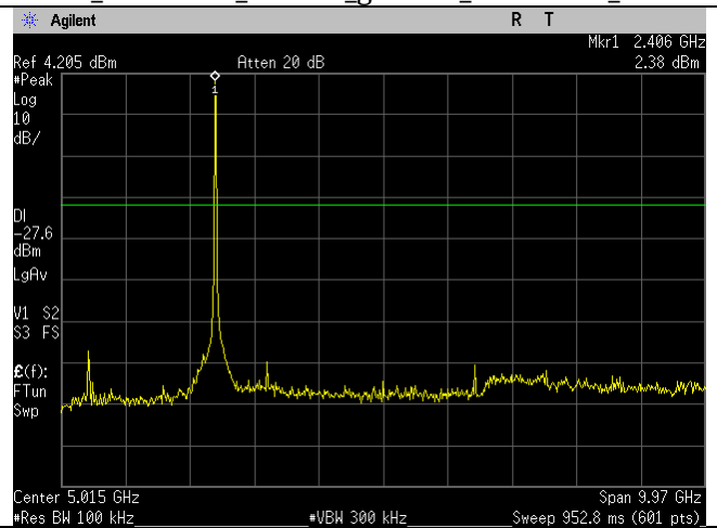
WIFI_2412MHz_20MHz_g-mode_30MHz-10GHz_Ant B
