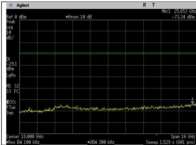
WIFI_2412MHz_20MHz_g-mode_10-26GHz_Ant A
