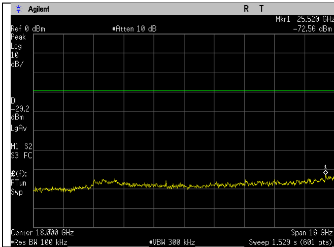
WIFI_2462MHz_20MHz_g-mode_10-26GHz_Ant A
