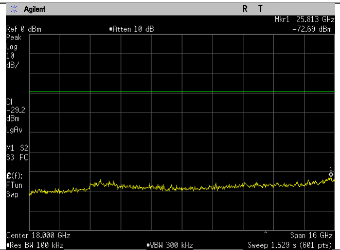
WIFI_2462MHz_20MHz_g-mode_10-26GHz_Ant B
