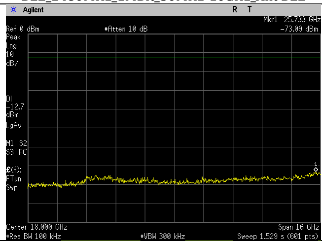
BLE_2480MHz_2MBit_10-26GHz_Ant BLE
