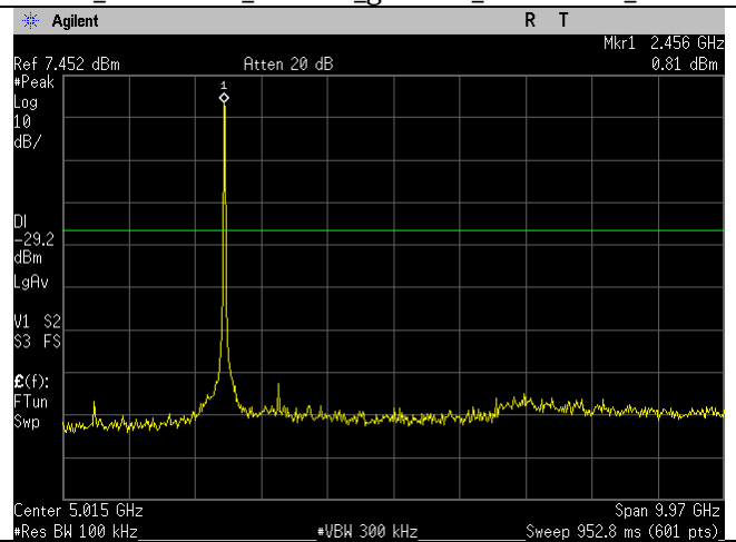
WIFI_2462MHz_20MHz_g-mode_30MHz-10GHz_Ant B
