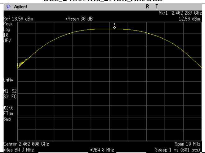
BLE_2402MHz_2MBit_Ant BLE
