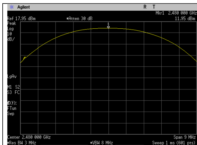
BLE_2480MHz_1Mbit_Ant BLE
