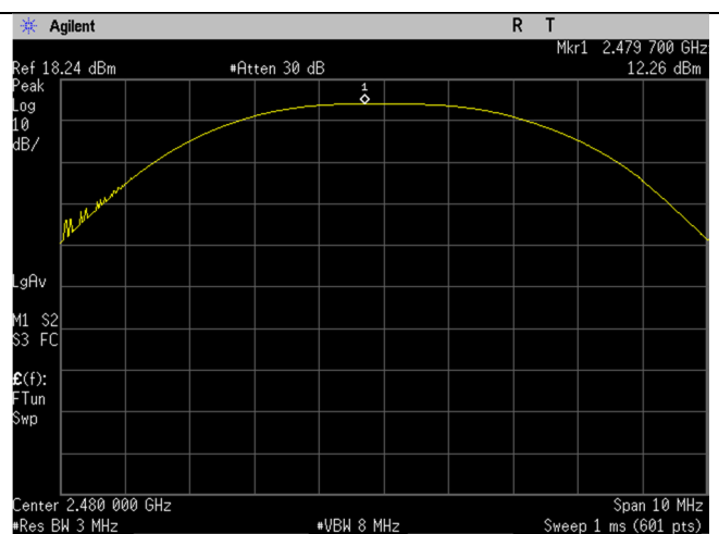
BLE_2480MHz_2MBit_Ant BLE
