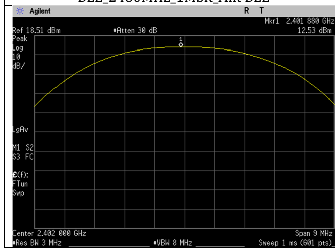
BLE_2402MHz_1MBit_Ant BLE
