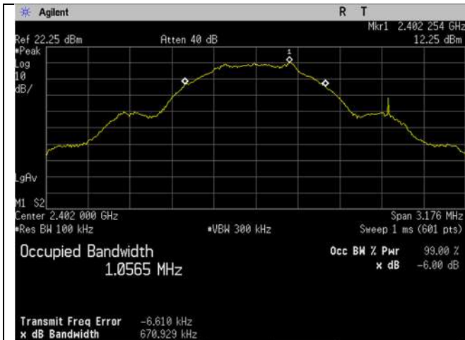
BLE_2402MHz_1MBit_-6dB_Ant BLE
