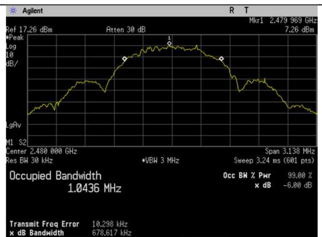
BLE_2480MHz_1MBit_99 percent_Ant BLE
