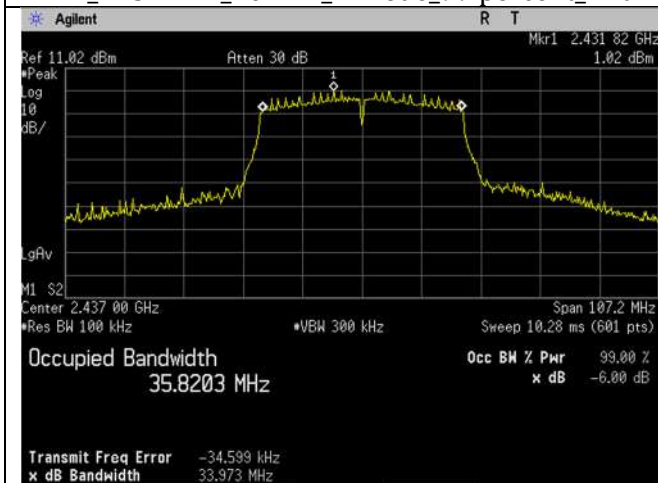
WIFI_2437MHz_40MHz_n-mode -6dB Ant A
