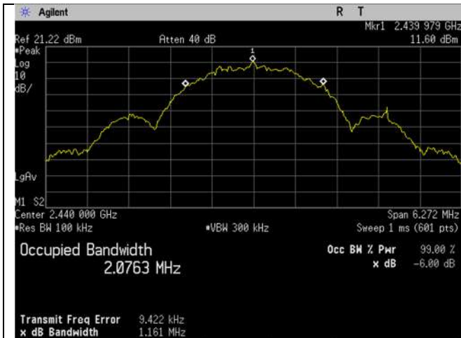
BLE_2440MHz_2MBit_-6dB_Ant BLE
