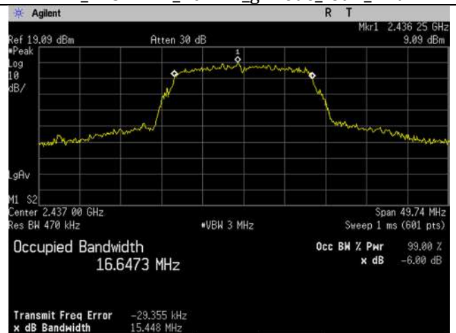
WIFI_2437MHz_20MHz_g-mode_99 percent_Ant B
