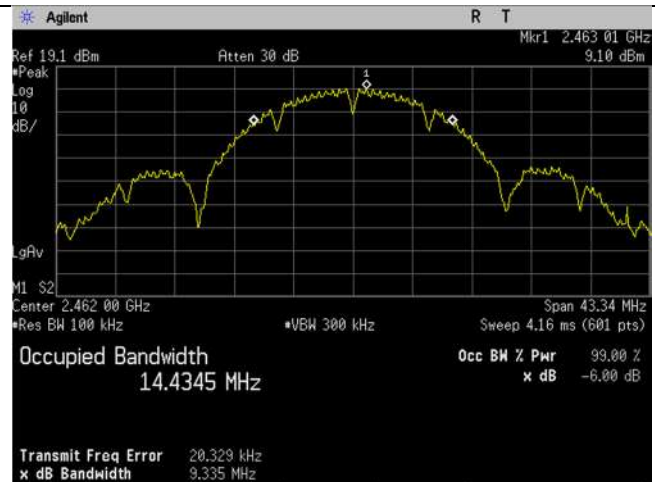
WIFI_2462MHz_20MHz_b-mode -6dB Ant B
