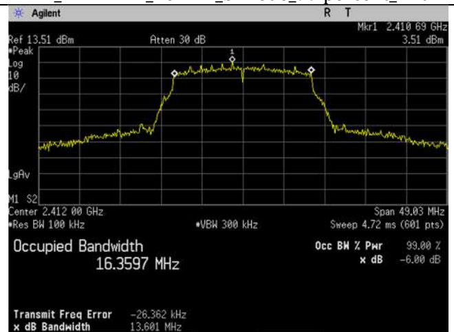
WIFI_2412MHz_20MHz_g-mode -6dB Ant B
