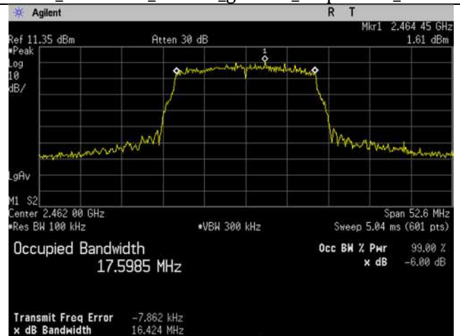
WIFI_2462MHz_20MHz_n-mode_-6dB_Ant B
