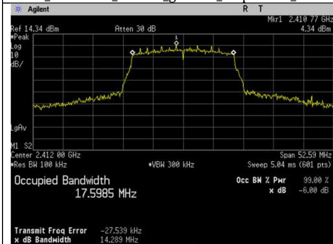
WIFI_2412MHz_20MHz_n-mode_-6dB_Ant A
