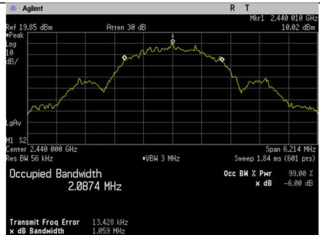
BLE_2440MHz_2MBit_99 percent_Ant BLE
