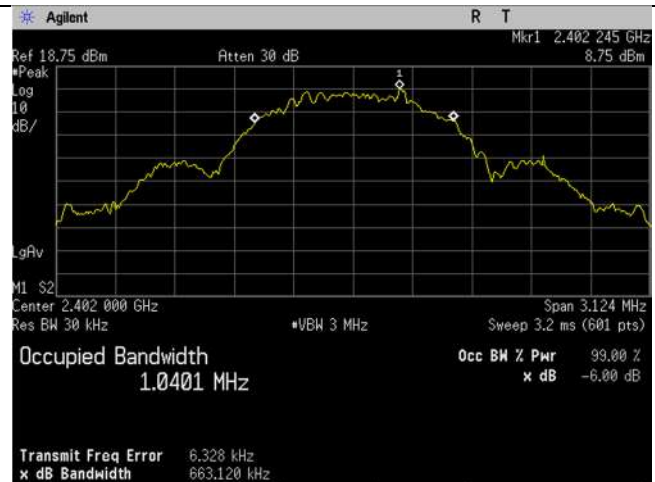
BLE_2402MHz_1MBit_99 percent_Ant BLE
