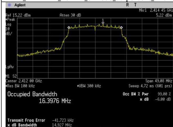
WIFI_2412MHz_20MHz_g-mode -6dB Ant A
