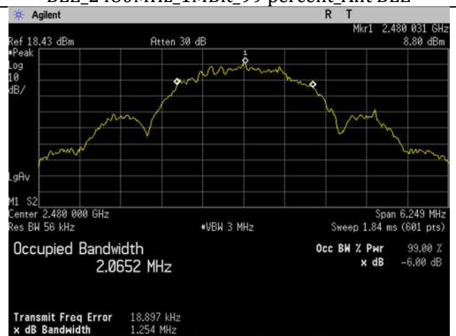
BLE_2480MHz_2MBit_99 percent_Ant BLE
