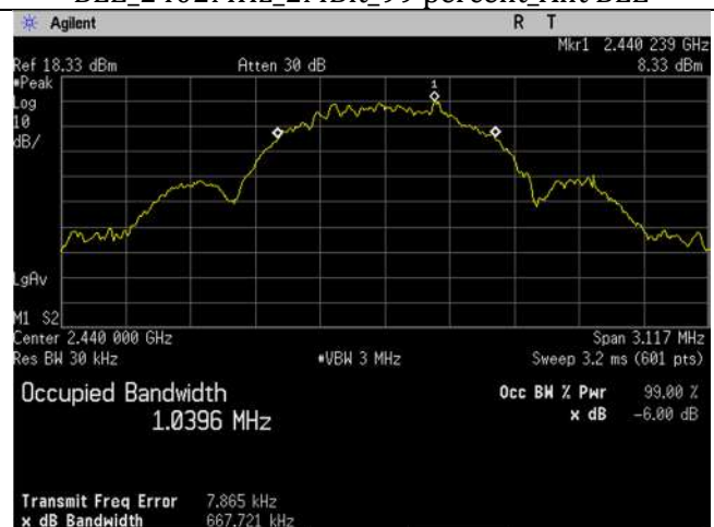
BLE_2440MHz_1MBit_99 percent_Ant BLE
