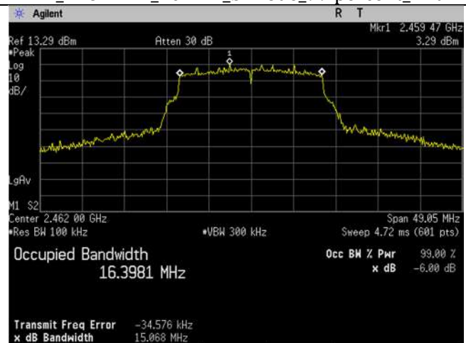
WIFI_2462MHz_20MHz_g-mode -6dB Ant B
