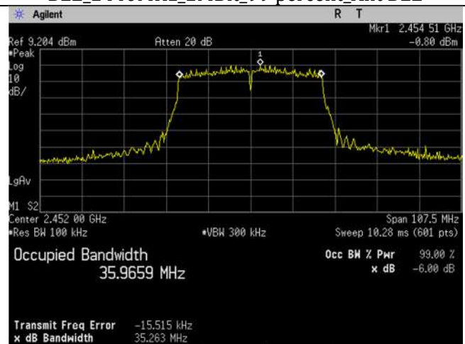
WIFI_2452MHz_40MHz_n-mode_-6dB_Ant B
