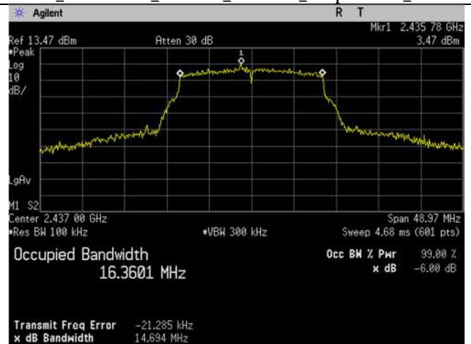
WIFI_2437MHz_20MHz_g-mode_-6dB_Ant B
