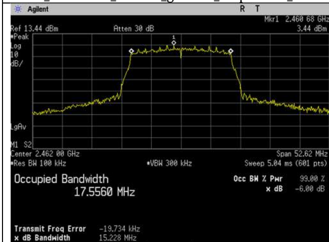
WIFI_2462MHz_20MHz_n-mode_-6dB_Ant A
