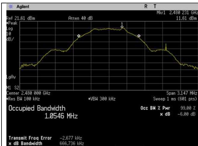
BLE_2480MHz_1MBit_-6dB_Ant BLE
