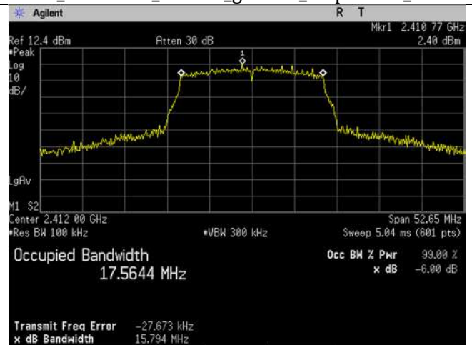
WIFI_2412MHz_20MHz_n-mode_-6dB_Ant B
