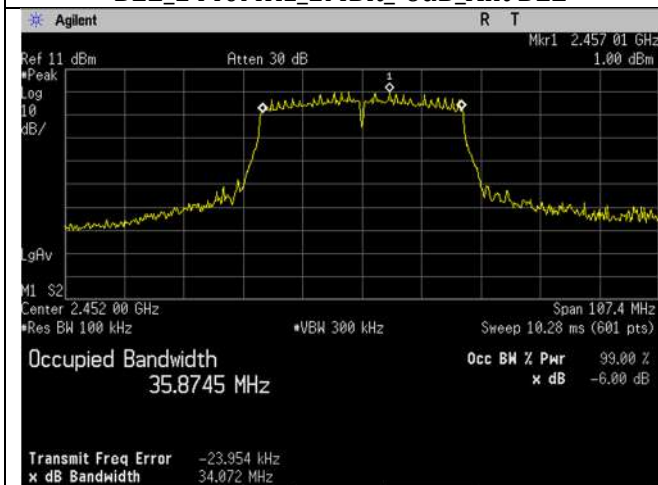
WIFI_2452MHz_40MHz_n-mode_-6dB_Ant A
