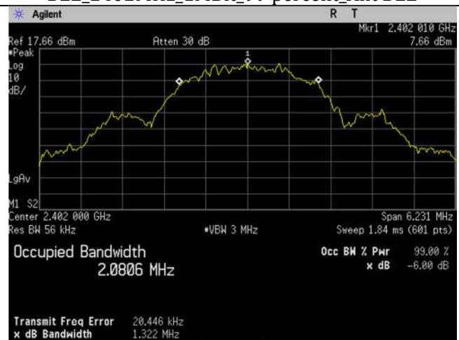
BLE_2402MHz_2MBit_99 percent_Ant BLE
