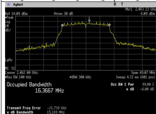
WIFI_2462MHz_20MHz_g-mode -6dB Ant A
