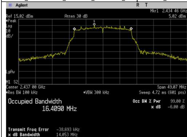
WIFI_2437MHz_20MHz_g-mode_-6dB_Ant A
