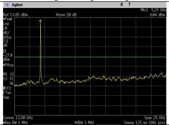
5310MHz_n40-mode_1-26GHz_Ant B
