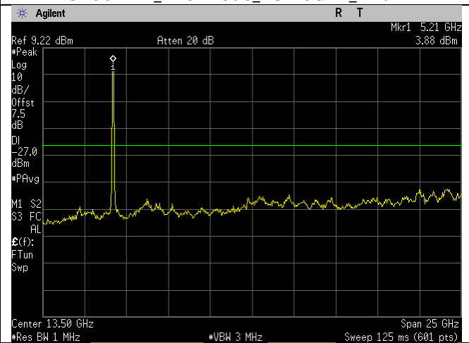
5210MHz_ac80-mode_1-26GHz_Ant B
