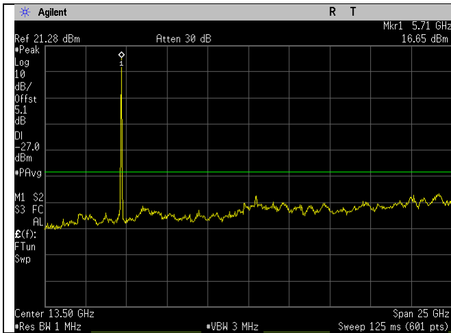
5700MHz_a-mode_1-26GHz_Ant A
