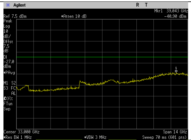
5210MHz_ac80-mode_26-40GHz Ant B
