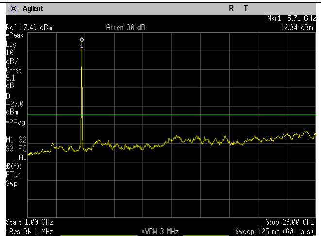
5700MHz_a-mode_1-26GHz_Ant B
