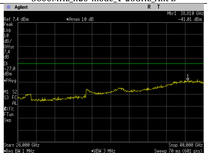
5600MHz_n20-mode_26-40GHz_Ant B
