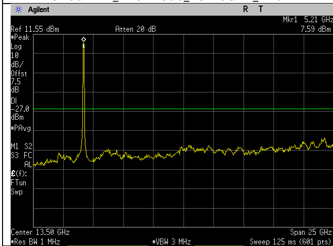
5210MHz_ac80-mode_1-26GHz_Ant A
