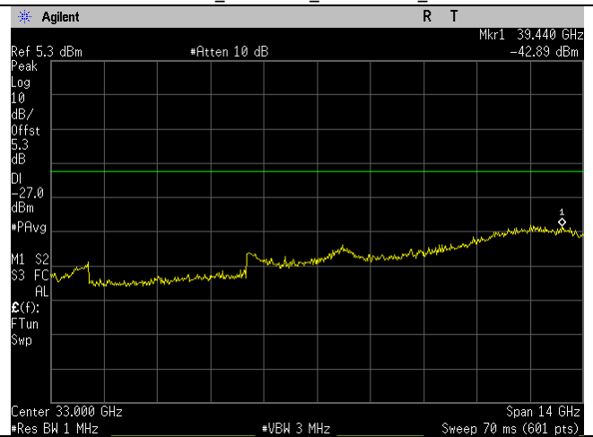
5320MHz_a-mode_26-40GHz_Ant B
