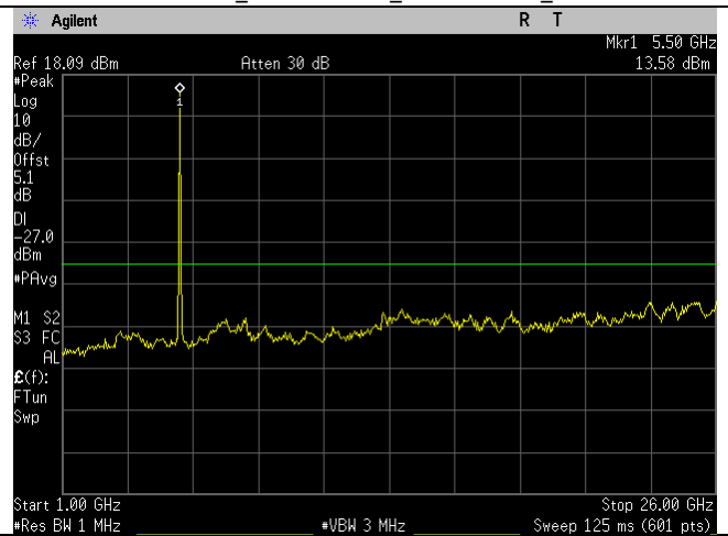
5500MHz_a-mode_1-26GHz_Ant B
