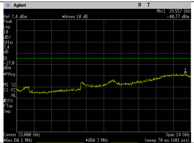
5610MHz_ac80-mode_26-40GHz_Ant B
