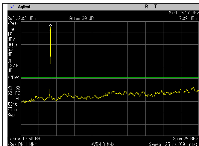
5180MHz_a-mode_1-26GHz_Ant A
