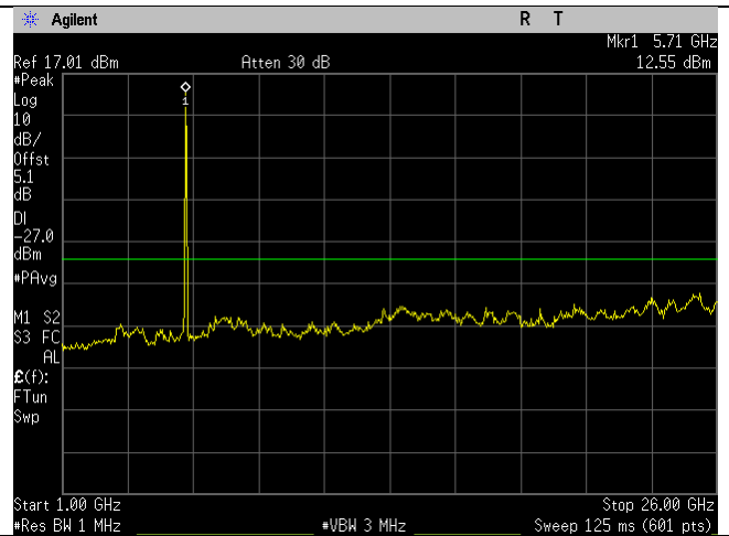
5720MHz_a-mode_1-26GHz_Ant B
