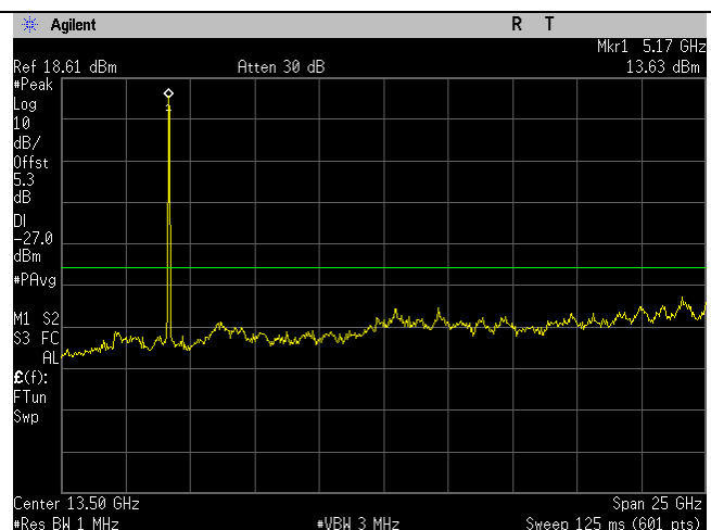
5180MHz_a-mode_1-26GHz_Ant B
