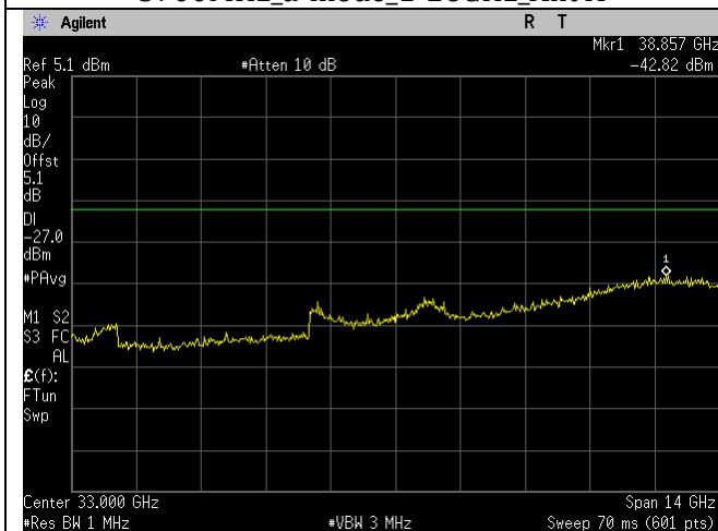
5700MHz_a-mode_26-40GHz_Ant A
