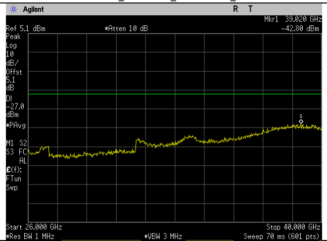
5720MHz_a-mode_26-40GHz_Ant B
