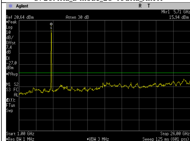
5720MHz_n20-mode_1-26GHz_Ant A
