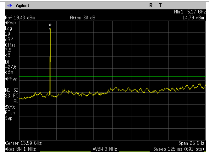
5180MHz_n20-mode_1-26GHz_Ant B
