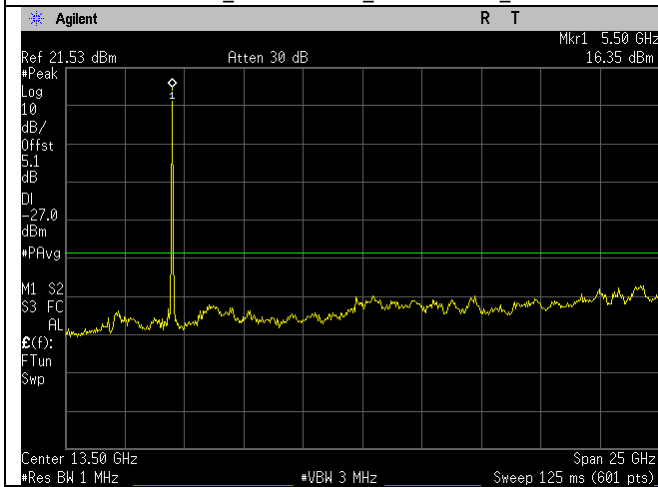
5500MHz_a-mode_1-26GHz_Ant A
