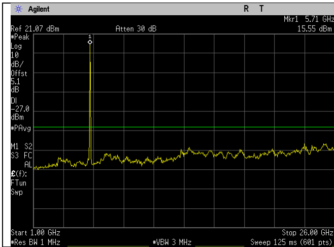
5720MHz_a-mode_1-26GHz_Ant A
