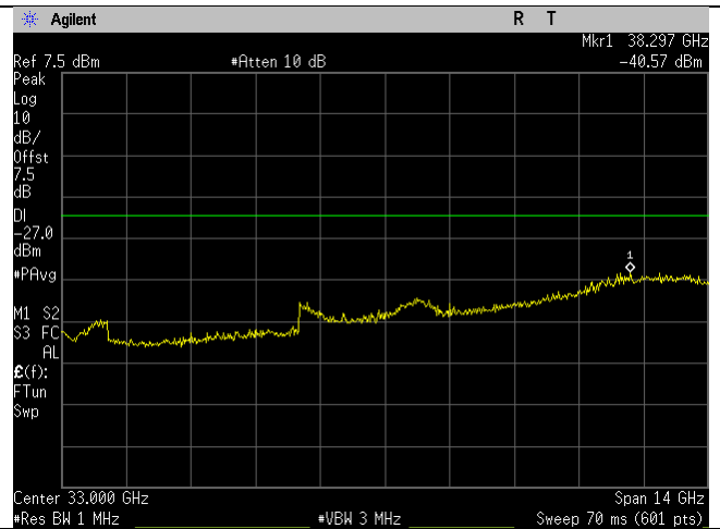
5270MHz_n40-mode_26-40GHz_Ant B
