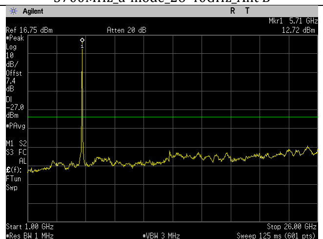
5700MHz_n20-mode_1-26GHz_Ant B
