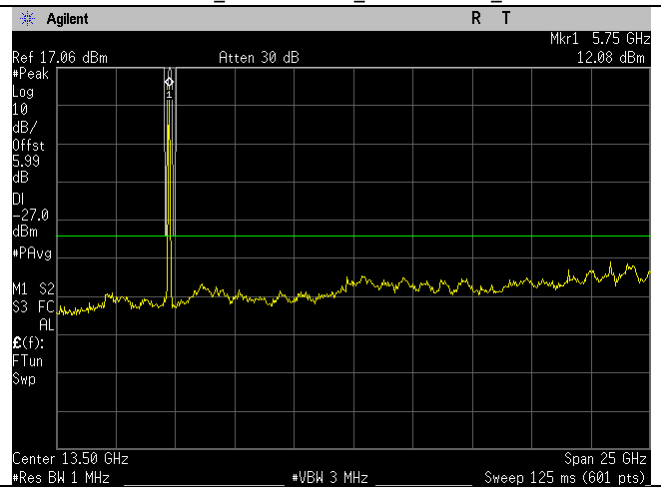
5745MHz_a-mode_1-26GHz_Ant B
