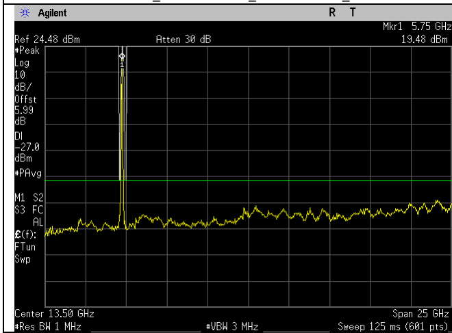
5745MHz_a-mode_1-26GHz_Ant A
