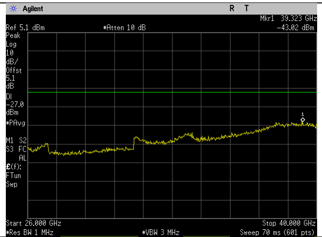
5600MHz_a-mode_26-40GHz_Ant B
