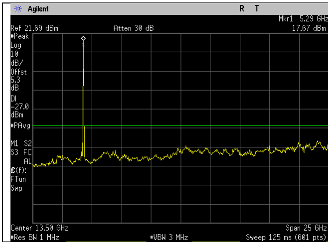
5300MHz_a-mode_1-26GHz_Ant A
