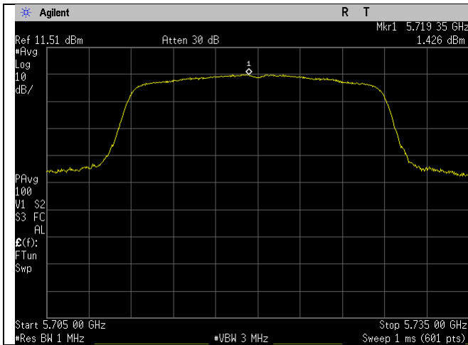
5720MHz_n20-mode_Ant A
