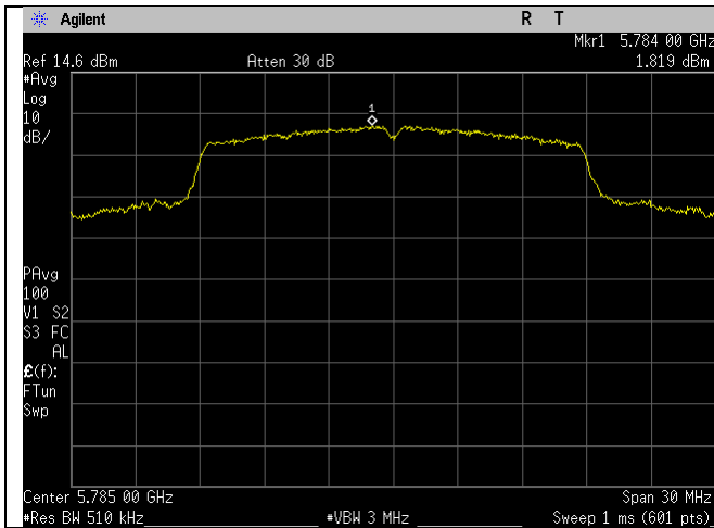
5785MHz_n20-mode_Ant A
