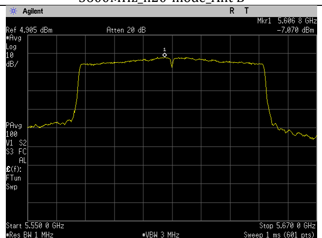
5610MHz_ac80-mode_Ant A
