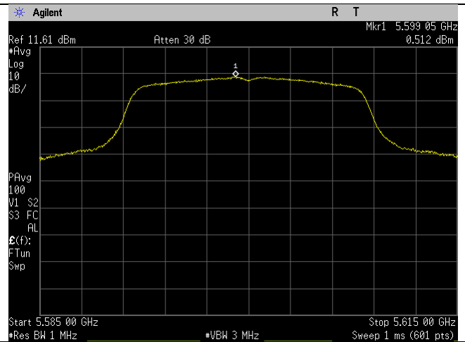
5600MHz_a-mode_Ant B
