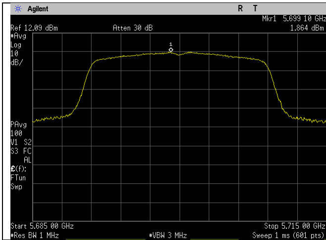
5700MHz_n20-mode_Ant A
