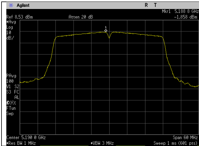
5190MHz_n40-mode_Ant A
