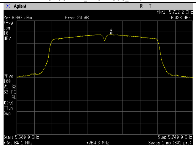
5710MHz_n40-mode_Ant B
