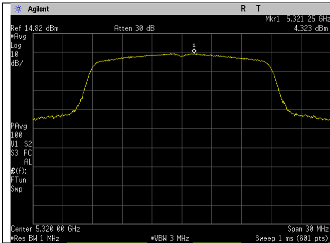
5320MHz_n20-mode_Ant A
