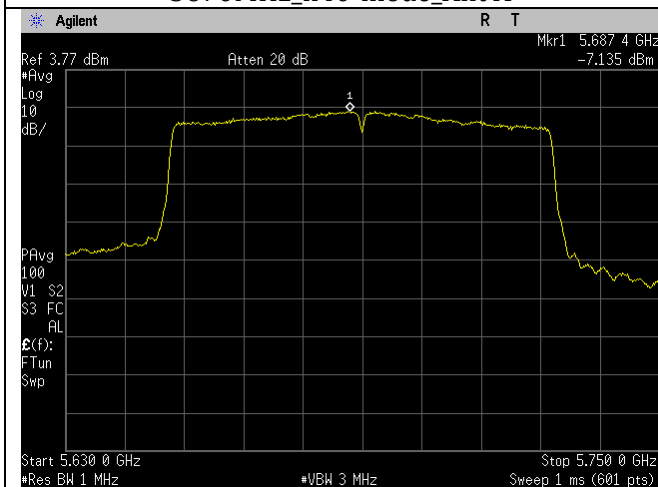
5690MHz_ac80-mode_Ant A
