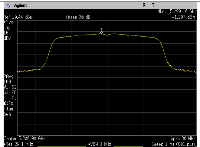
5300MHz_n20-mode_Ant B
