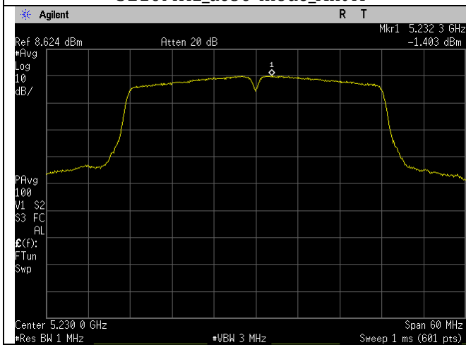
5230MHz_n40-mode_Ant A
