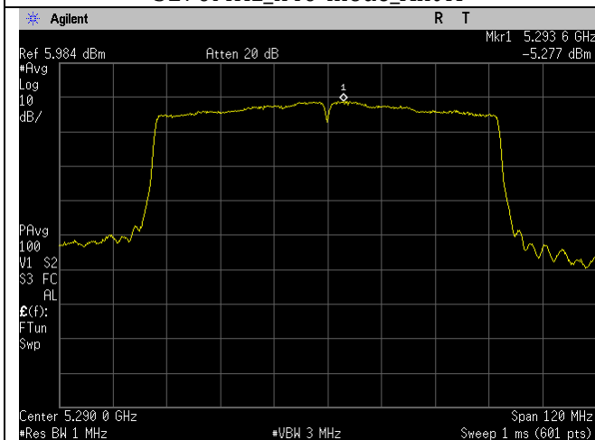
5290MHz_ac80-mode_Ant A
