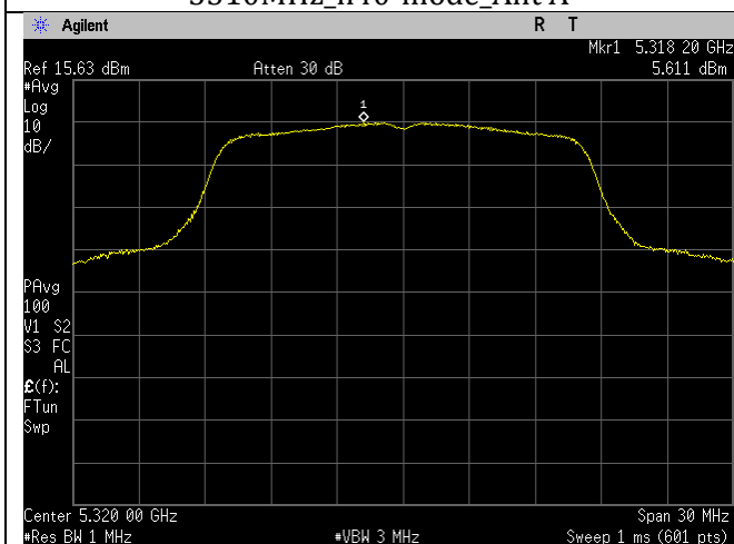
5320MHz_a-mode_Ant A
