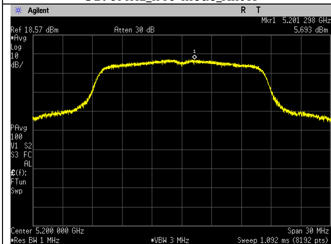
5200MHz_a-mode_Ant A
