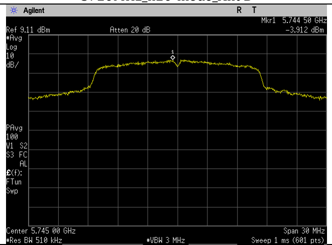
5745MHz_a-mode_Ant B
