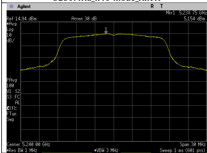
5240MHzCh_48_a-mode_Ant A
