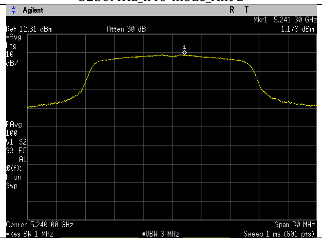
5240MHzCh_48_a-mode_Ant B
