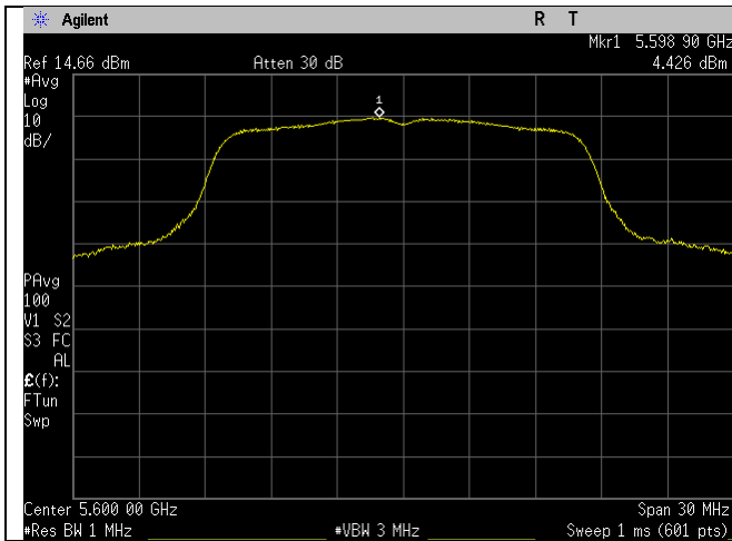
5600MHz_a-mode_Ant A
