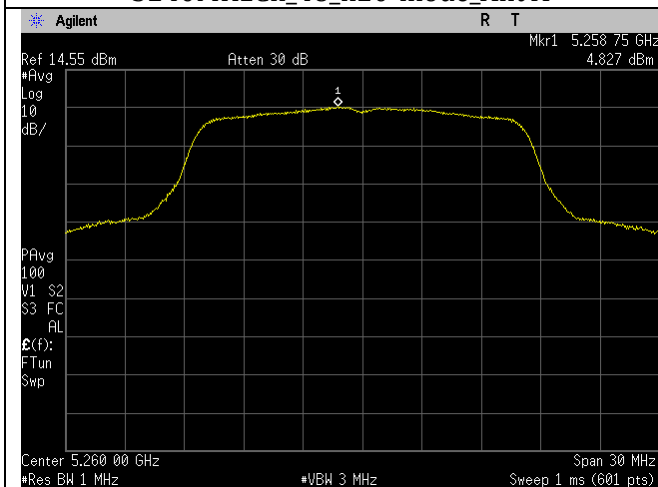
5260MHz_a-mode_Ant A
