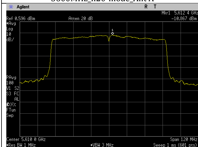
5610MHz_ac80-mode_Ant B
