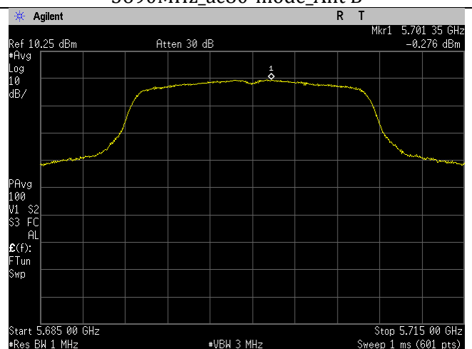
5700MHz_a-mode_Ant B
