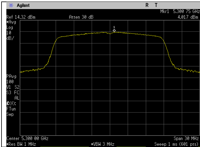
5300MHz_n20-mode_Ant A
