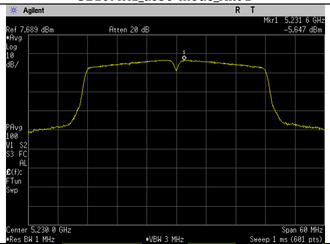
5230MHz_n40-mode_Ant B
