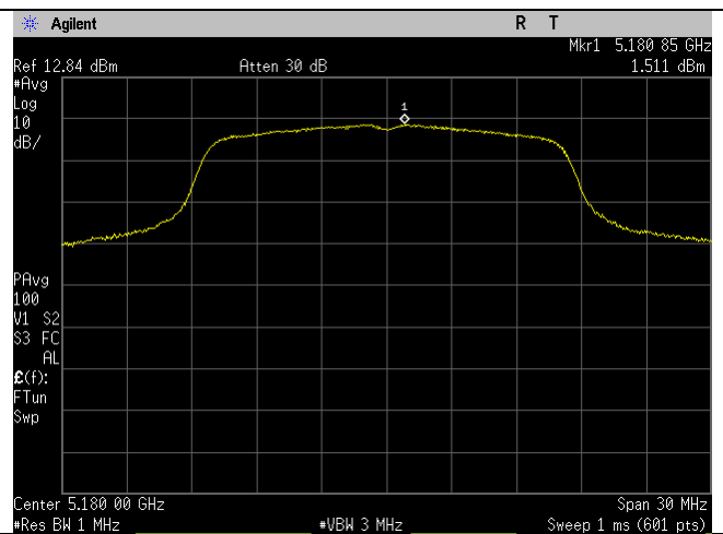
5180MHz_a-mode_Ant B
