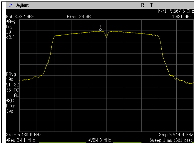
5510MHz_n40-mode_Ant A
