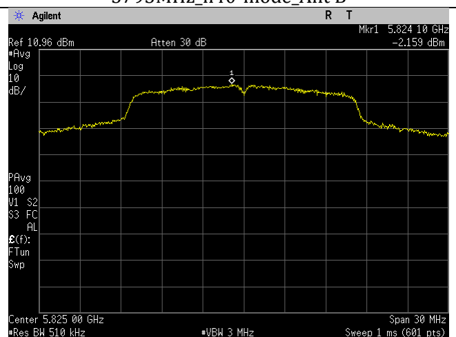
5825MHz_a-mode_Ant B
