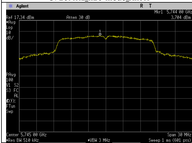
5745MHz_a-mode_Ant A
