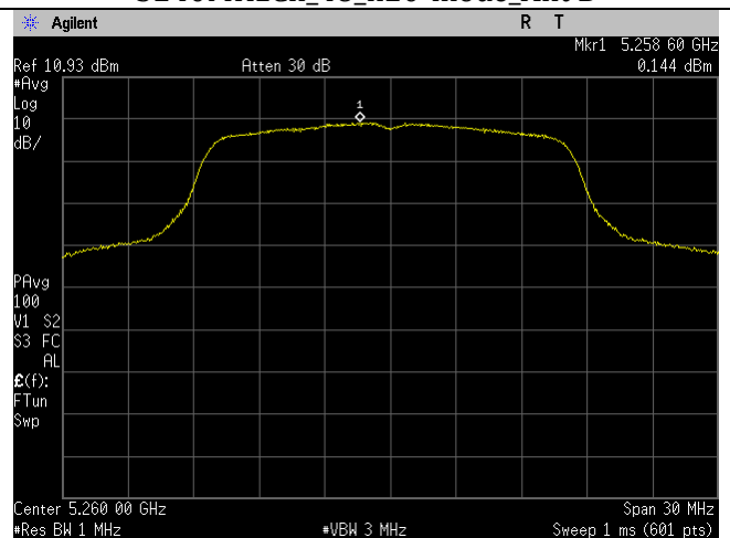
5260MHz_a-mode_Ant B
