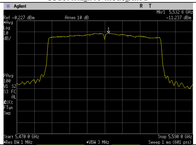
5530MHz_ac80-mode_Ant B
