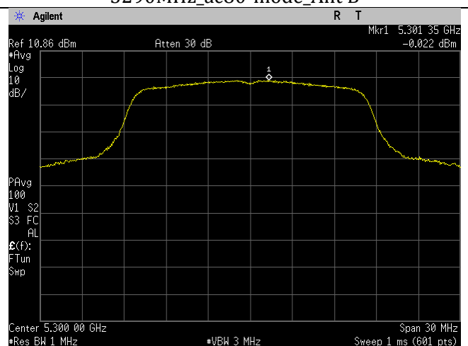
5300MHz_a-mode_Ant B
