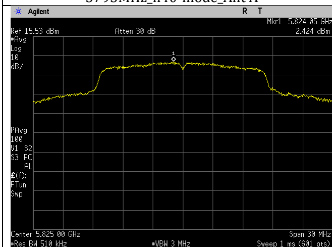
5825MHz_a-mode_Ant A
