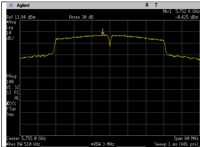
5755MHz_n40-mode_Ant A
