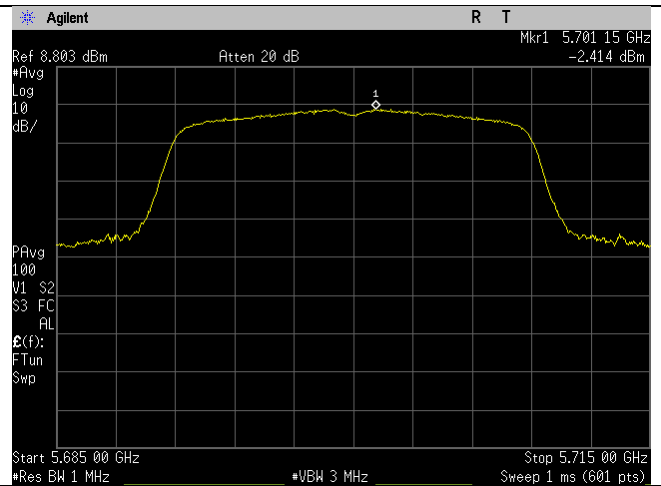
5700MHz_n20-mode_Ant B
