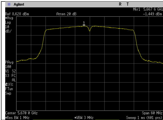
5670MHz_n40-mode_Ant A
