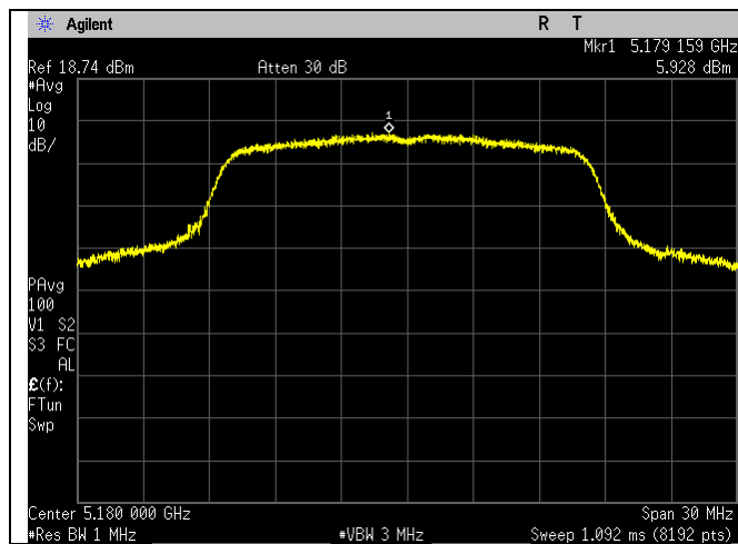
5180MHz_a-mode_Ant A
