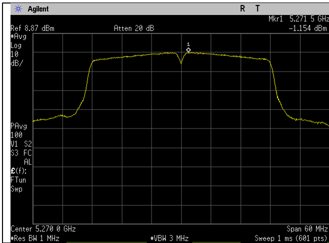
5270MHz_n40-mode_Ant A
