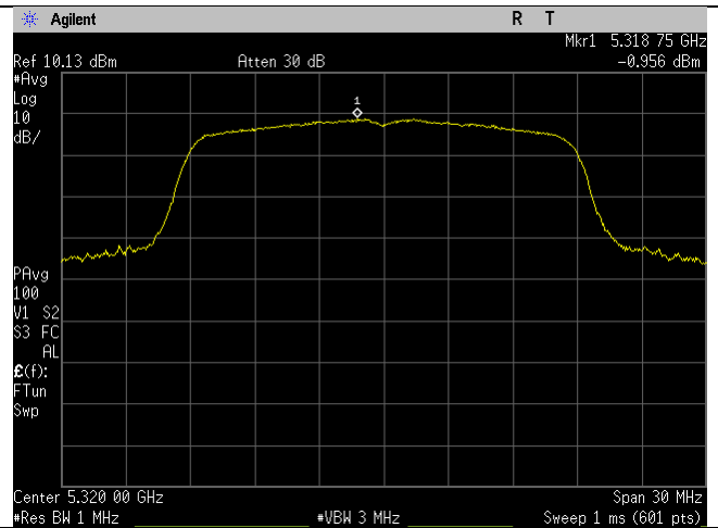
5320MHz_n20-mode_Ant B
