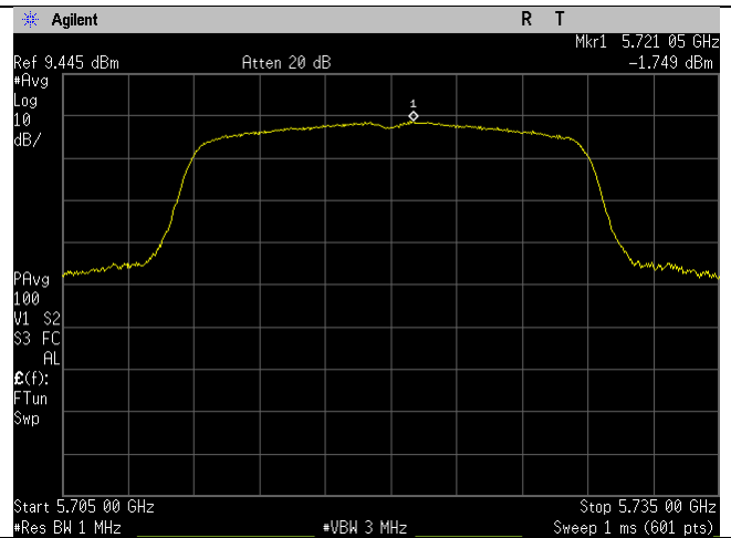
5720MHz_n20-mode_Ant B
