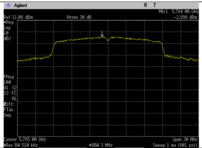
5785MHz_n20-mode_Ant B
