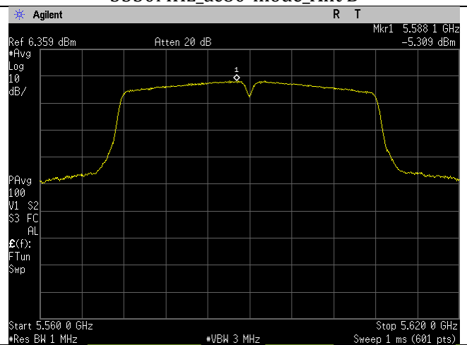
5590MHz_n40-mode_Ant B
