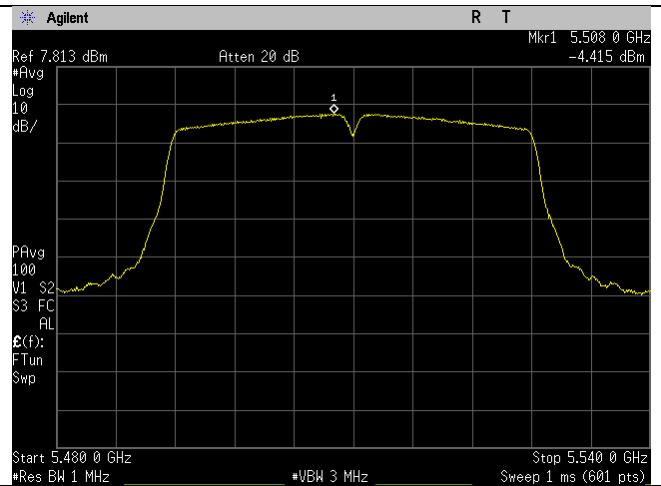
5510MHz_n40-mode_Ant B
