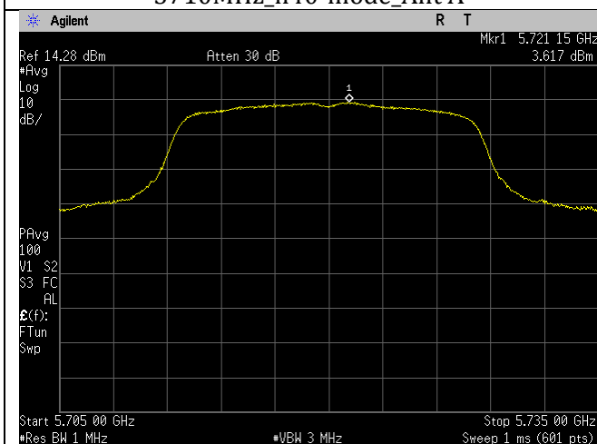
5720MHz_a-mode_Ant A
