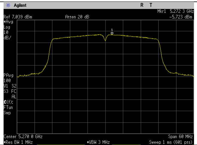
5270MHz_n40-mode_Ant B
