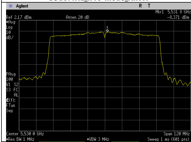
5530MHz_ac80-mode_Ant A
