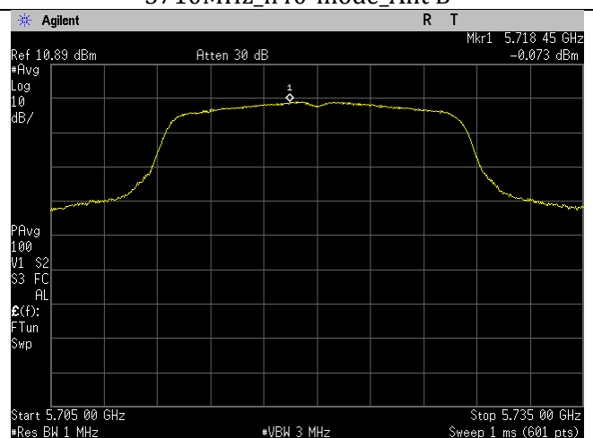
5720MHz_a-mode_Ant B
