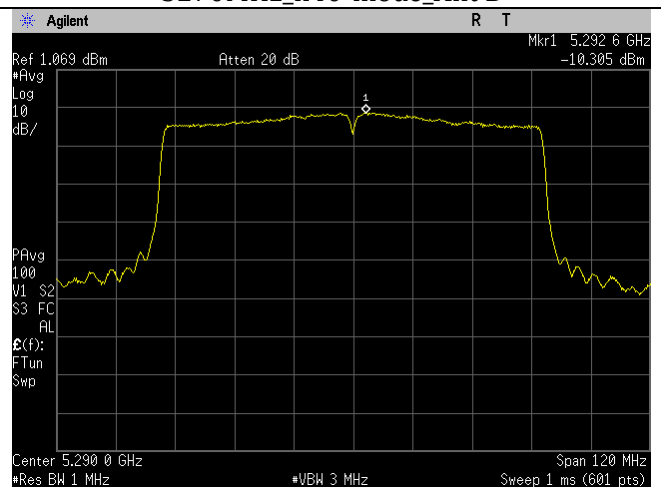
5290MHz_ac80-mode_Ant B
