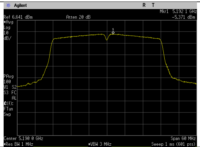
5190MHz_n40-mode_Ant B
