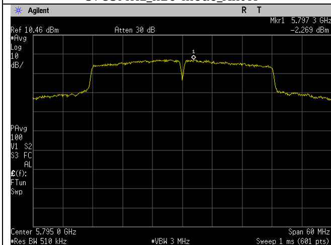
5795MHz_n40-mode_Ant A
