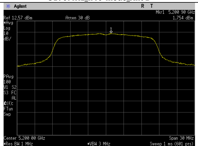
5200MHz_a-mode_Ant B
