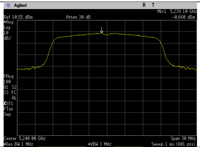
5240MHzCh_48_n20-mode_Ant B
