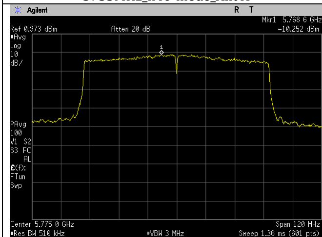
5775MHz_ac80-mode_Ant A
