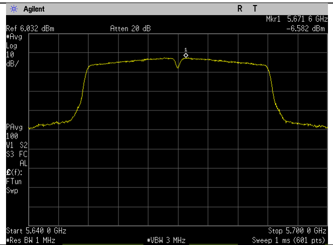
5670MHz_n40-mode_Ant B
