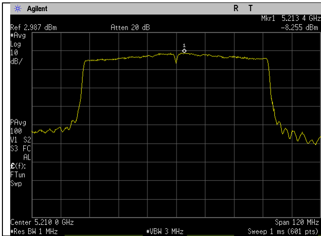
5210MHz_ac80-mode_Ant A
