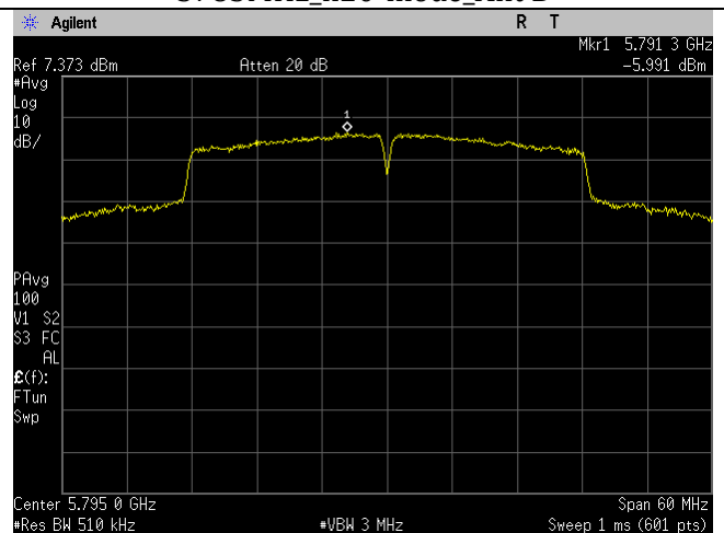
5795MHz_n40-mode_Ant B
