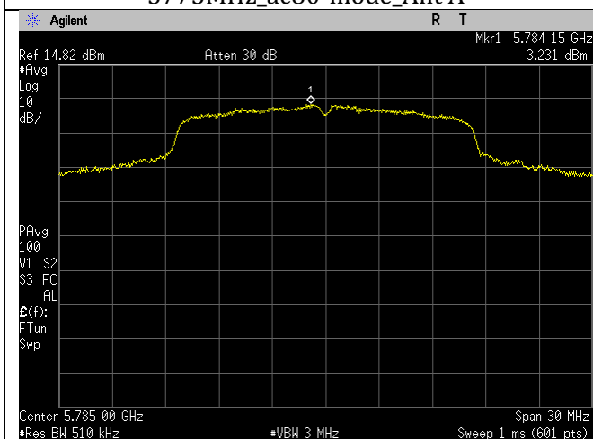
5785MHz_a-mode_Ant A
