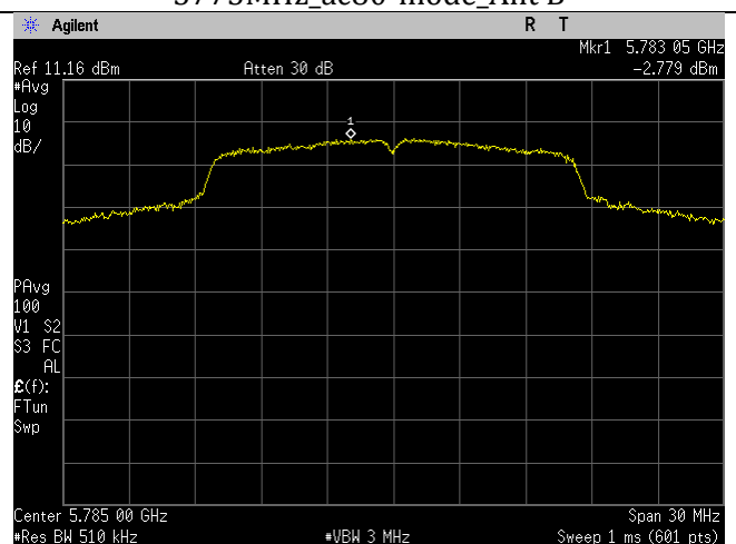
5785MHz_a-mode_Ant B
