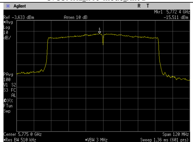
5775MHz_ac80-mode_Ant B
