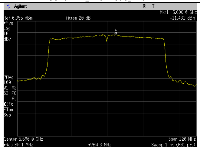
5690MHz_ac80-mode_Ant B
