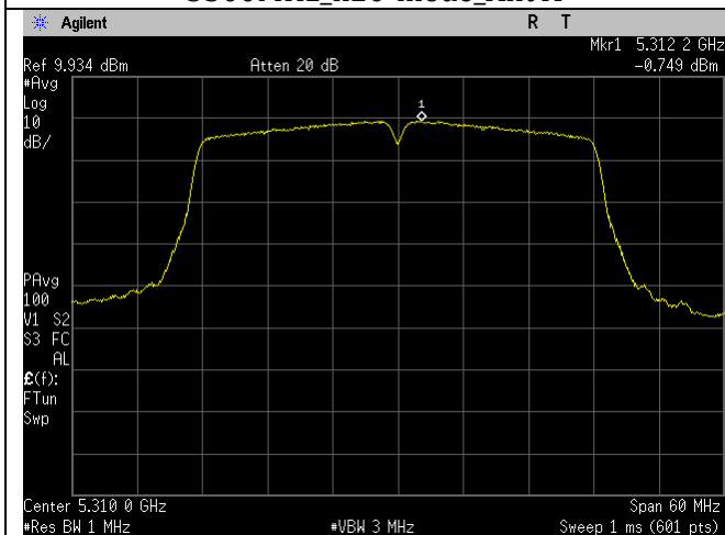
5310MHz_n40-mode_Ant A
