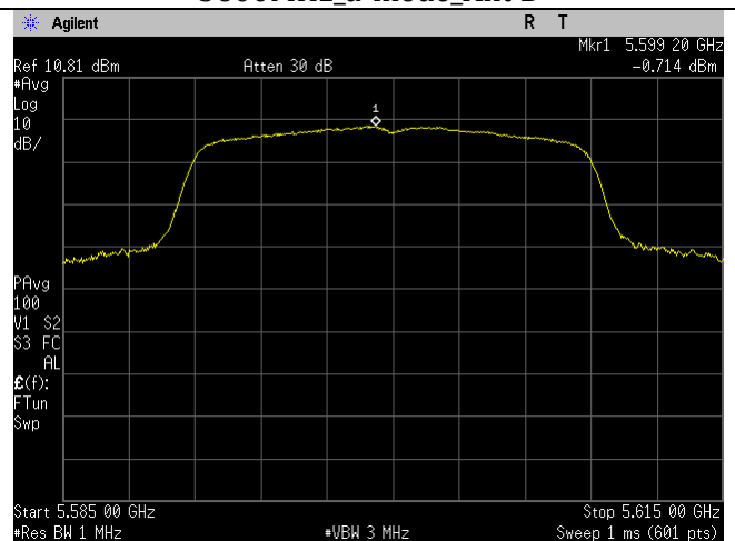
5600MHz_n20-mode_Ant B
