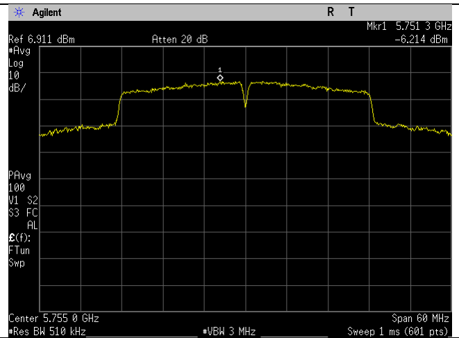
5755MHz_n40-mode_Ant B
