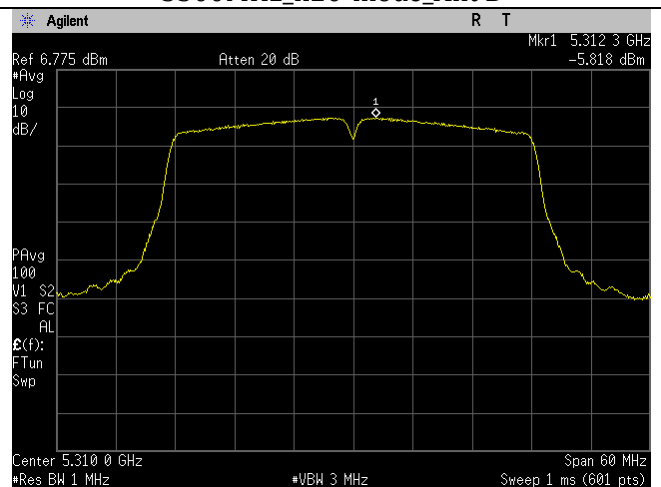
5310MHz_n40-mode_Ant B
