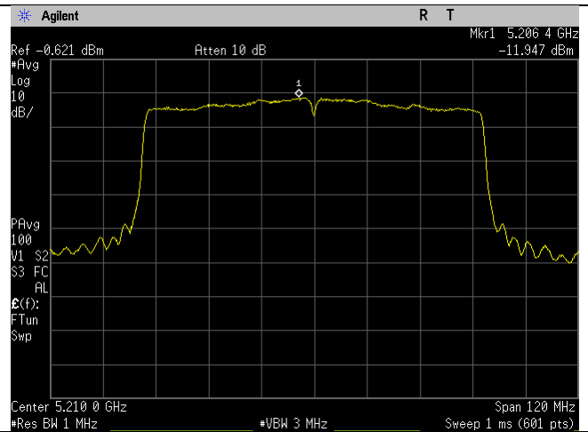
5210MHz_ac80-mode_Ant B
