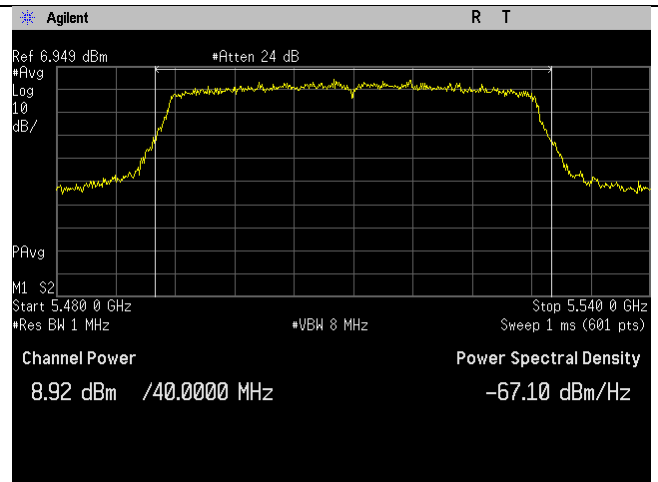
5510MHz_n40-mode_Ant B
