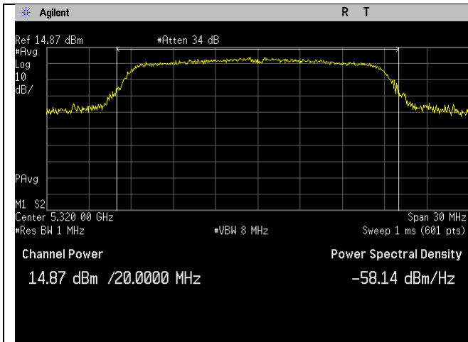
5320MHz_n20-mode_Ant A
