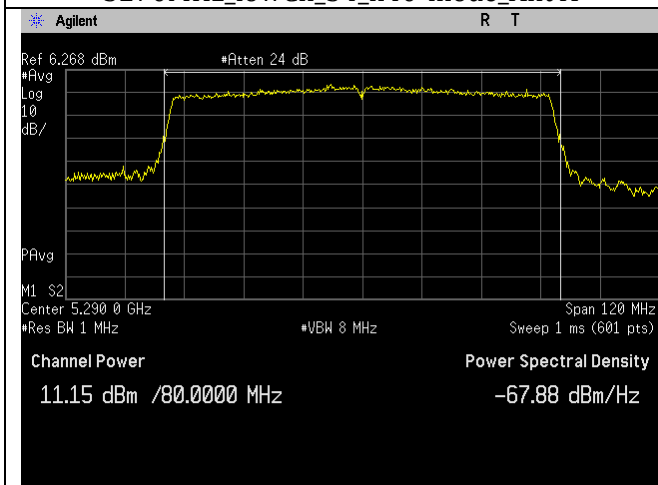
5290MHz_ac80-mode_Ant A
