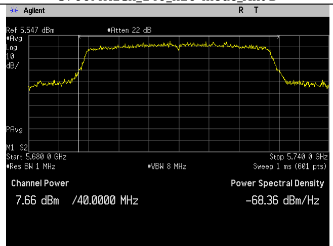
5710MHz_n40-mode_Ant B
