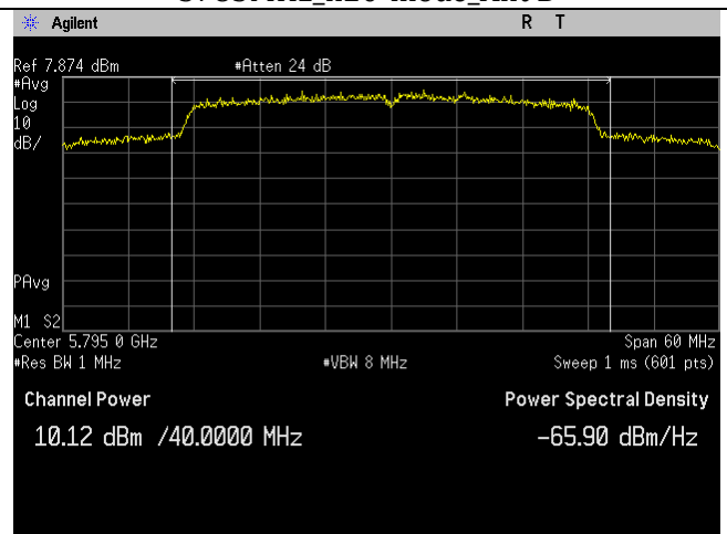
5795MHz_n40-mode_Ant B
