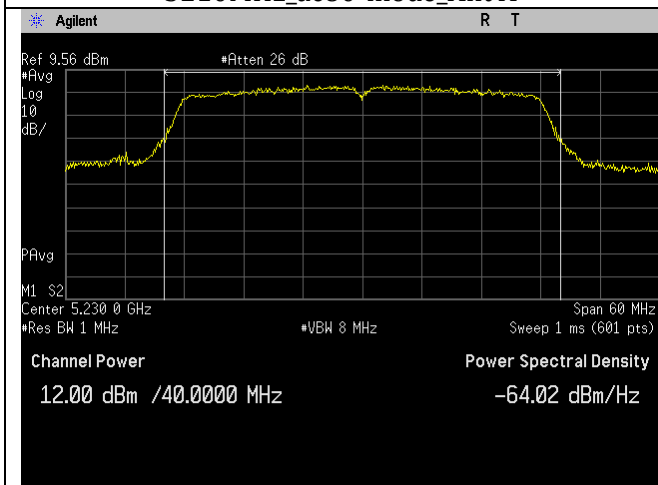
5230MHz_n40-mode_Ant A
