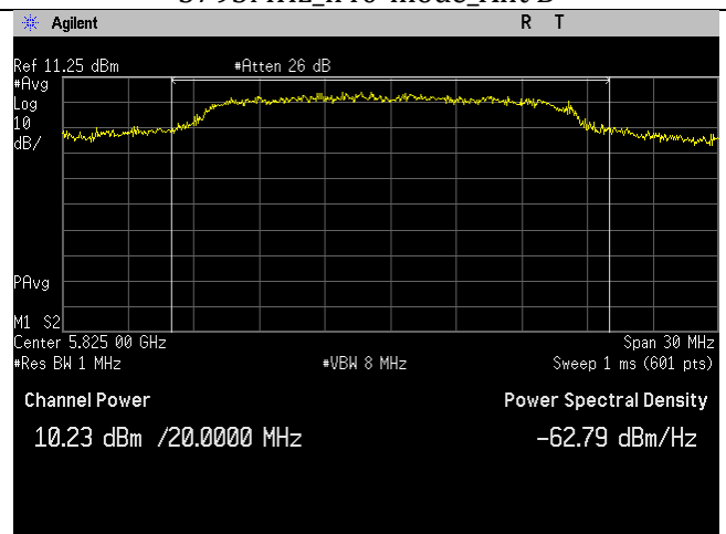
5825MHz_a-mode_Ant B
