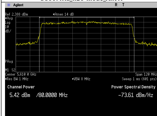
5610MHz_ac80-mode_Ant B
