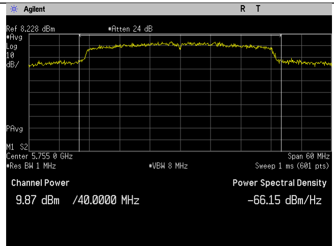
5755MHz_n40-mode_Ant B
