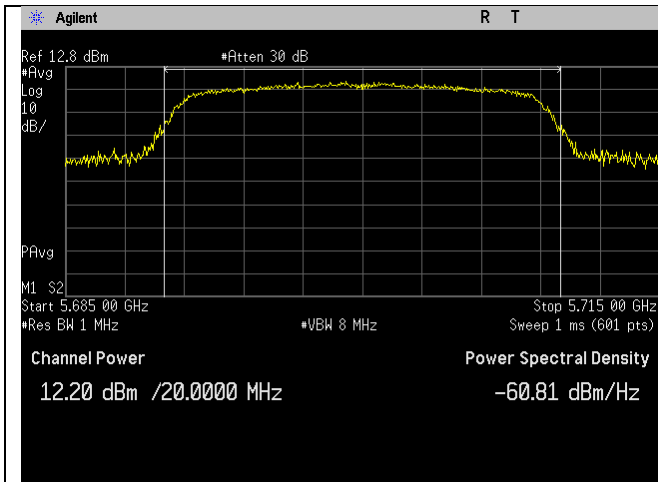
5700MHzCh_140_n20-mode_Ant A
