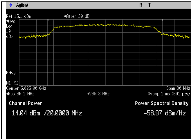
5825MHz_n20-mode_Ant A
