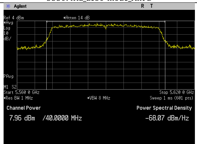
5590MHz_n40-mode_Ant B
