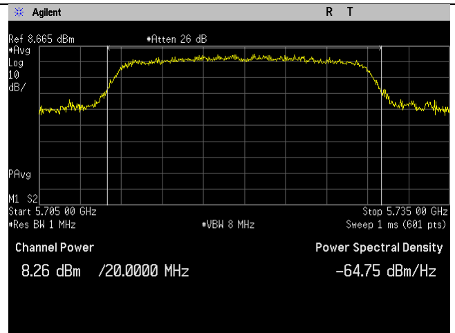
5720MHz_n20-mode_Ant B
