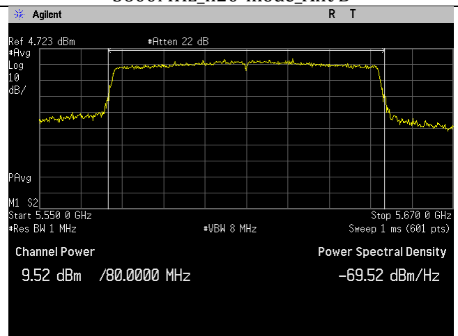
5610MHz_ac80-mode_Ant A
