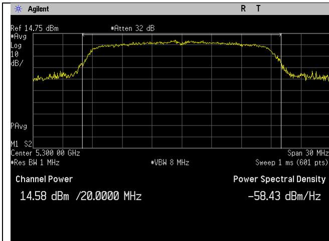
5300MHz_n20-mode_Ant A
