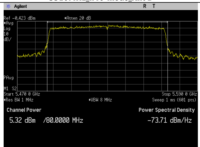
5530MHz_ac80-mode_Ant B
