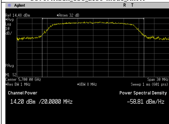
5700MHzCh_140_a-mode_Ant A
