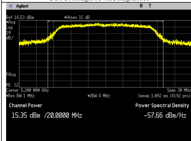
5200MHz_low_a-mode_Ant A
