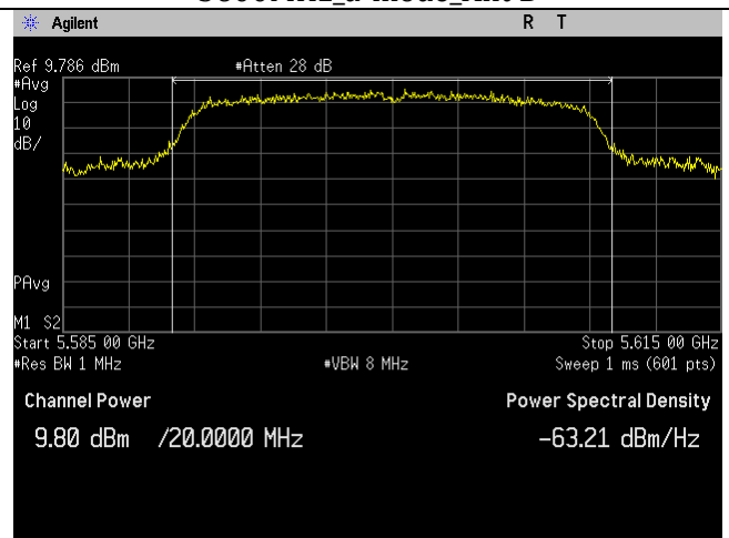
5600MHz_n20-mode_Ant B
