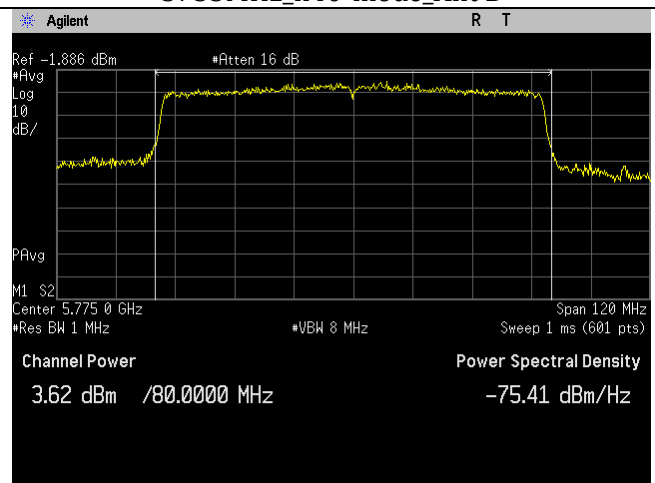
5775MHz_ac80-mode_Ant B
