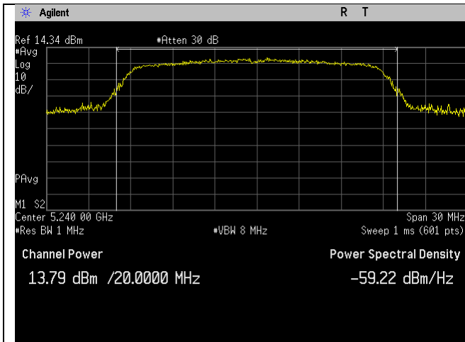
5240MHz_n20-mode_Ant A
