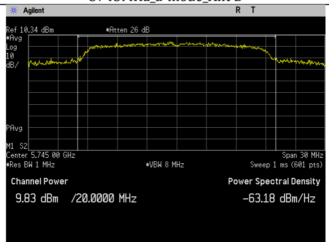
5745MHz_n20-mode_Ant B
