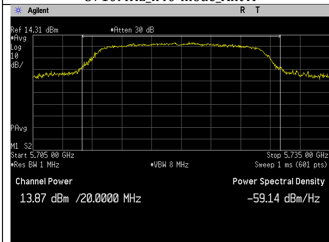
5720MHz_a-mode_Ant A
