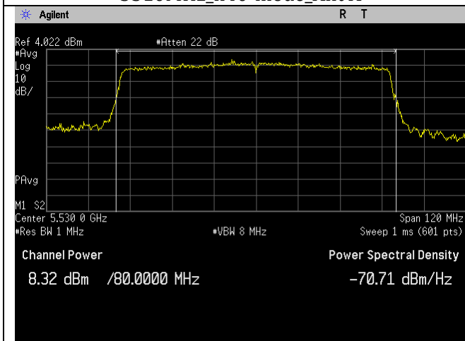
5530MHz_ac80-mode_Ant A
