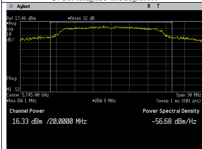
5745MHz_a-mode_Ant A
