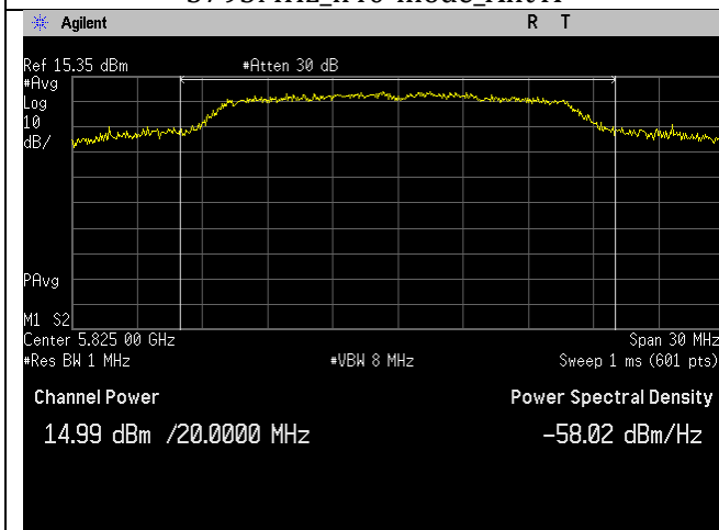
5825MHz_a-mode_Ant A
