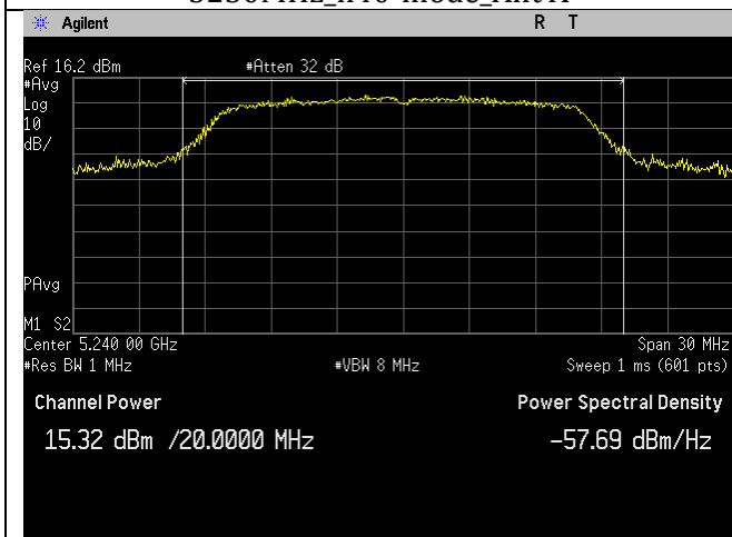
5240MHz_a-mode_Ant A
