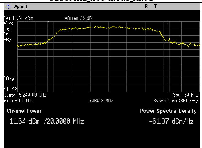
5240MHz_a-mode_Ant B
