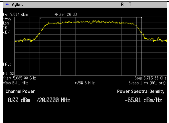
5700MHzCh_140_n20-mode_Ant B
