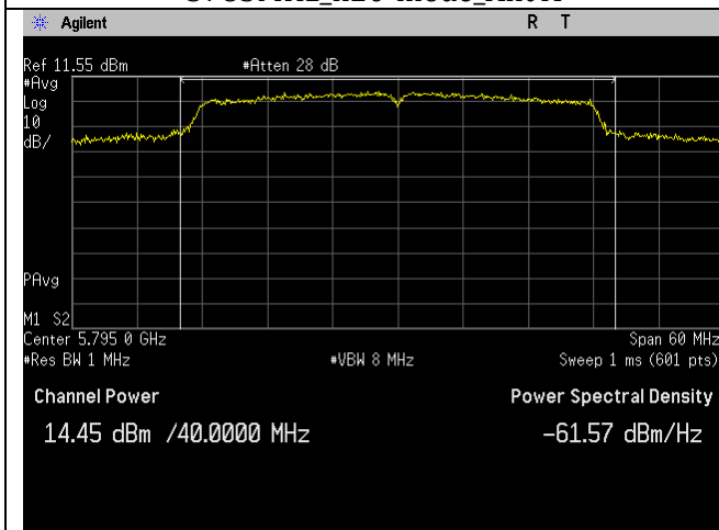
5795MHz_n40-mode_Ant A
