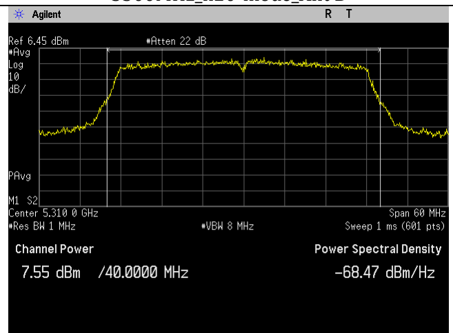
5310MHz_n40-mode_Ant B
