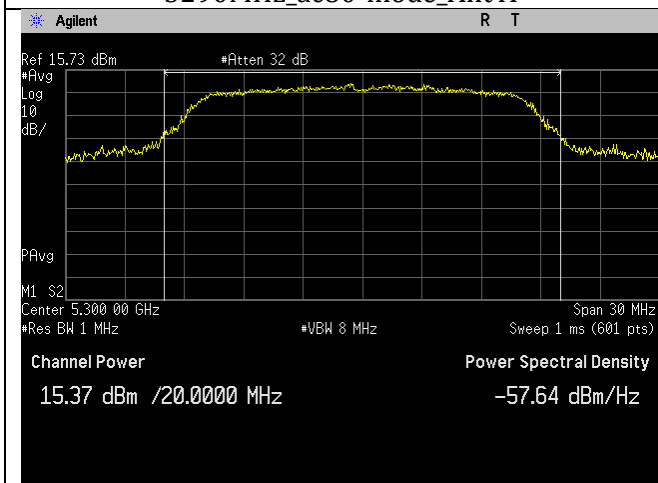
5300MHz_a-mode_Ant A
