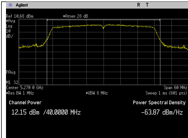
5270MHz_lowCh_54_n40-mode_Ant A
