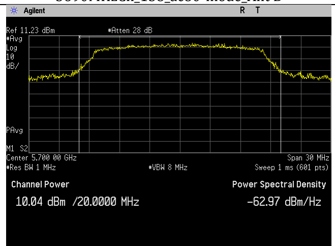
5700MHzCh_140_a-mode_Ant B
