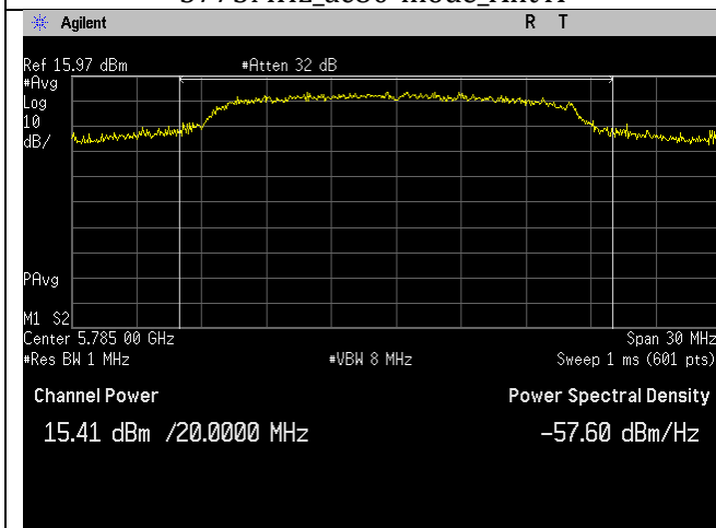
5785MHz_a-mode_Ant A
