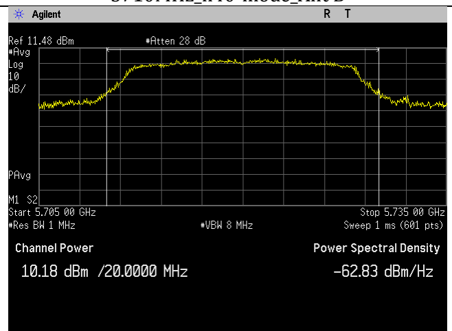
5720MHz_a-mode_Ant B
