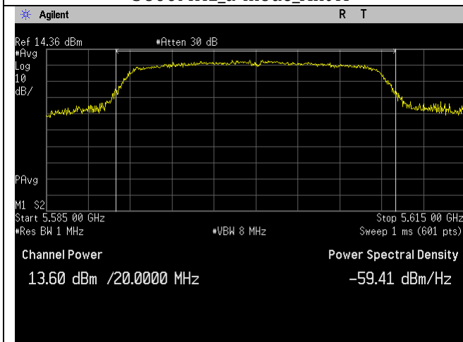
5600MHz_n20-mode_Ant A
