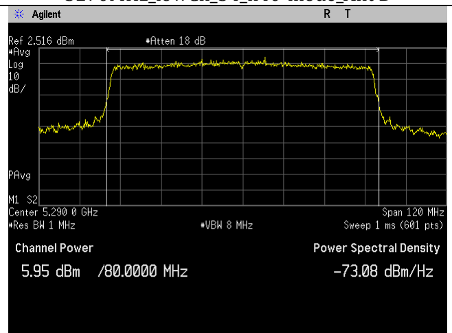
5290MHz_ac80-mode_Ant B
