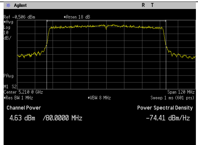
5210MHz_ac80-mode_Ant B
