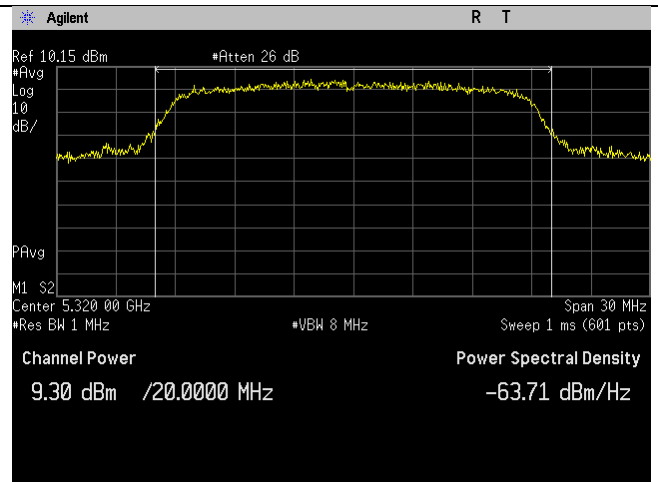
5320MHz_n20-mode_Ant B
