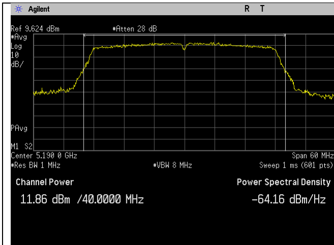
5190MHz_n40-mode_Ant A
