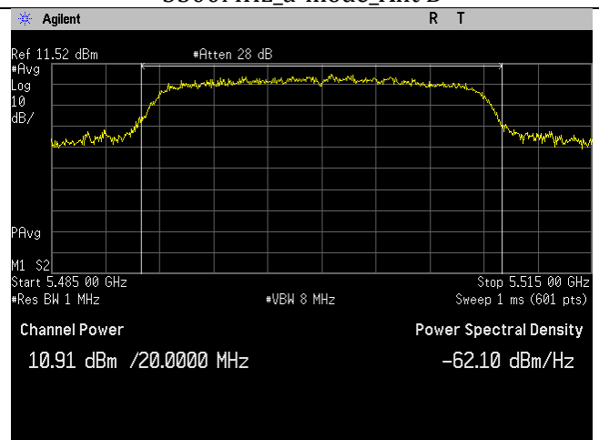
5500MHz_n20-mode_Ant B
