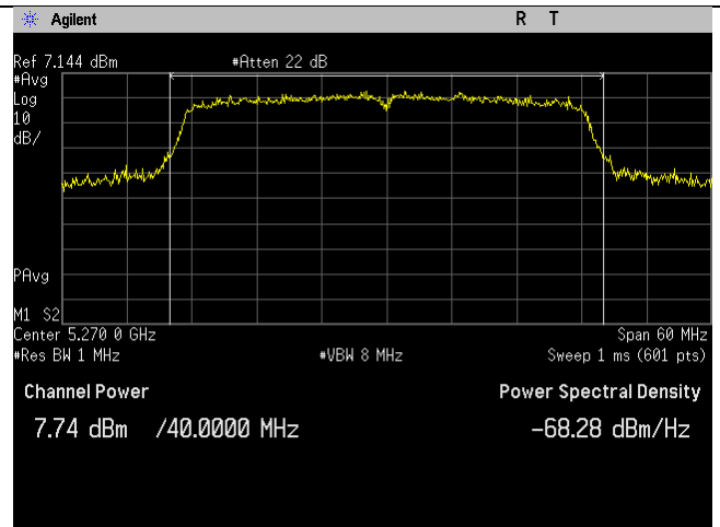
5270MHz_lowCh_54_n40-mode_Ant B
