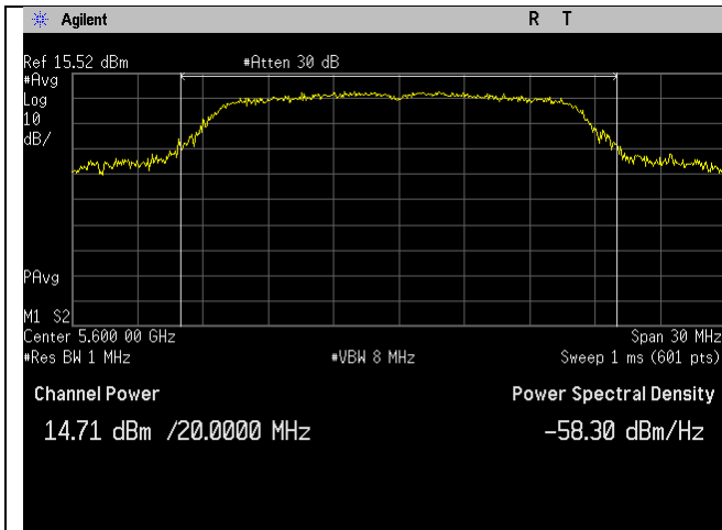
5600MHz_a-mode_Ant A
