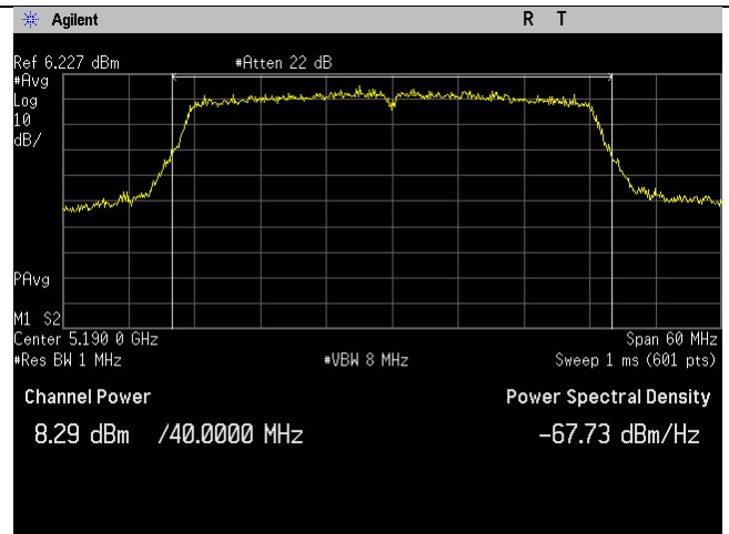
5190MHz_n40-mode_Ant B
