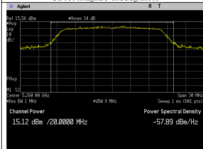
5260MHz_low_a-mode_Ant A
