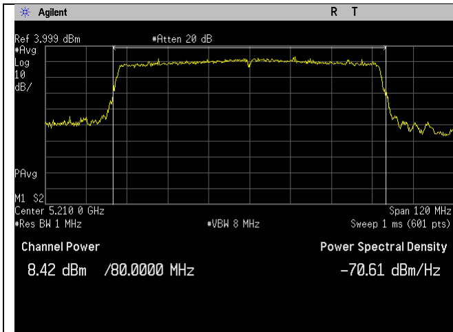
5210MHz_ac80-mode_Ant A
