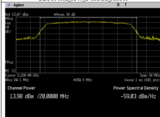
5260MHz_low_n20-mode_Ant A
