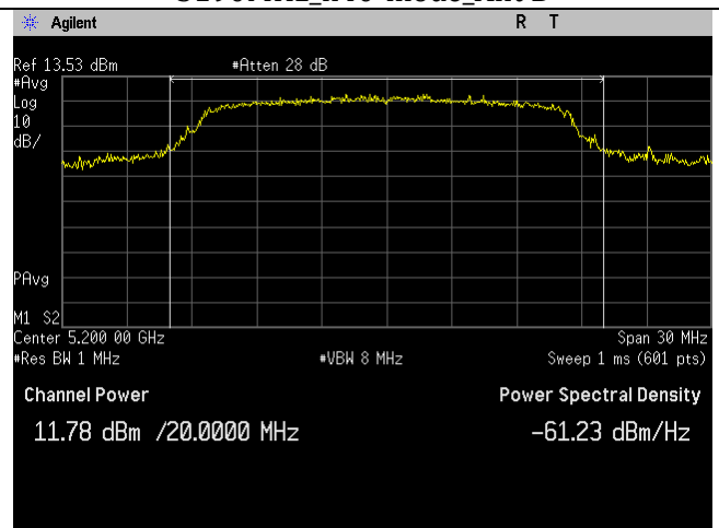
5200MHz_low_a-mode_Ant B
