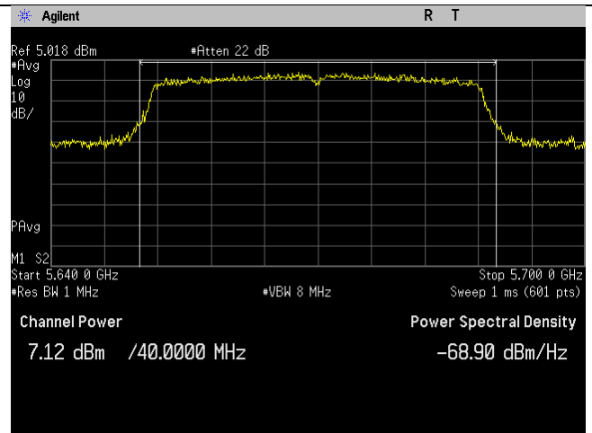
5670MHz_n40-mode_Ant B
