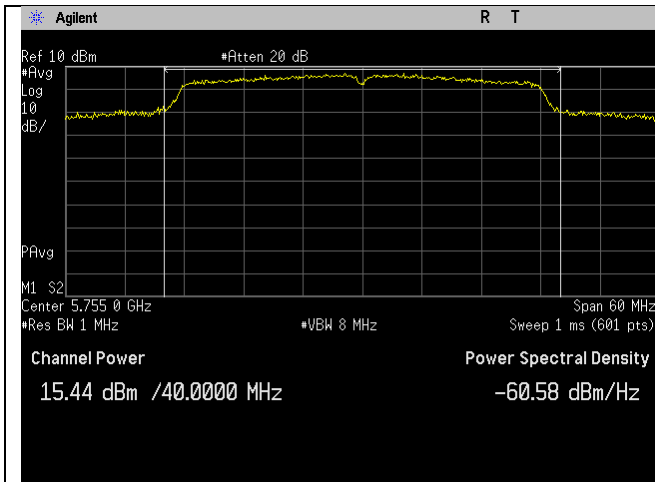
5755MHz_n40-mode_Ant A
