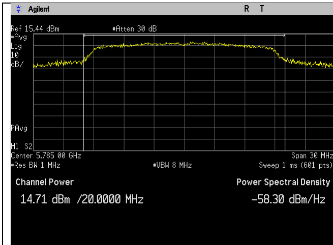
5785MHz_n20-mode_Ant A
