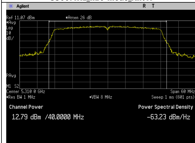
5310MHz_n40-mode_Ant A
