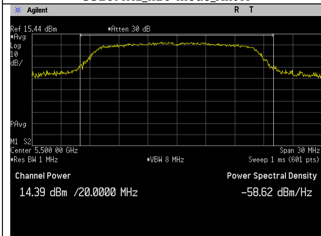
5500MHz_a-mode_Ant A
