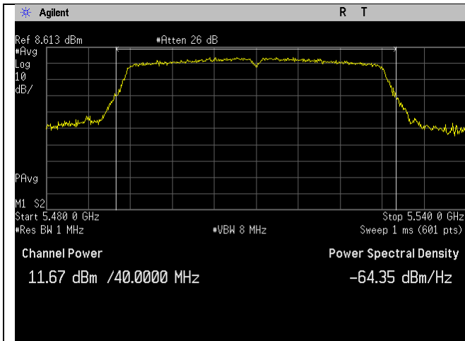
5510MHz_n40-mode_Ant A
