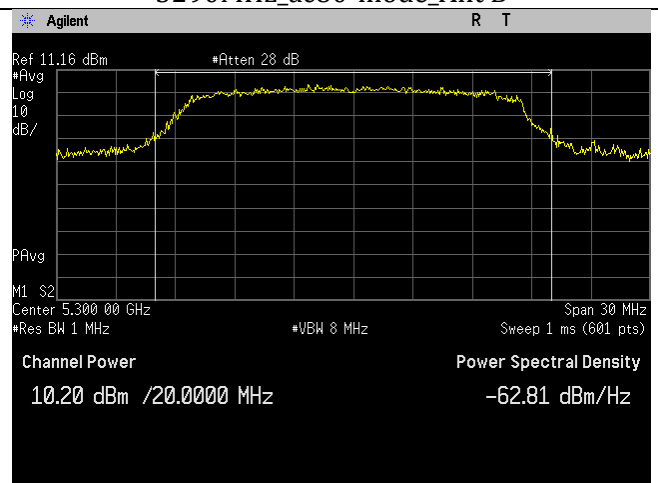
5300MHz_a-mode_Ant B
