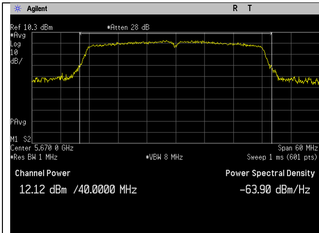
5670MHz_n40-mode_Ant A
