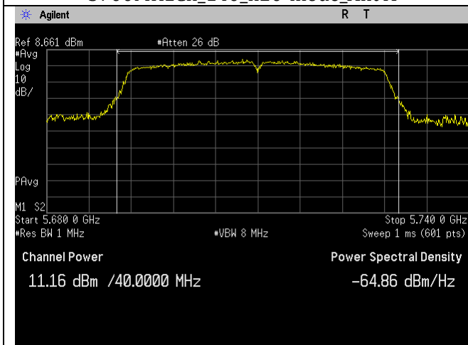
5710MHz_n40-mode_Ant A
