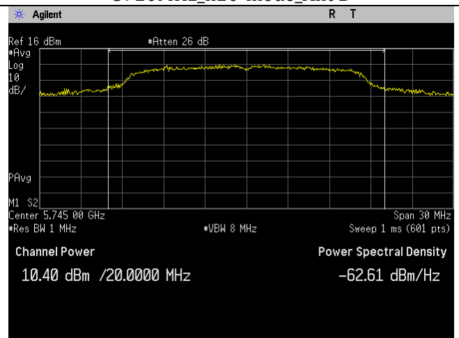
5745MHz_a-mode_Ant B
