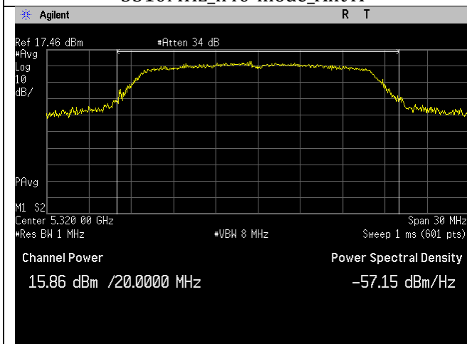
5320MHz_a-mode_Ant A
