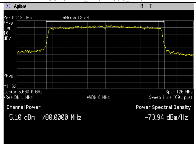
5690MHzCh_138_ac80-mode_Ant B
