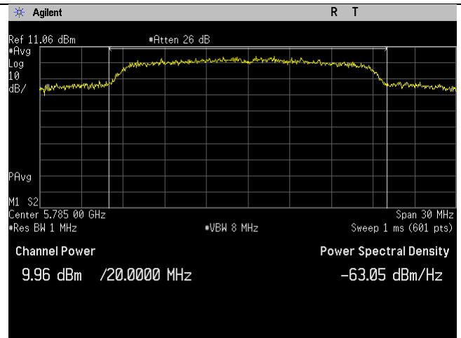
5785MHz_n20-mode_Ant B
