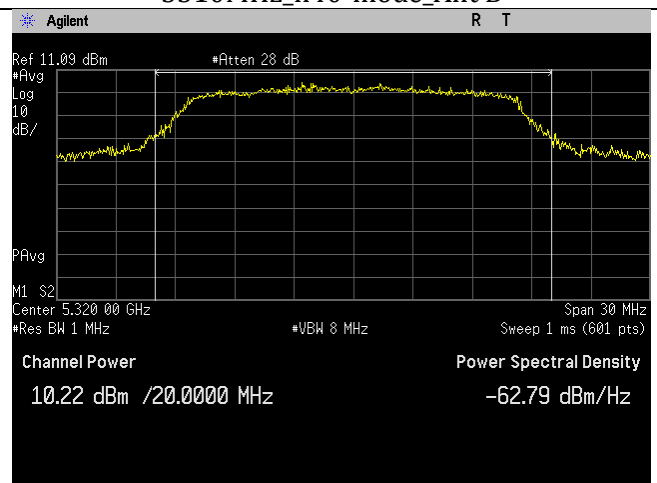
5320MHz_a-mode_Ant B
