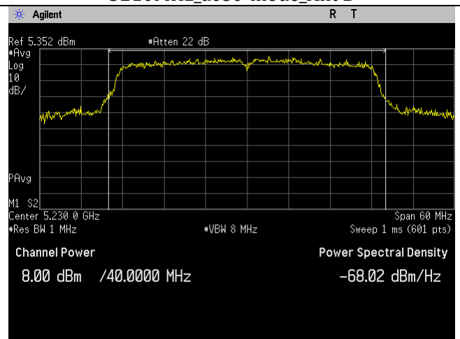
5230MHz_n40-mode_Ant B
