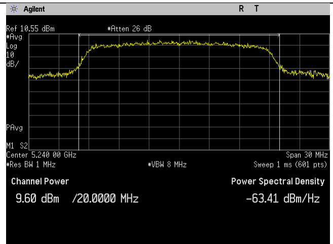
5240MHz_n20-mode_Ant B
