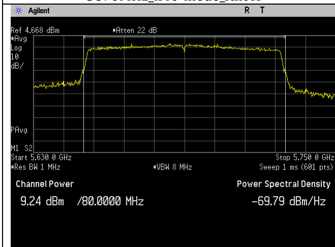
5690MHzCh_138_ac80-mode_Ant A
