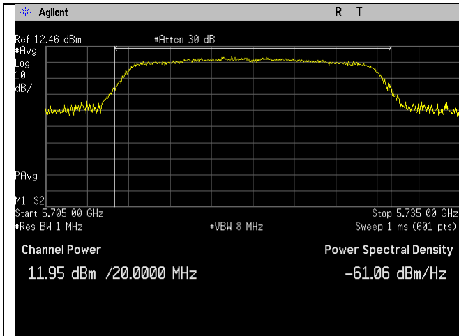
5720MHz_n20-mode_Ant A
