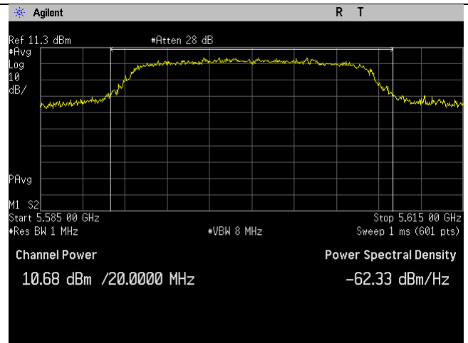
5600MHz_a-mode_Ant B
