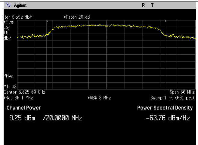
5825MHz_n20-mode_Ant B
