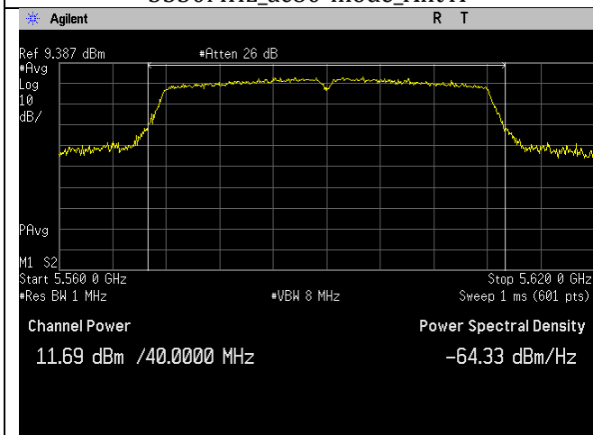
5590MHz_n40-mode_Ant A
