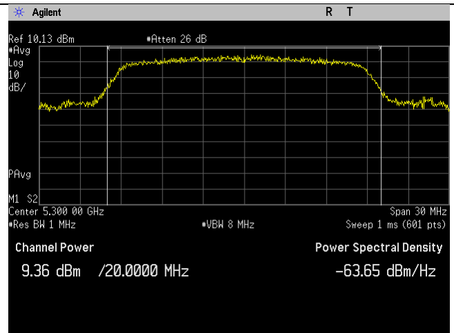
5300MHz_n20-mode_Ant B
