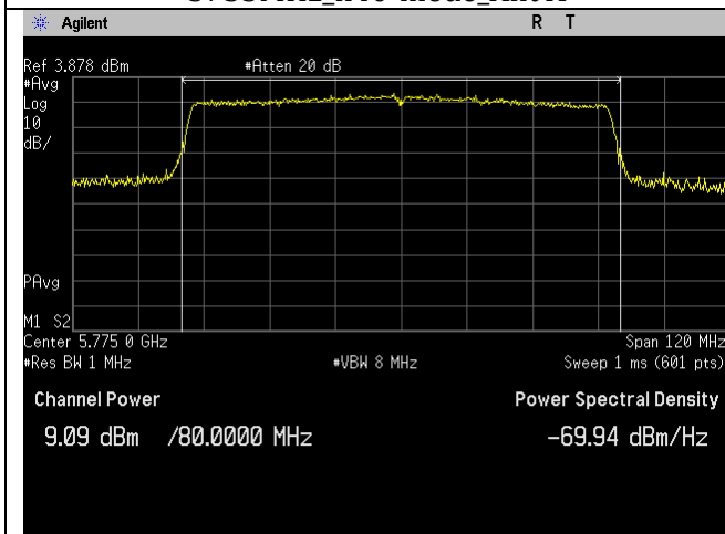
5775MHz_ac80-mode_Ant A
