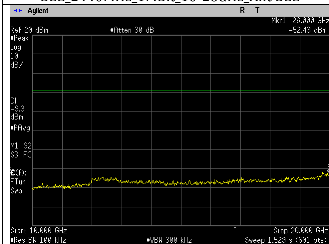
BLE_2440MHz_2MBit_10-26GHz_Ant BLE
