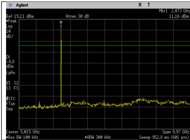
BLE_2480MHz_2MBit_30MHz-10GHz_Ant BLE
