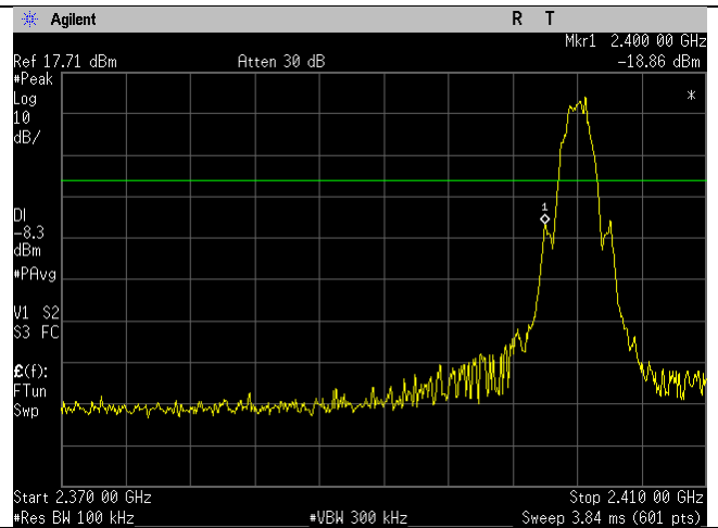
BLE_2402MHz_2MBit_Lower Band Edge_Ant BLE
