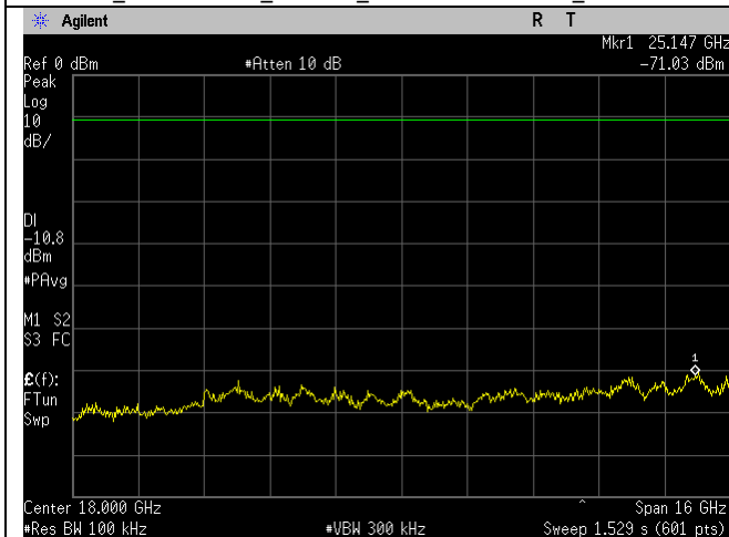
BLE_2440MHz_1MBit_10-26GHz_Ant BLE
