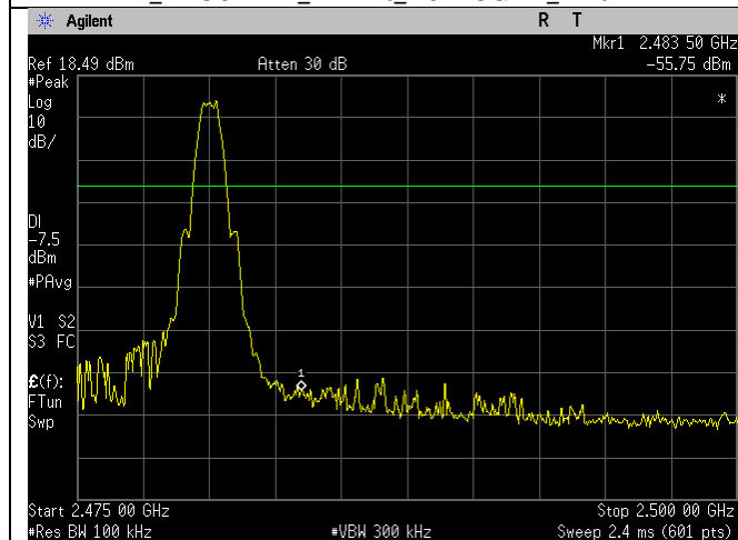
BLE_2480MHz_1MBit_Upper Band Edge_Ant BLE
