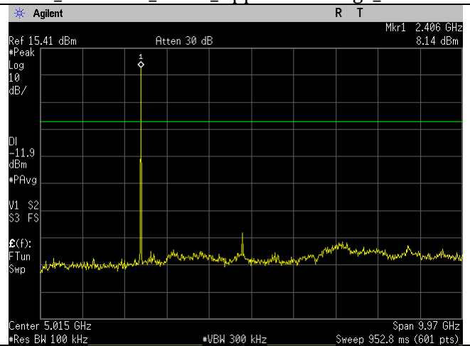
BLE_2402MHz_1MBit_30MHz-10GHz_Ant BLE
