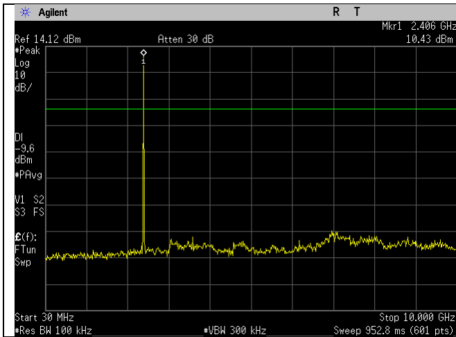
BLE_2402MHz_2MBit_30MHz-10GHz_Ant BLE
