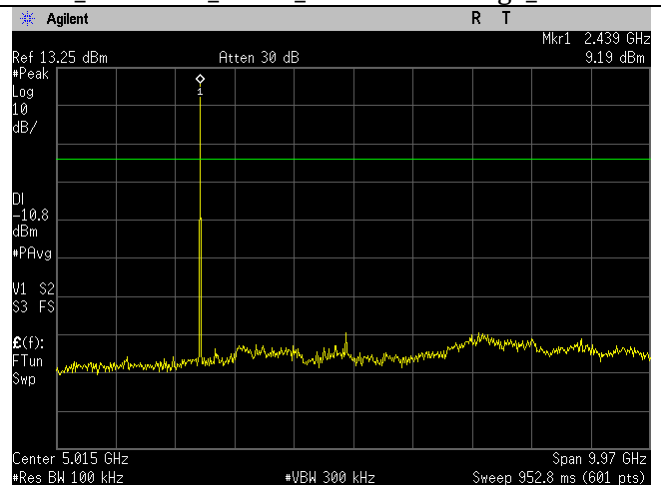
BLE_2440MHz_1MBit_30MHz-10GHz_Ant BLE
