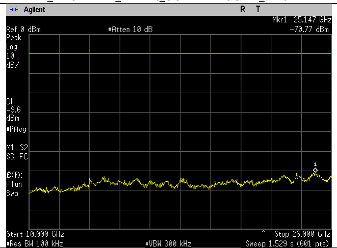
BLE_2402MHz_2MBit_10-26GHz_Ant BLE
