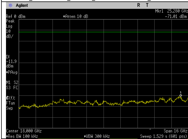
BLE_2402MHz_1MBit_10-26GHz_Ant BLE
