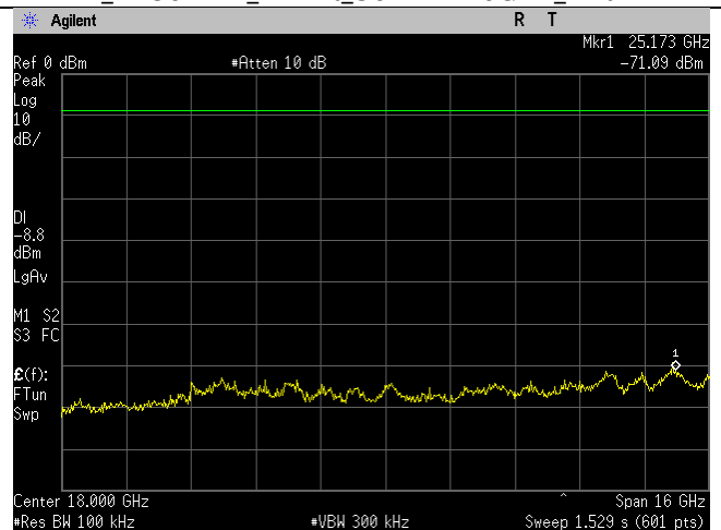
BLE_2480MHz_2MBit_10-26GHz_Ant BLE
