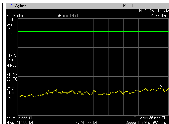
BLE_2480MHz_1MBit_10-26GHz_Ant BLE
