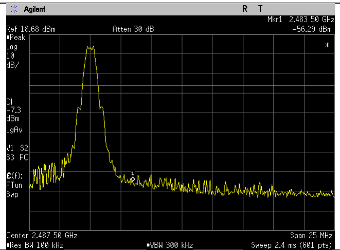
BLE_2480MHz_2MBit_Upper Band Edge_Ant BLE
