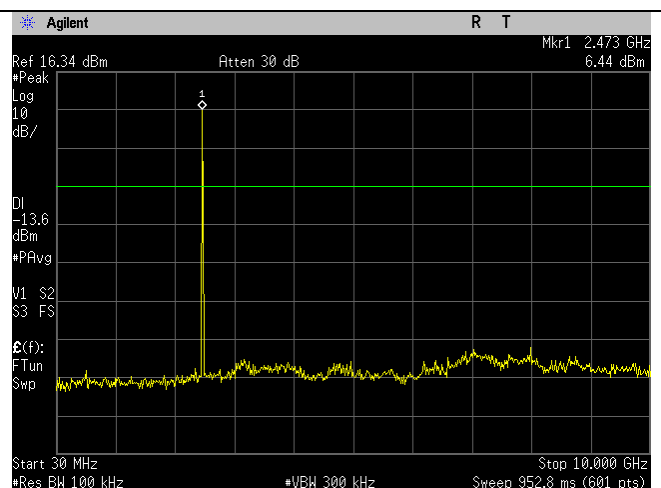
BLE_2480MHz_1MBit_30MHz-10GHz_Ant BLE
