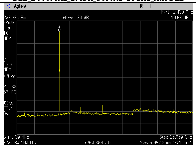
BLE_2440MHz_2MBit_30MHz-10GHz_Ant BLE
