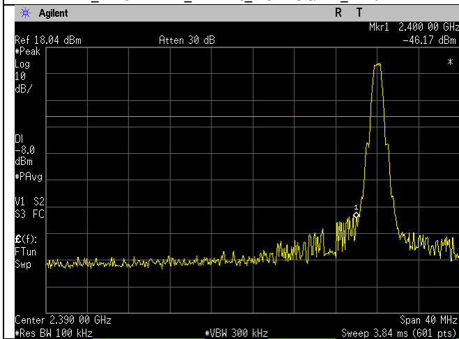
BLE_2402MHz_1MBit_Lower Band Edge_Ant BLE
