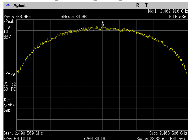
BLE_2402MHz_2MBit_Ant BLE
