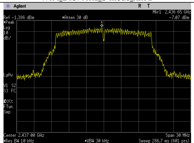
WIFI_2437MHz_g-mode_Ant B
