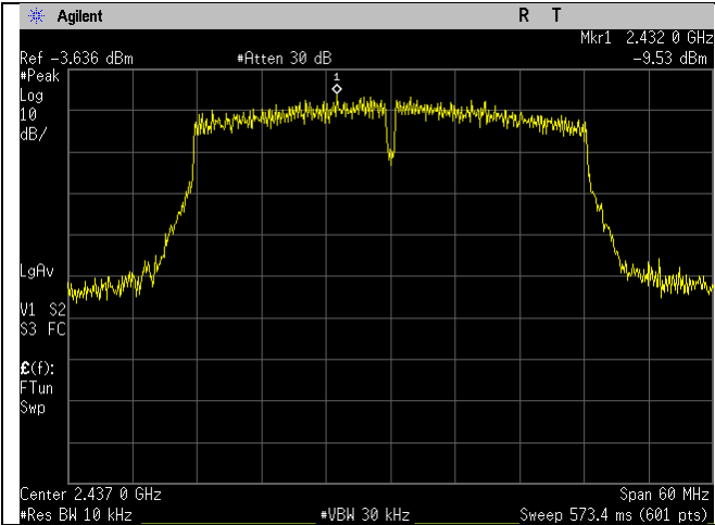
WIFI_2437MHz_n40-mode_Ant A
