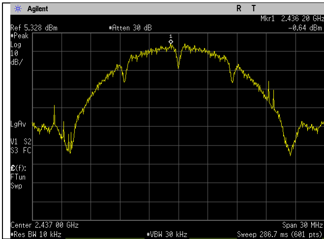
WIFI_2437MHz_b-mode_Ant A
