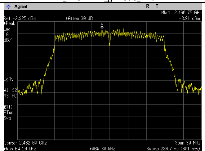
WIFI_2462MHz_n20-mode_Ant B
