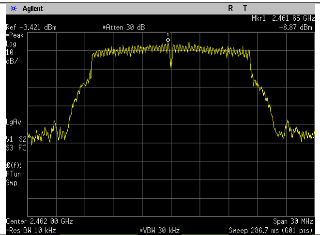
WIFI_2462MHz_g-mode_Ant B
