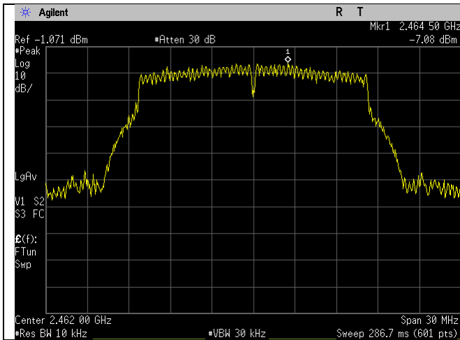
WIFI_2462MHz_g-mode_Ant A
