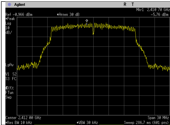
WIFI_2412MHz_g-mode_Ant A
