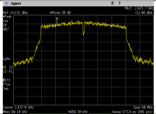
WIFI_2437MHz_n40-mode_Ant B
