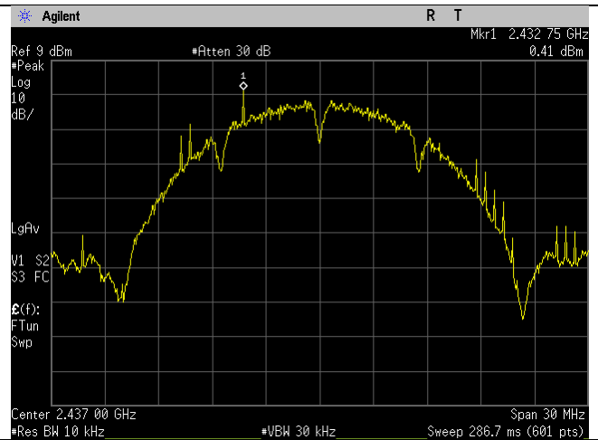
WIFI_2437MHz_b-mode_Ant B
