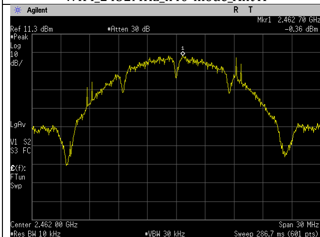
WIFI_2462MHz_b-mode_Ant A
