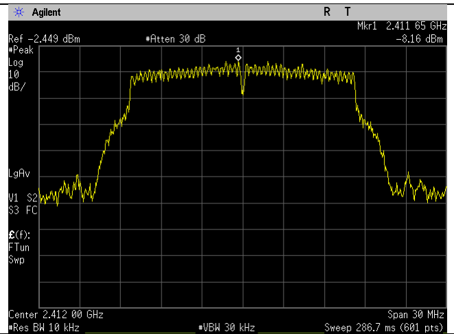
WIFI_2412MHz_g-mode_Ant B
