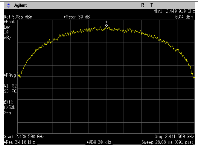
BLE_2440MHz_2MBit_Ant BLE
