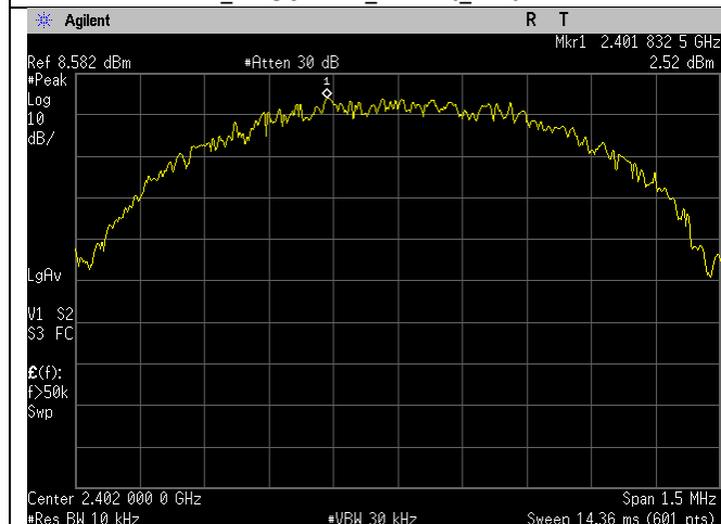
BLE_2402MHz_1MBit_Ant BLE
