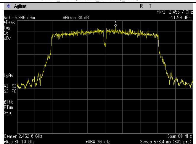
WIFI_2452MHz_n40-mode_Ant B
