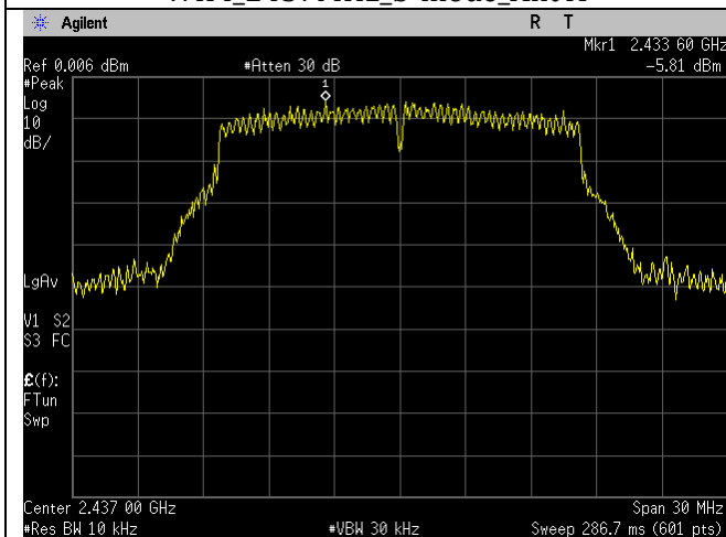
WIFI_2437MHz_g-mode_Ant A
