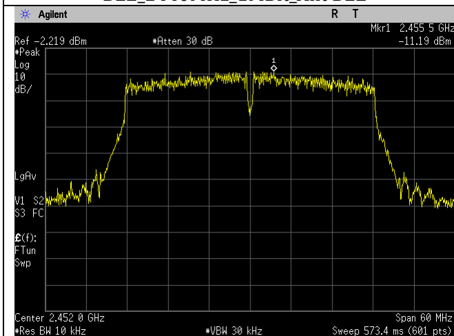
WIFI_2452MHz_n40-mode_Ant A
