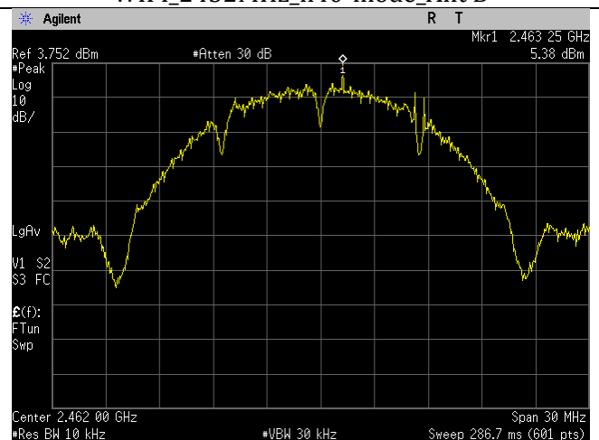
WIFI_2462MHz_b-mode_Ant B
