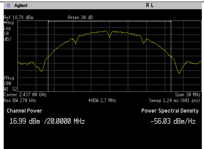
WIFI_2437MHz_b-mode_Ant B
