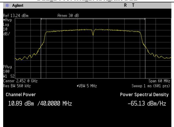
WIFI_2452MHz_n40-mode_Ant B
