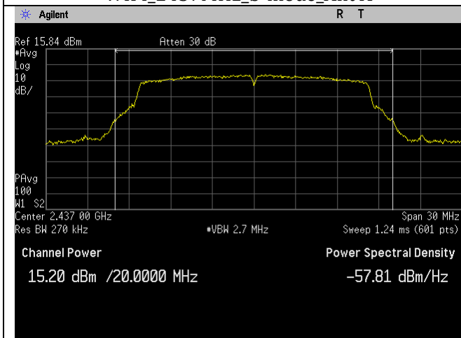
WIFI_2437MHz_g-mode_Ant A
