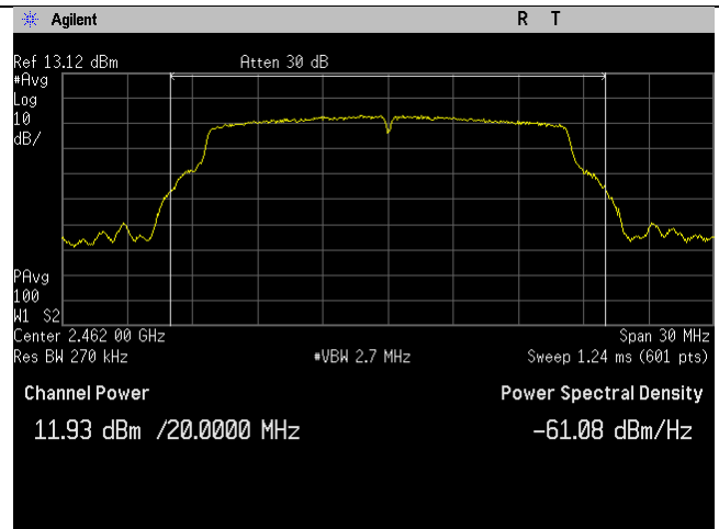
WIFI_2462MHz_g-mode_Ant B
