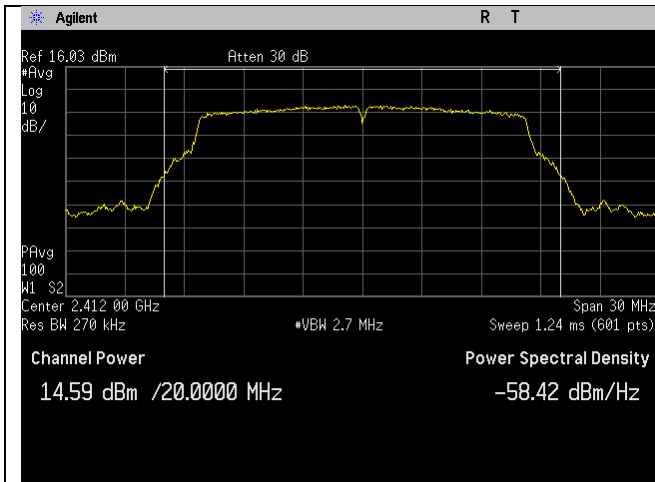
WIFI_2412MHz_g-mode_Ant A
