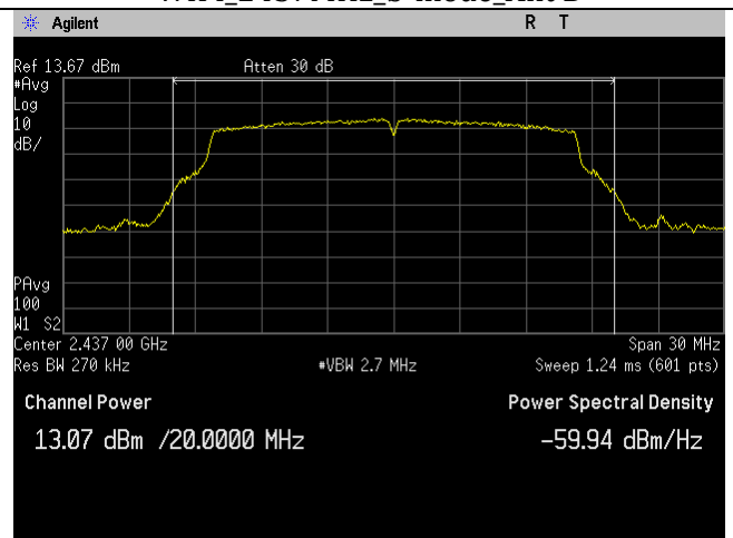
WIFI_2437MHz_g-mode_Ant B
