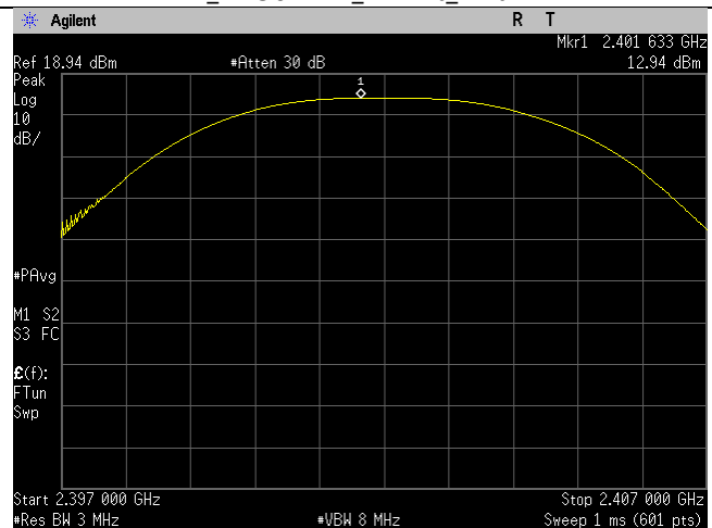
BLE_2402MHz_2MBit_Ant BLE
