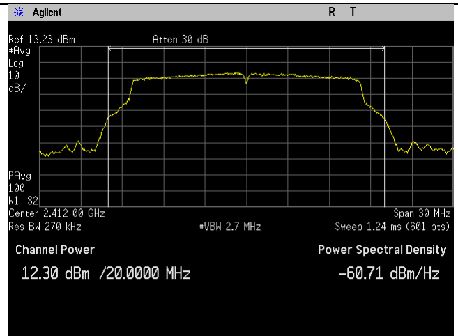
WIFI_2412MHz_g-mode_Ant B
