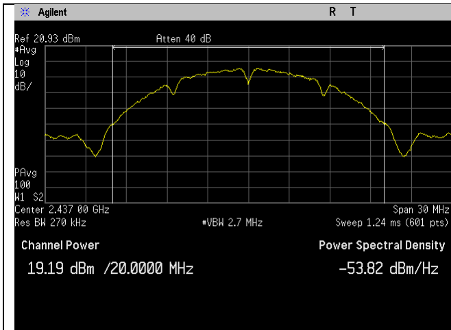
WIFI_2437MHz_b-mode_Ant A
