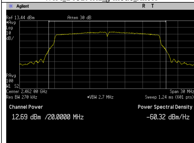
WIFI_2462MHz_n20-mode_Ant A
