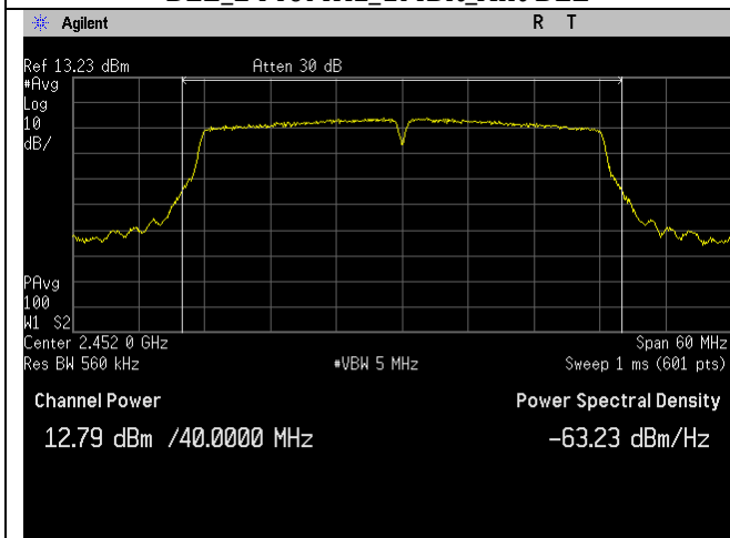
WIFI_2452MHz_n40-mode_Ant A
