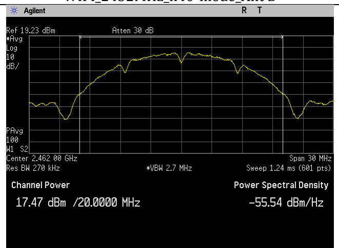
WIFI_2462MHz_b-mode_Ant B
