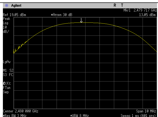
BLE_2480MHz_2MBit_Ant BLE
