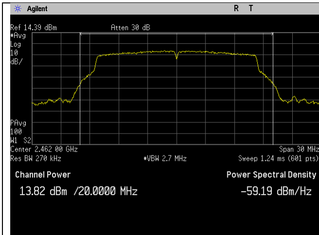
WIFI_2462MHz_g-mode_Ant A
