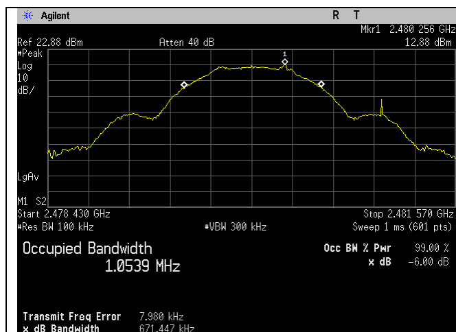
BLE_2480MHz_1MBit_-6dB_Ant BLE
