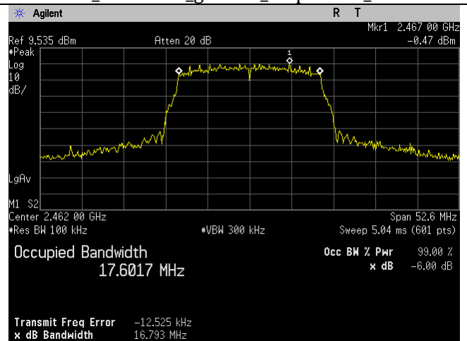
WIFI_2462MHz_n20-mode_-6dB_Ant B
