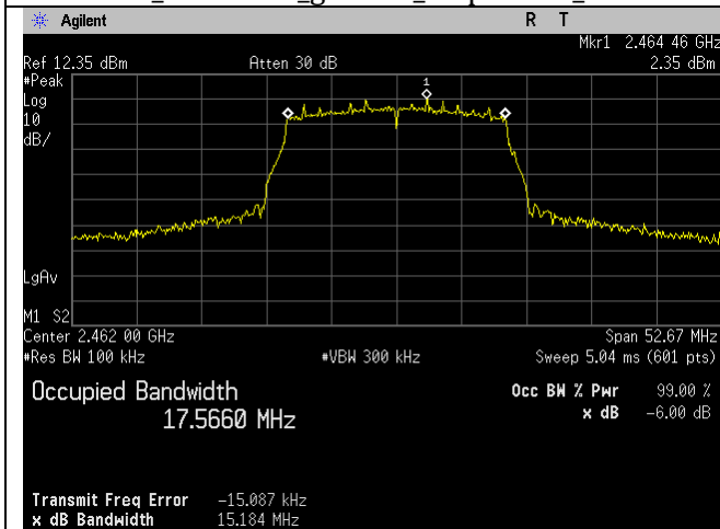
WIFI_2462MHz_n20-mode_-6dB_Ant A
