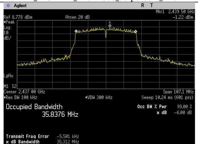
WIFI_2437MHz_n40-mode_-6dB_Ant B
