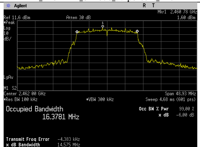
WIFI_2462MHz_g-mode_-6dB_Ant B
