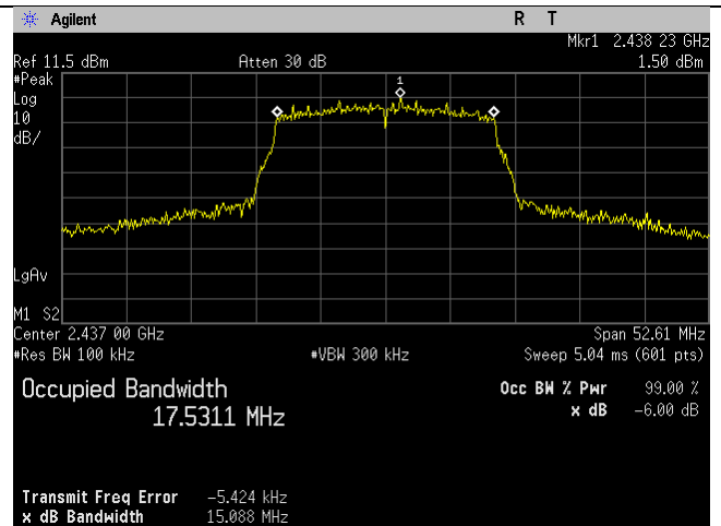
WIFI_2437MHz_n20-mode_-6dB_Ant B
