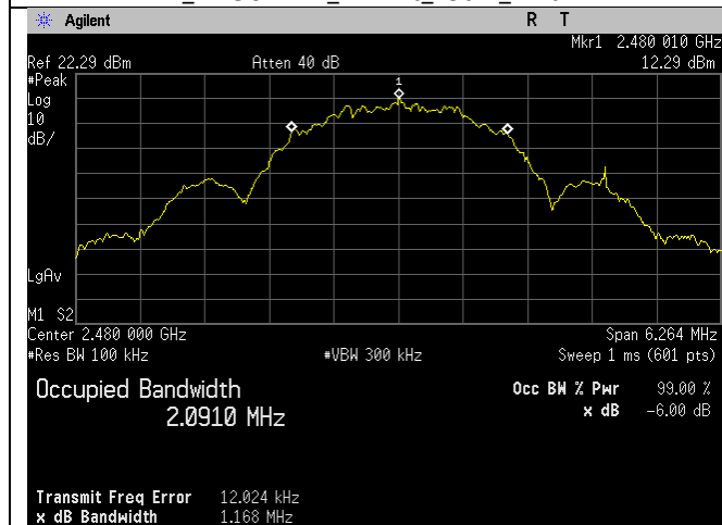
BLE_2480MHz_2MBit_-6dB_Ant BLE
