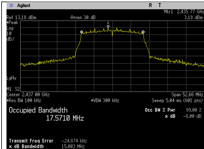
WIFI_2437MHz_n20-mode_-6dB_Ant A
