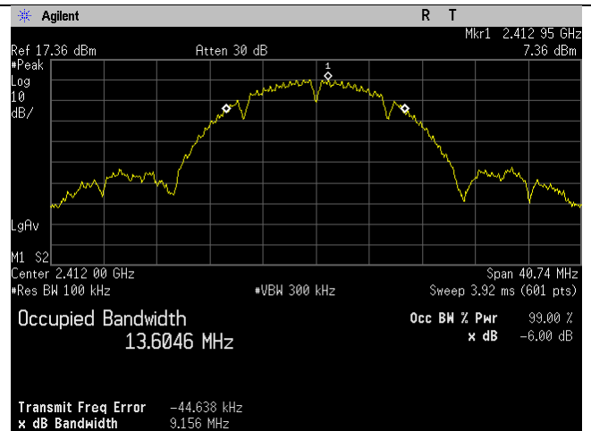
WIFI_2412MHz_b-mode_-6dB_Ant B
