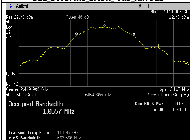
BLE_2440MHz_1MBit_-6dB_Ant BLE
