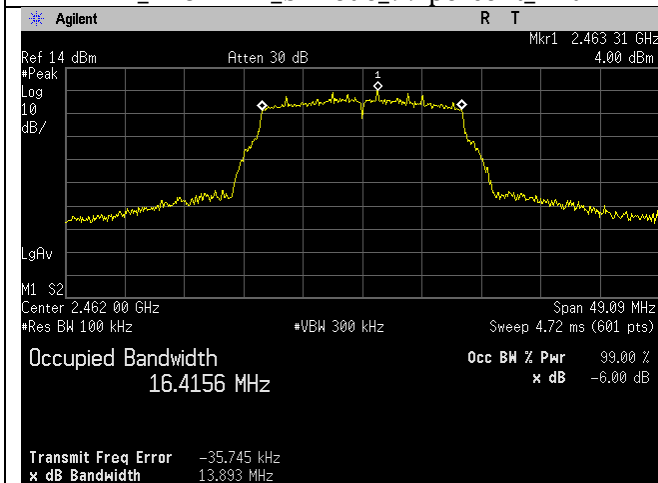
WIFI_2462MHz_g-mode_-6dB_Ant A
