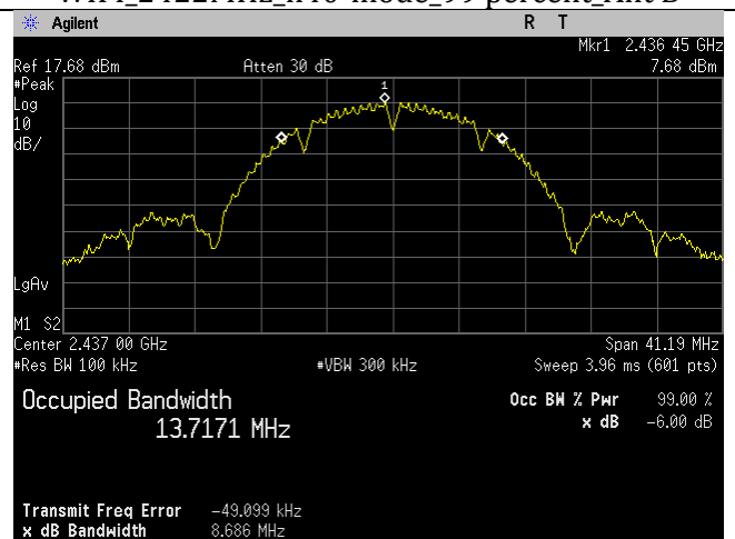
WIFI_2437MHz_b-mode_-6dB_Ant B
