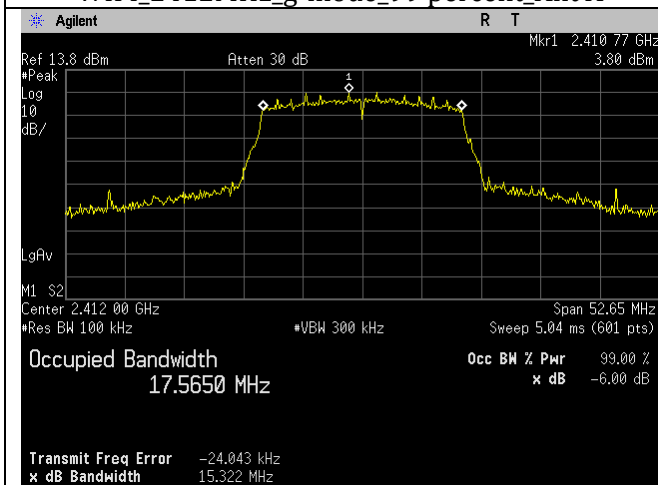
WIFI_2412MHz_n20-mode_-6dB_Ant A
