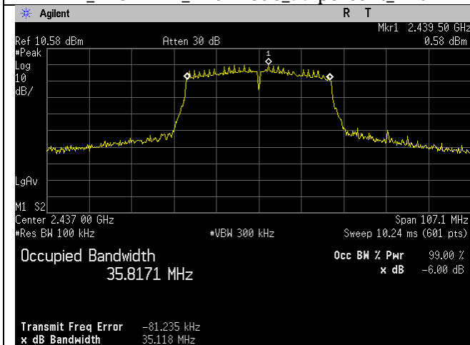
WIFI_2437MHz_n40-mode_-6dB_Ant A
