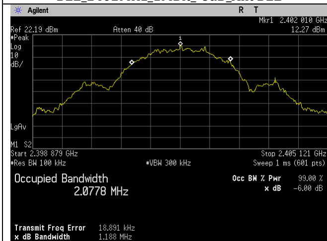
BLE_2402MHz_2MBit_-6dB_Ant BLE
