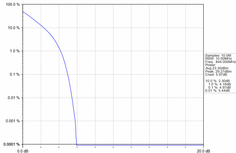
B26_10MHz_QPSK_HCH_844MHz_RB_50_0_NTNV
