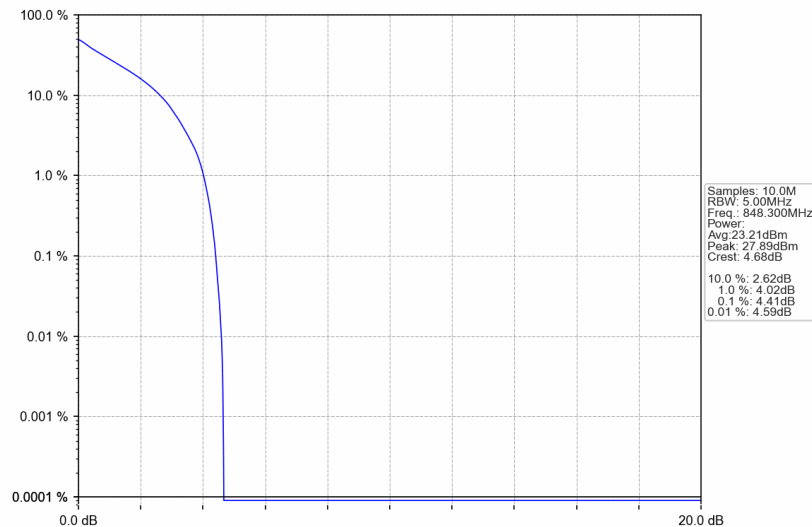
B26_1.4MHz_QPSK_HCH_848.3MHz_RB_6_0_NTNV
