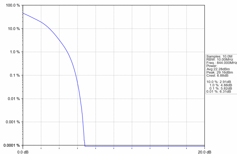
B26_10MHz_16QAM_HCH_844MHz_RB_50_0_NTNV
