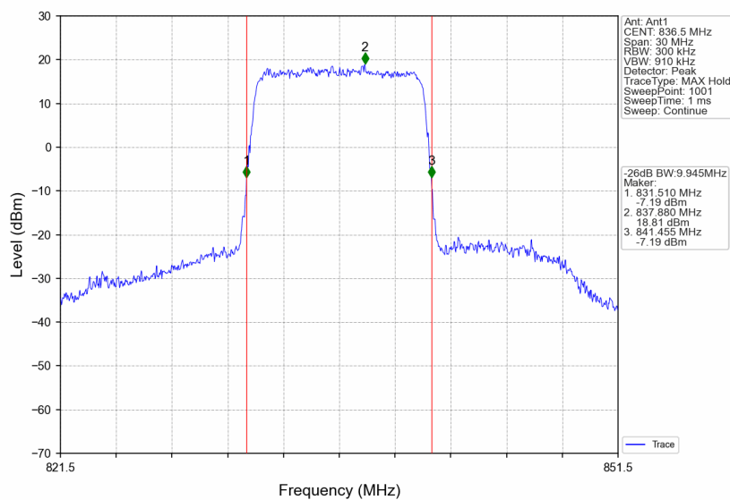
B26_10MHz_16QAM_MCH_836.5MHz_RB_50_0_NTNV
