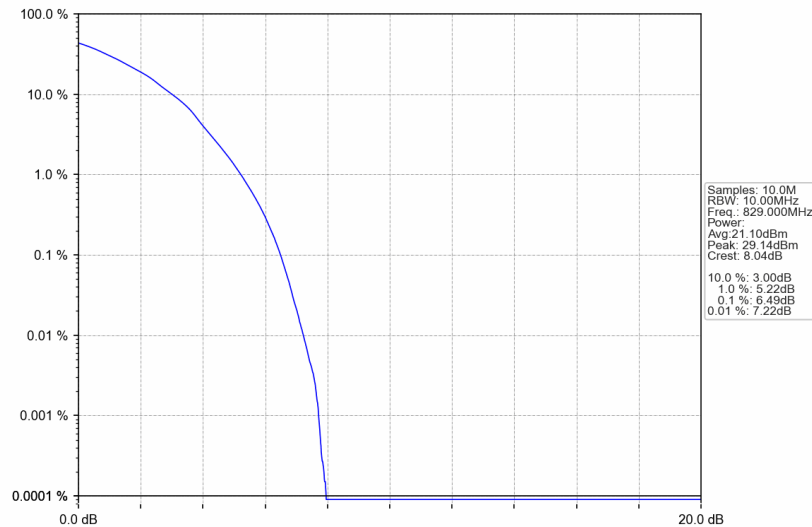
B26_10MHz_64QAM_LCH_829MHz_RB_50_0_NTNV
