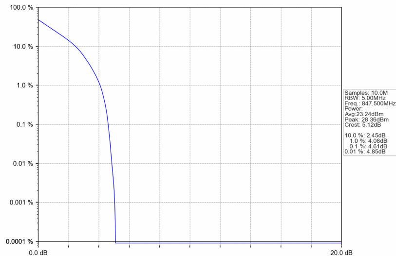
B26_3MHz_QPSK_HCH_847.5MHz_RB_15_0_NTNV
