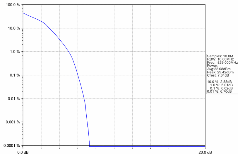
B26_10MHz_16QAM_LCH_829MHz_RB_50_0_NTNV
