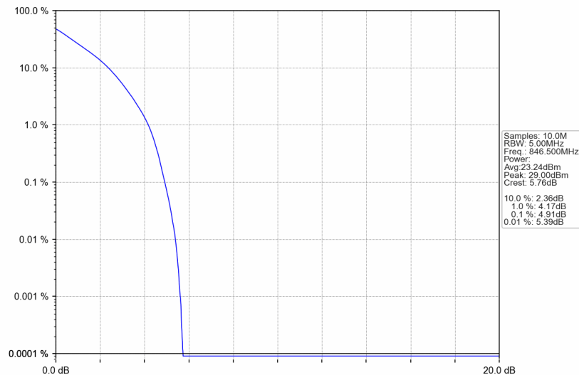
B26_5MHz_QPSK_HCH_846.5MHz_RB_25_0_NTNV
