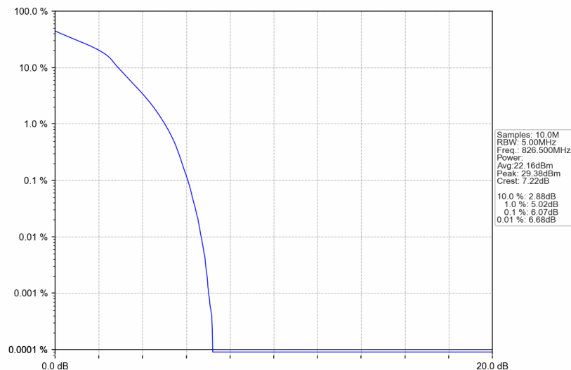
B26_5MHz_16QAM_LCH_826.5MHz_RB_25_0_NTNV
