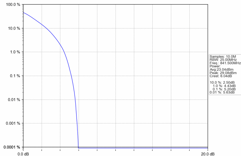
B26_15MHz_QPSK_HCH_841.5MHz_RB_75_0_NTNV
