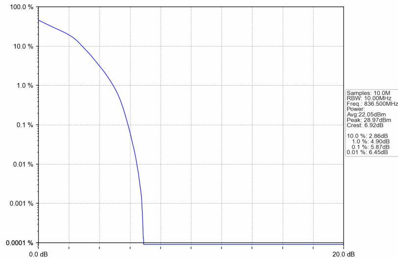
B26_10MHz_16QAM_MCH_836.5MHz_RB_50_0_NTNV
