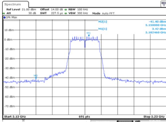
ANT 1(11AC20)
