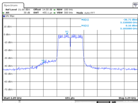
ANT 1(11N40)
