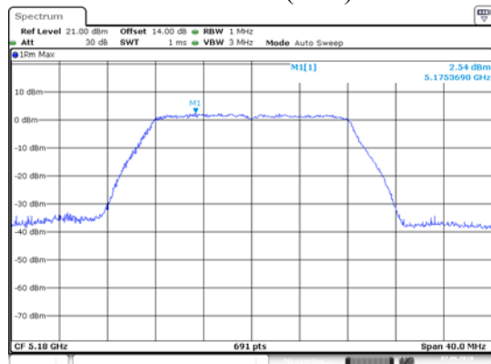
ANT 1(11A)
