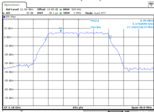
ANT 1(11A)
