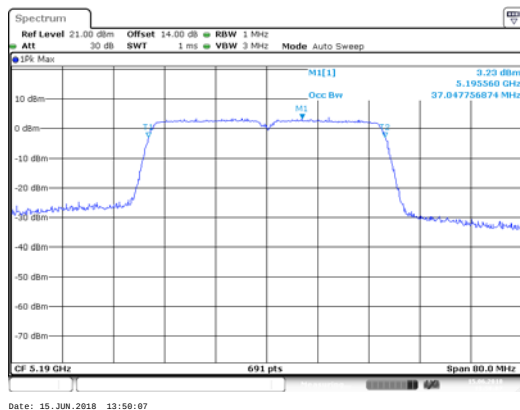
ANT 1(11N40)
