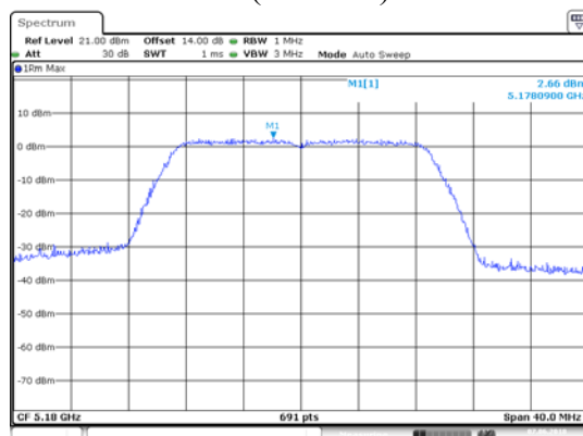
ANT 2(11AC20)
