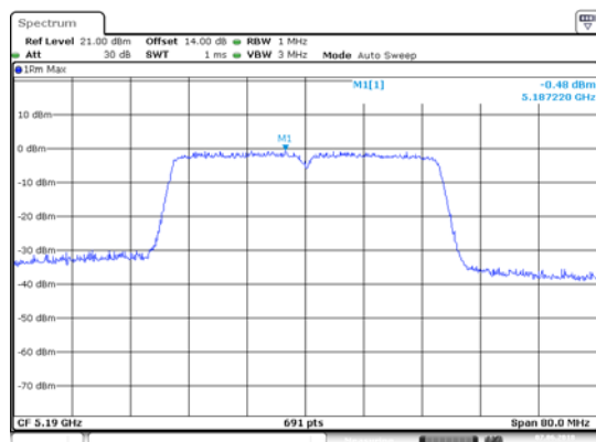
ANT 1(11N40)
