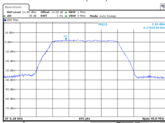
ANT 2(11A)
