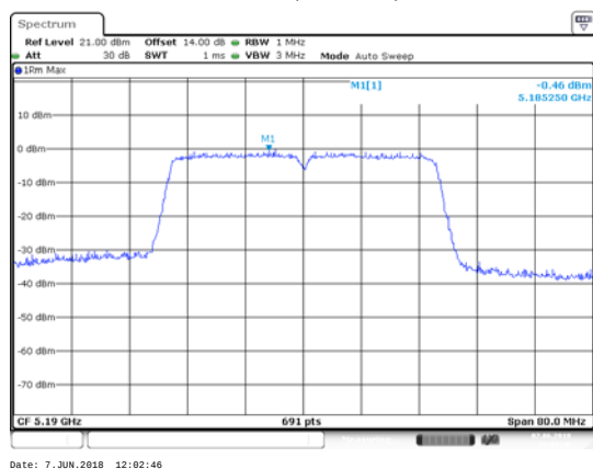
ANT 1(11N40)
