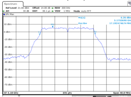
ANT 2(11A)
