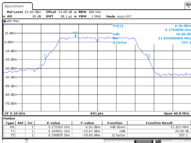
ANT 1(11A)
