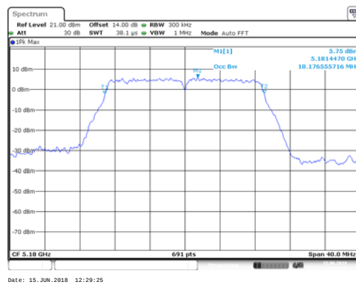
ANT 2(11AC20)
