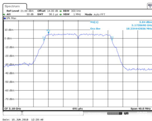
ANT 1(11AC20)
