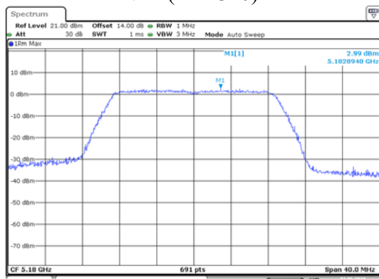
ANT 1(11AC20)
