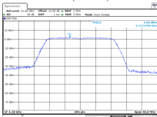
ANT 1(11AC20)
