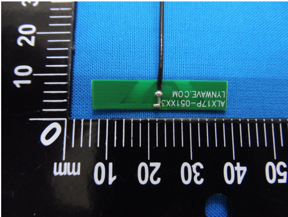
BLE Antenna 2 – Top View
