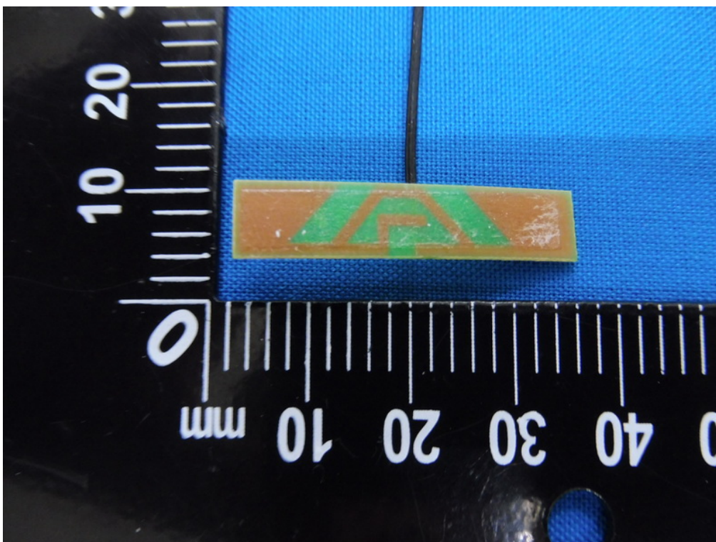
BLE Antenna 2 – Bottom View
