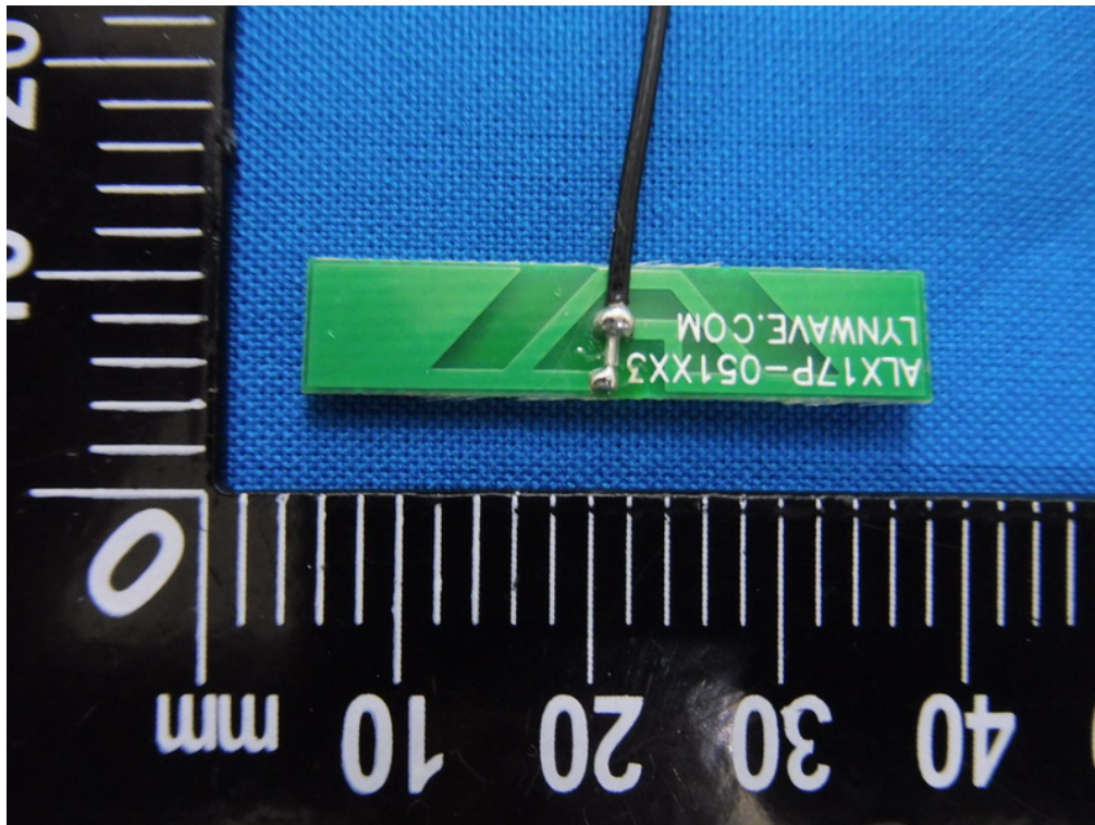
BLE Antenna 1 – Top View
