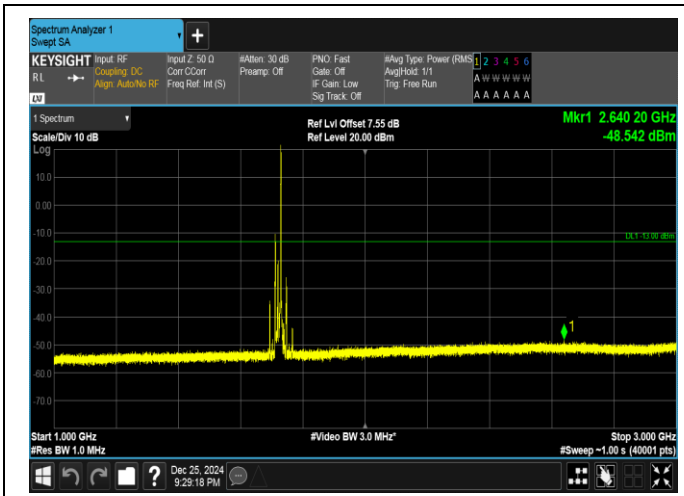
Band66-20MHz-QPSK-132072-1RB#99-1000~3000-PASS
