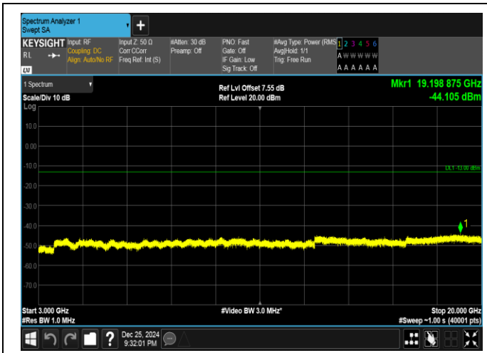
Band66-20MHz-QPSK-132072-100RB#0-3000~20000-PAS S
