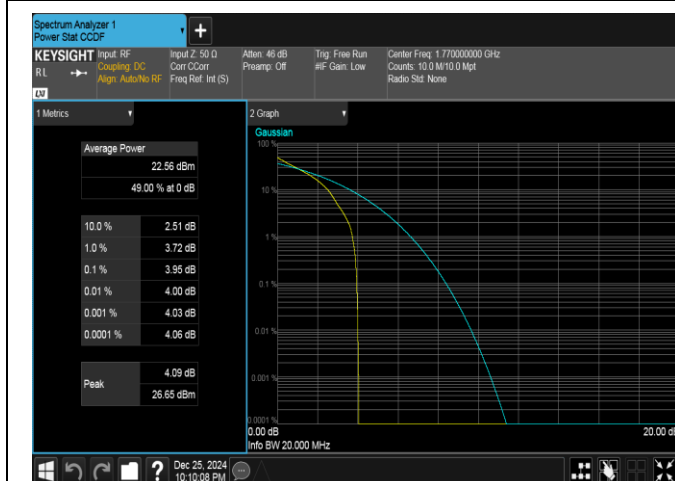
Band66-20MHz-QPSK-132572-1RB#0-PASS
