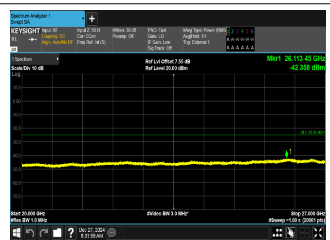
Band41-20MHz-QPSK-41490-1RB#99-20000~27000-PASS
