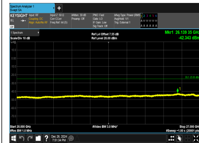
Band41-5MHz-QPSK-41565-1RB#0-20000~27000-PASS
