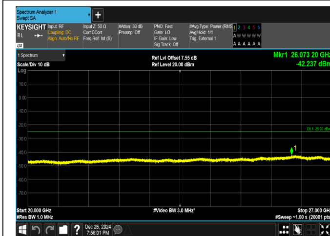
Band41-5MHz-16QAM-41565-1RB#24-20000~27000-PASS
