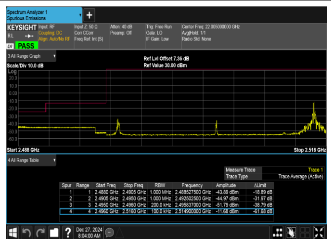
Band41-20MHz-QPSK-39750-1RB#99-PASS
