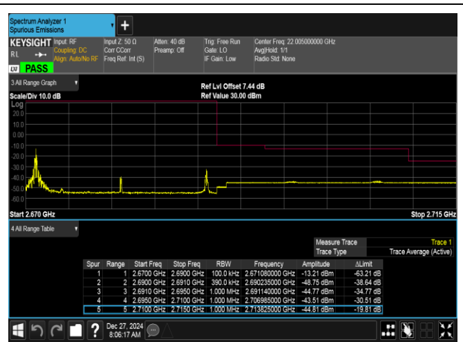
Band41-20MHz-QPSK-41490-1RB#0-PASS
