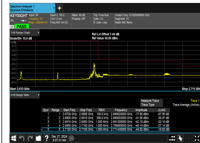
Band41-20MHz-QPSK-41490-1RB#99-PASS
