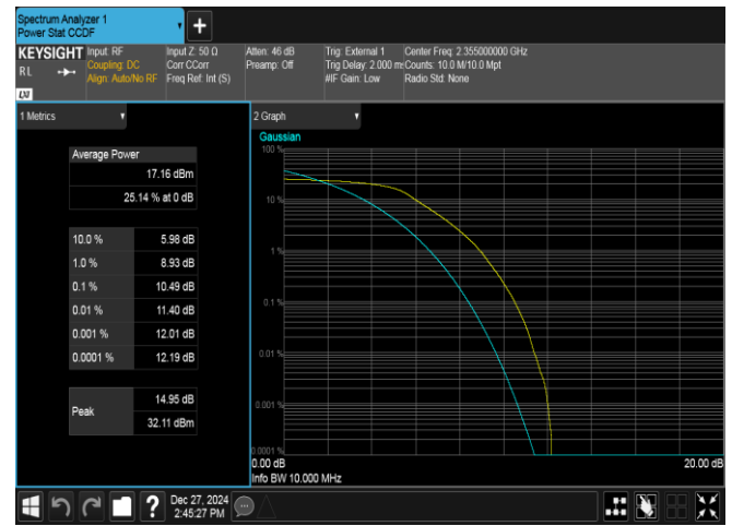
Band40(2350-2360)-10MHz-QPSK-39200-50RB#0-PASS
