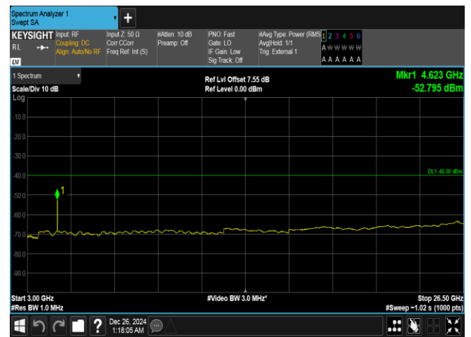
Band40(2305-2315)-10MHz-QPSK-38750-1RB#49-3000~26500-PASS
