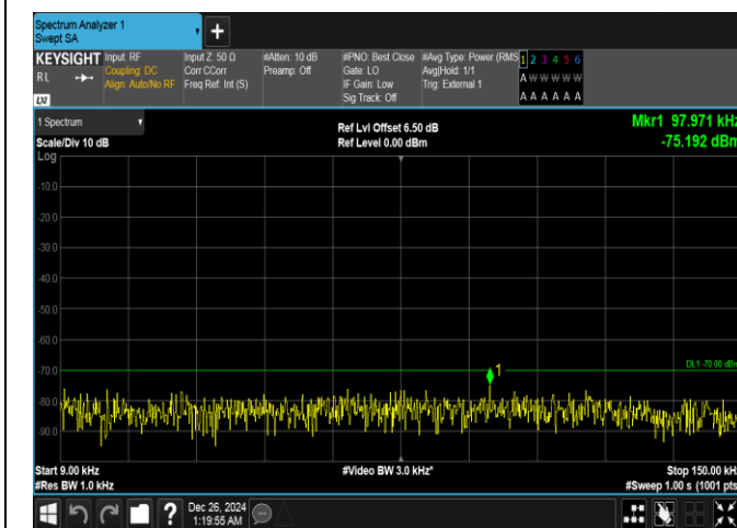
Band40(2305-2315)-10MHz-QPSK-38750-50RB#0-0.009~0.15-PASS
