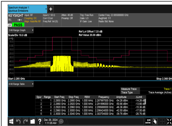
Band40(2305-2315)-10MHz-QPSK-38750-50RB#0-PASS
