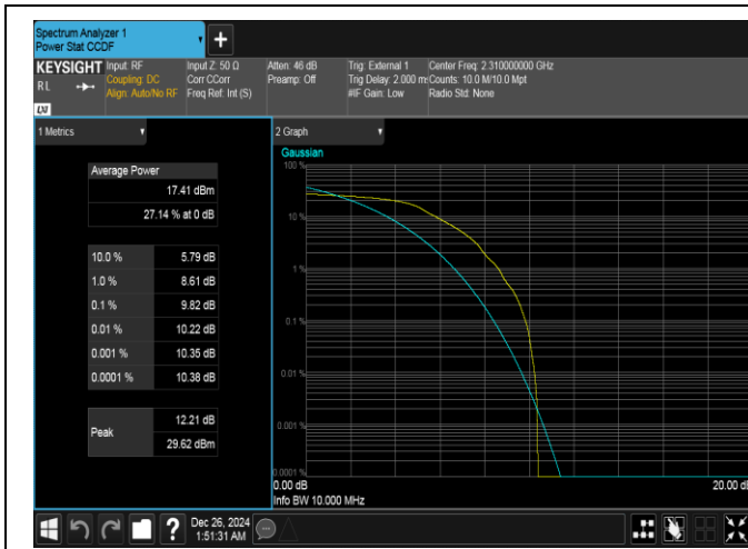
Band40(2305-2315)-10MHz-QPSK-38750-1RB#0-PASS
