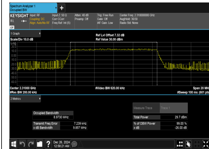
Band40(2305-2315)-10MHz-QPSK-38750-50RB#0-PASS
