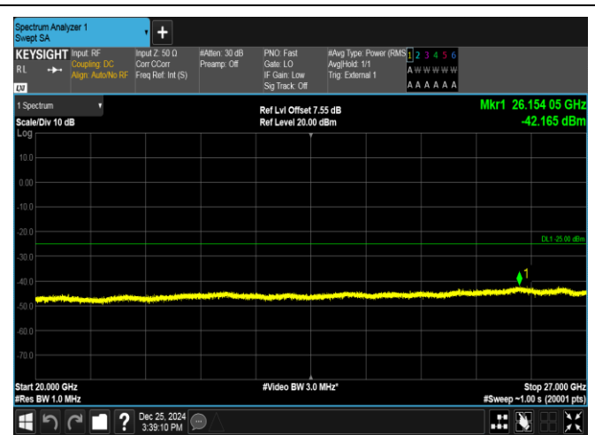
Band38-15MHz-QPSK-38175-1RB#74-20000~27000-PASS
