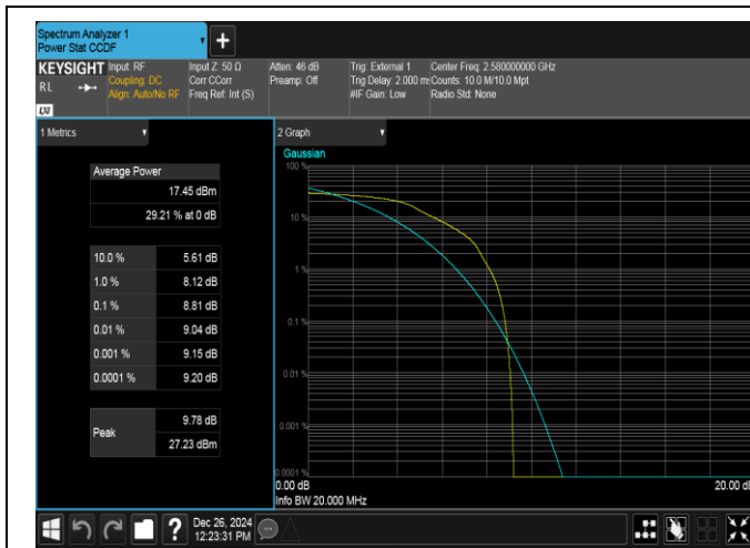
Band38-20MHz-QPSK-37850-1RB#0-PASS
