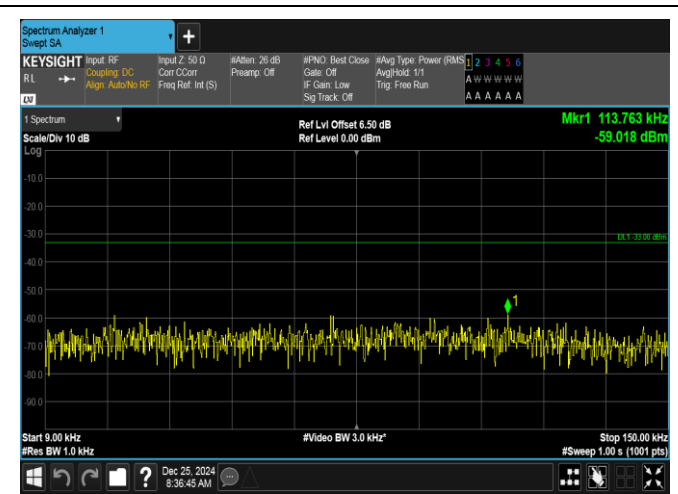
Band26(824-849)-3MHz-QPSK-26915-15RB#0-0.009~0.15-PASS
