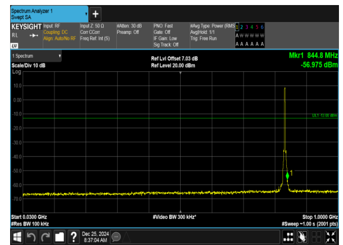
Band26(824-849)-3MHz-QPSK-26915-15RB#0-30~1000-PASS
