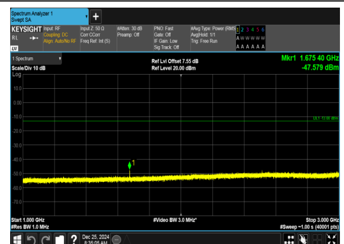
Band26(824-849)-3MHz-QPSK-26915-1RB#14-1000~3000-PASS
