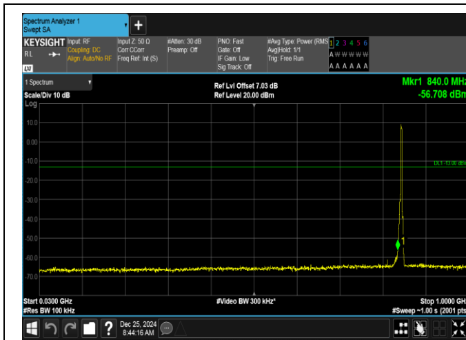
Band26(824-849)-3MHz-QPSK-27025-15RB#0-30~1000-PASS
