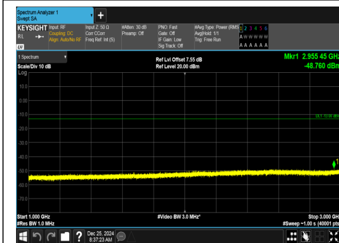
Band26(824-849)-3MHz-QPSK-26915-15RB#0-1000~3000-PASS
