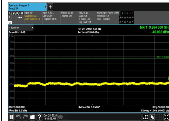
Band26(824-849)-3MHz-QPSK-27025-15RB#0-3000~10000-PASS
