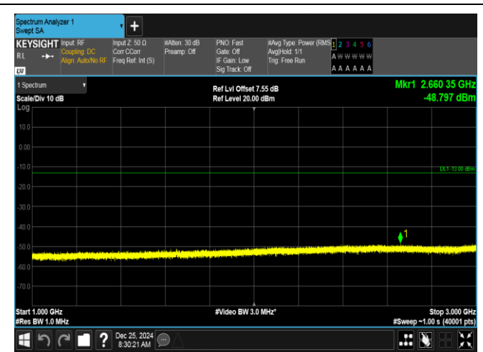
Band26(824-849)-3MHz-QPSK-26805-15RB#0-1000~3000-PASS
