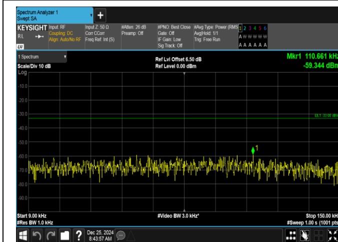
Band26(824-849)-3MHz-QPSK-27025-15RB#0-0.009~0.15-PASS
