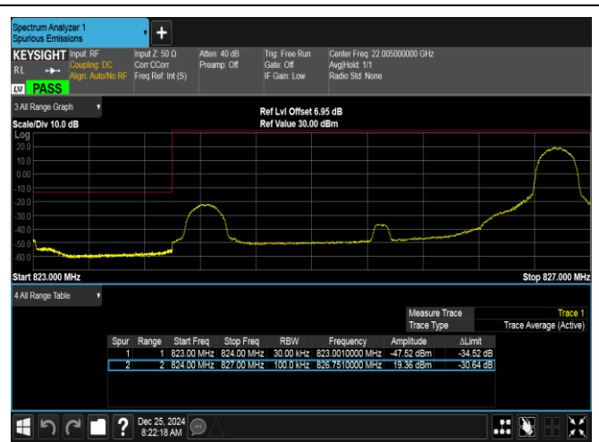
Band26(824-849)-3MHz-QPSK-26805-1RB#14-PASS
