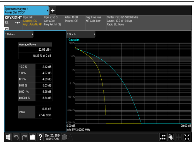
Band26(824-849)-3MHz-QPSK-26805-15RB#0-PASS
