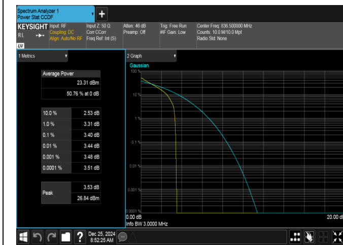
Band26(824-849)-3MHz-QPSK-26915-1RB#0-PASS
