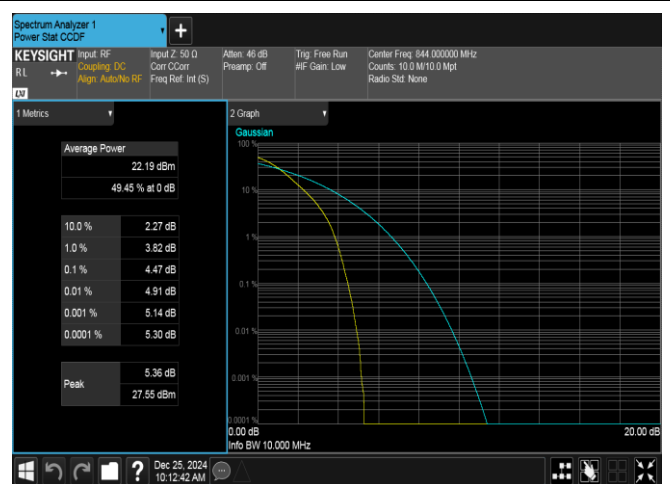
Band26(824-849)-10MHz-QPSK-26990-50RB#0-PASS
