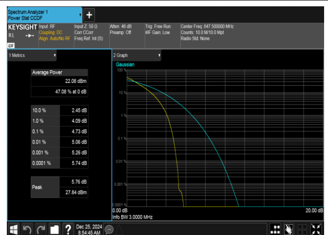
Band26(824-849)-3MHz-QPSK-27025-15RB#0-PASS
