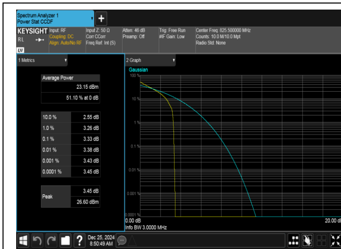
Band26(824-849)-3MHz-QPSK-26805-1RB#0-PASS
