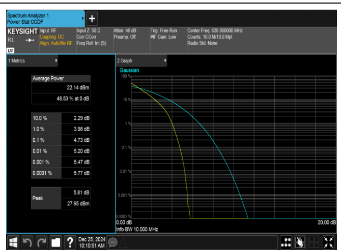
Band26(824-849)-10MHz-QPSK-26840-50RB#0-PASS
