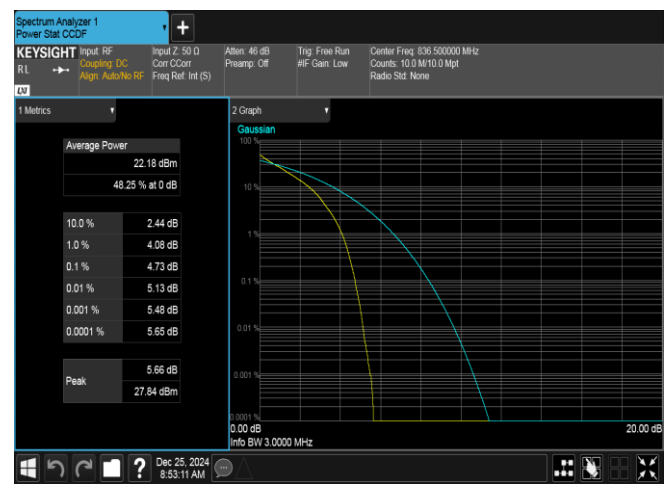
Band26(824-849)-3MHz-QPSK-26915-15RB#0-PASS
