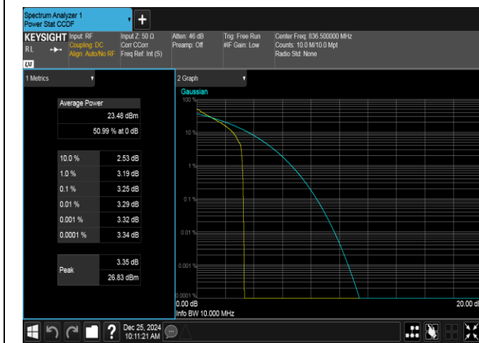
Band26(824-849)-10MHz-QPSK-26915-1RB#0-PASS
