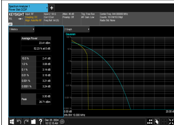
Band26(824-849)-10MHz-QPSK-26990-1RB#0-PASS
