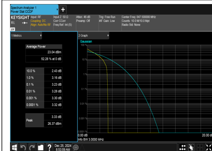
Band26(824-849)-3MHz-QPSK-27025-1RB#0-PASS
