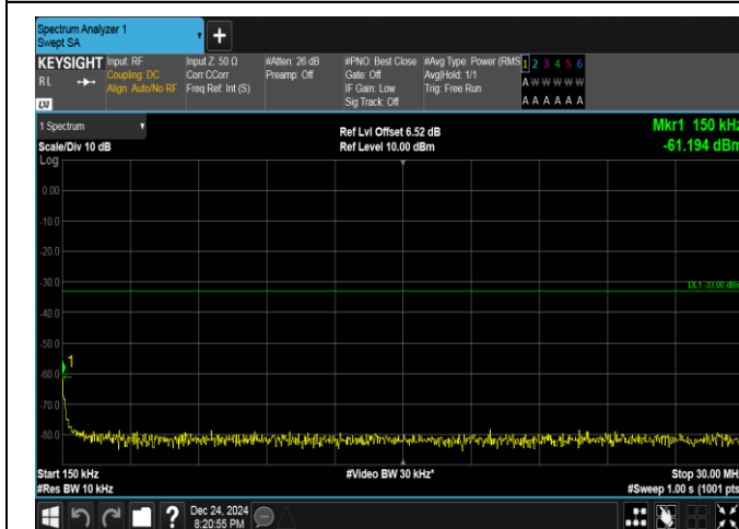
Band25-10MHz-QPSK-26365-1RB#0-0.15~30-PASS
