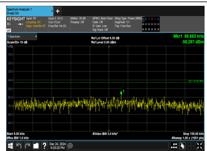
Band25-10MHz-QPSK-26365-50RB#0-0.009~0.15-PASS
