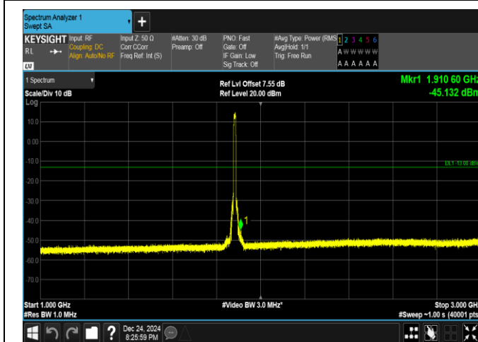
Band25-10MHz-QPSK-26365-50RB#0-1000~3000-PASS
