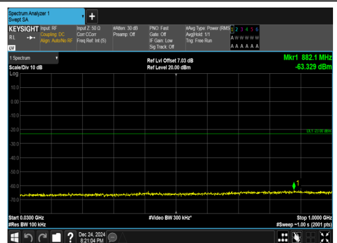
Band25-10MHz-QPSK-26365-1RB#0-30~1000-PASS
