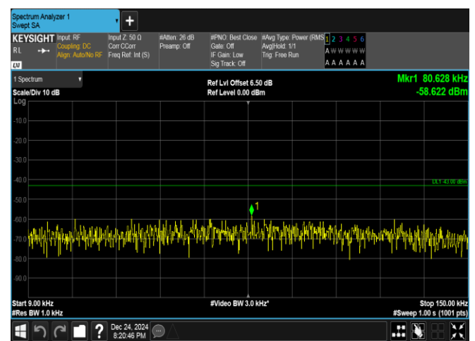
Band25-10MHz-QPSK-26365-1RB#0-0.009~0.15-PASS
