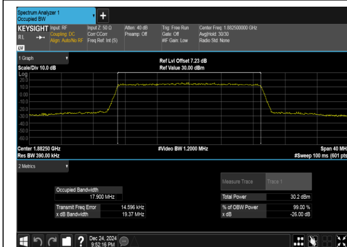
Band25-20MHz-16QAM-26365-100RB#0-PASS
