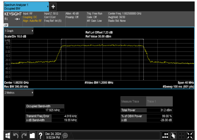
Band25-20MHz-QPSK-26365-100RB#0-PASS
