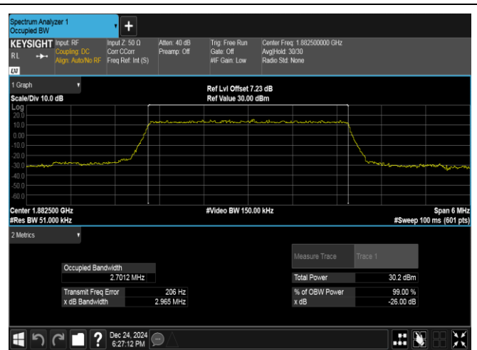
Band25-3MHz-QPSK-26365-15RB#0-PASS
