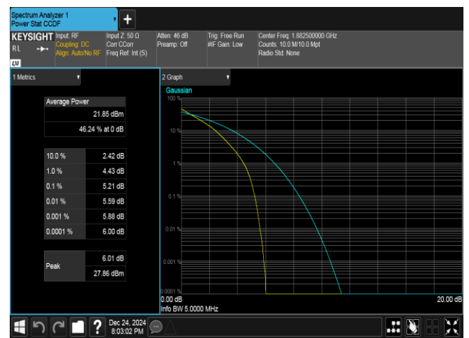
Band25-5MHz-QPSK-26365-25RB#0-PASS
