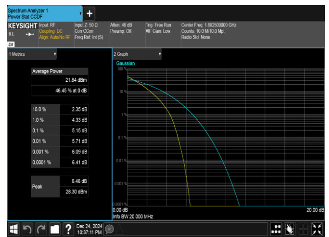
Band25-20MHz-QPSK-26365-100RB#0-PASS
