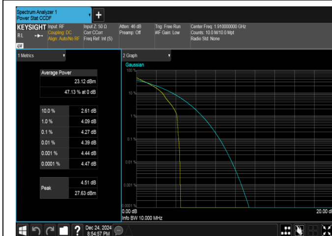
Band25-10MHz-QPSK-26640-1RB#0-PASS
