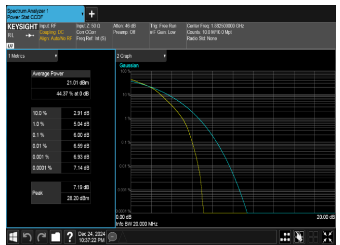
Band25-20MHz-16QAM-26365-100RB#0-PASS
