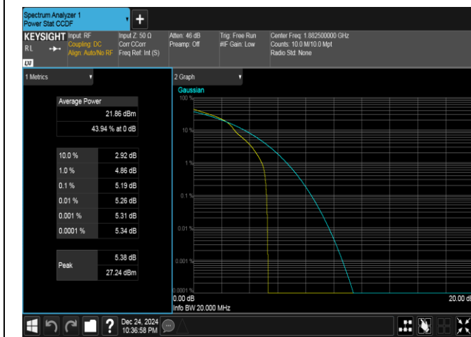
Band25-20MHz-16QAM-26365-1RB#0-PASS
