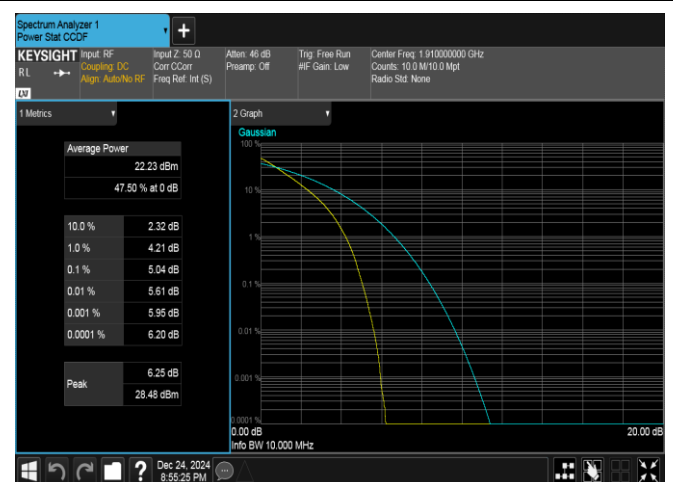
Band25-10MHz-QPSK-26640-50RB#0-PASS
