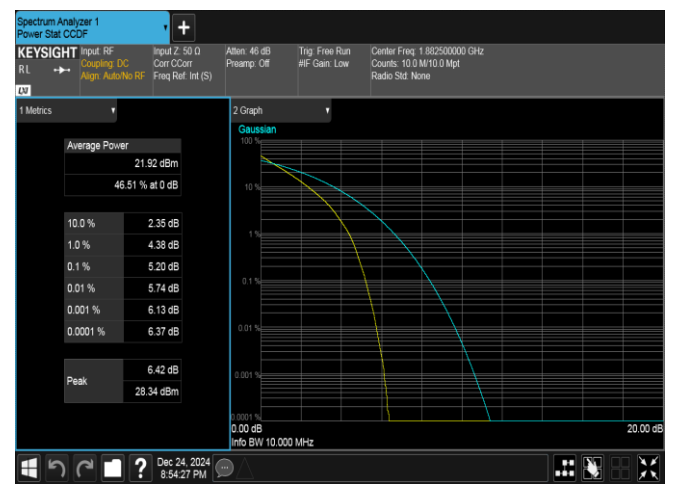
Band25-10MHz-QPSK-26365-50RB#0-PASS
