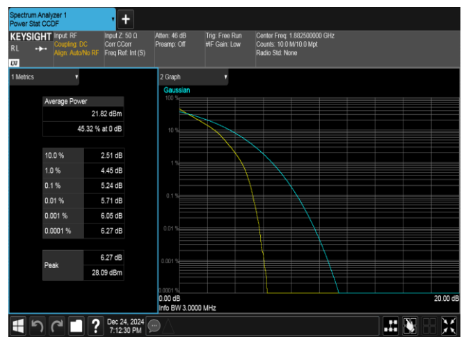
Band25-3MHz-QPSK-26365-15RB#0-PASS
