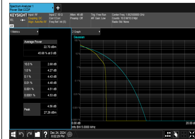
Band25-5MHz-QPSK-26365-1RB#0-PASS
