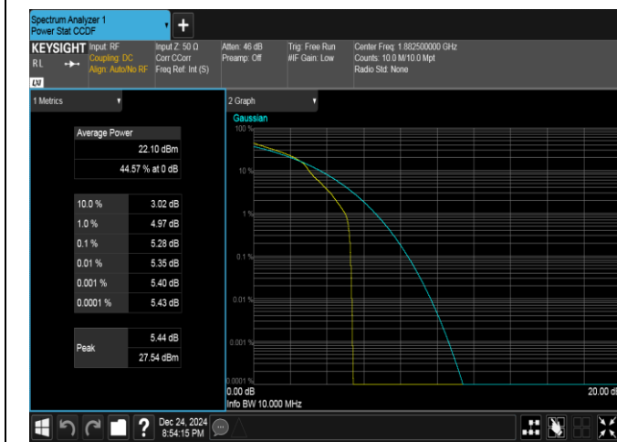
Band25-10MHz-16QAM-26365-1RB#0-PASS
