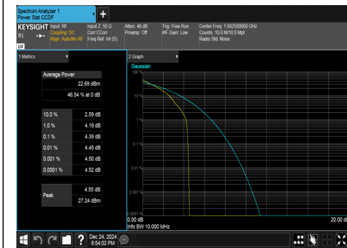
Band25-10MHz-QPSK-26365-1RB#0-PASS
