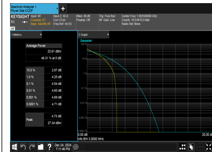
Band25-3MHz-QPSK-26365-1RB#0-PASS
