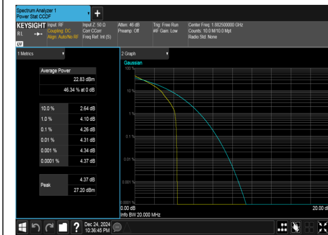
Band25-20MHz-QPSK-26365-1RB#0-PASS
