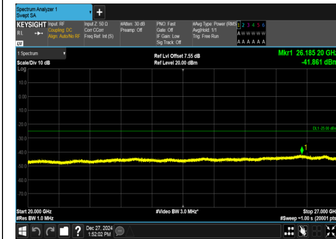
Band7-20MHz-QPSK-20850-1RB#0-20000~27000-PASS
