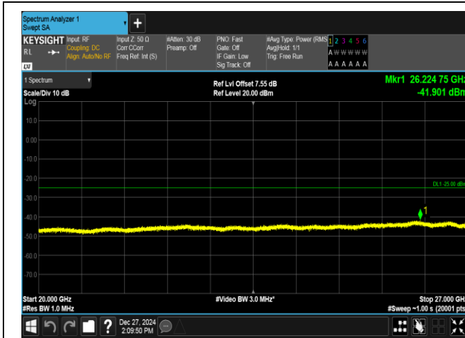
Band7-20MHz-QPSK-21350-100RB#0-20000~27000-PASS
