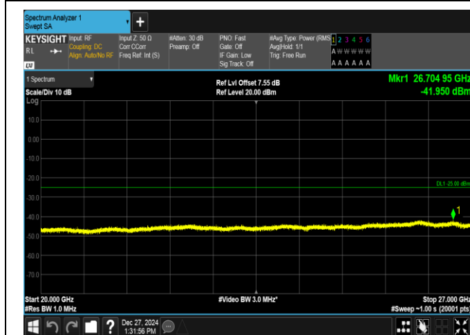
Band7-15MHz-QPSK-20825-1RB#0-20000~27000-PASS
