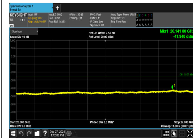
Band7-10MHz-QPSK-20800-1RB#0-20000~27000-PASS
