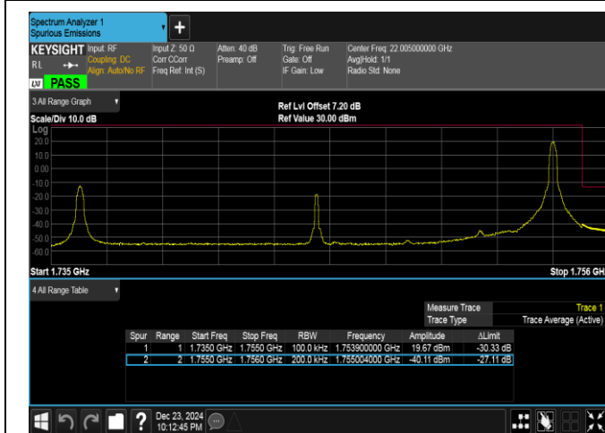
Band4-20MHz-QPSK-20300-1RB#99-PASS
