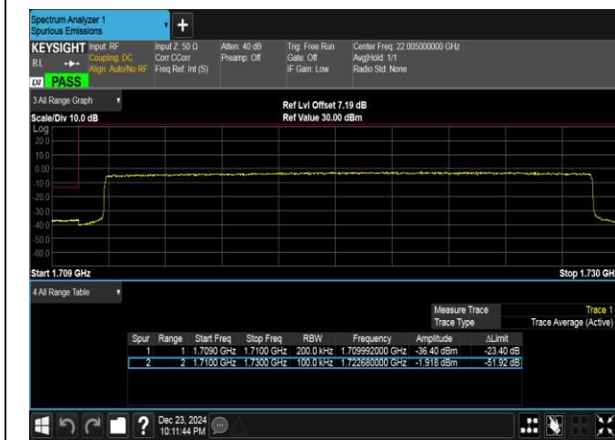
Band4-20MHz-QPSK-20050-100RB#0-PASS
