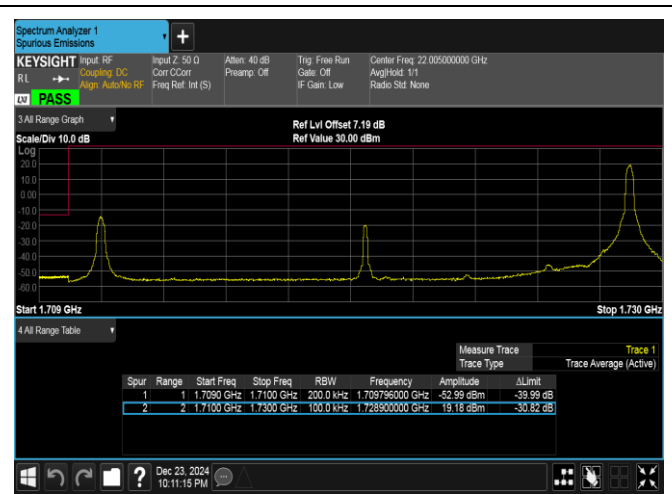
Band4-20MHz-QPSK-20050-1RB#99-PASS
