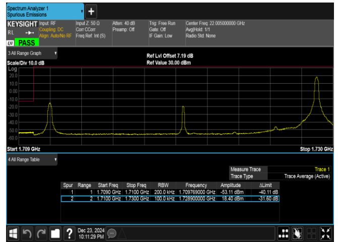
Band4-20MHz-16QAM-20050-1RB#99-PASS
