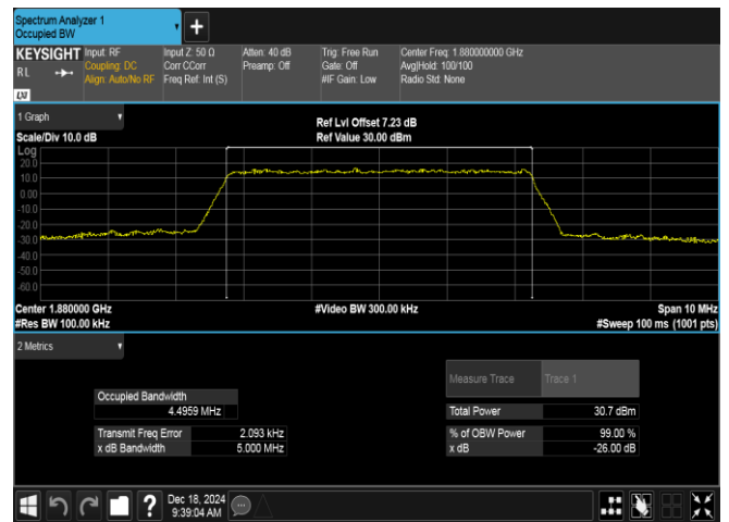
Band2-5MHz-QPSK-18900-25RB#0-PASS
