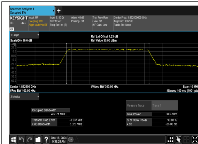
Band2-5MHz-QPSK-18625-25RB#0-PASS
