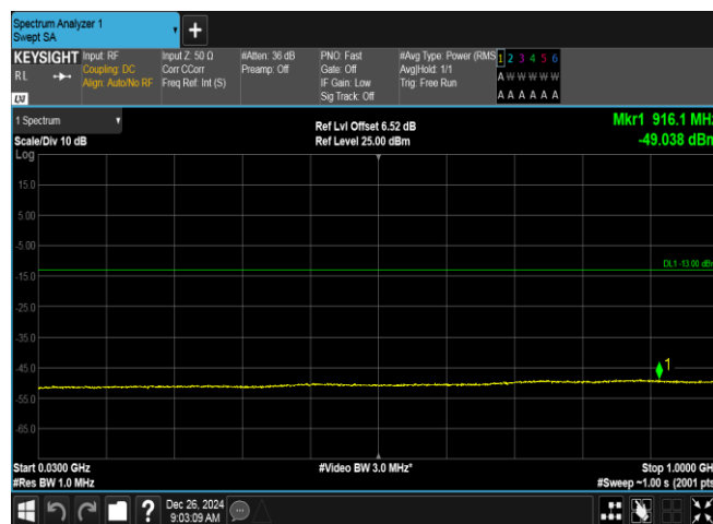
Band2-9538-1-30~1000MHz-PASS
