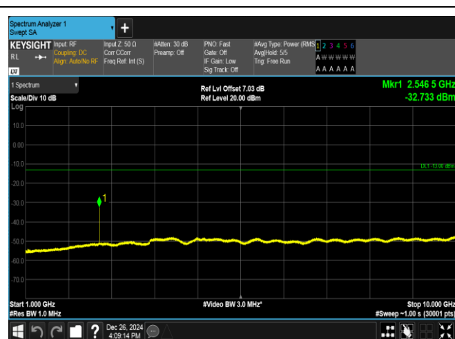
GPRS850-251-5-1000~10000MHz-PASS
