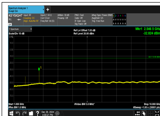
GSM850-251-5-1000~10000MHz-PASS
