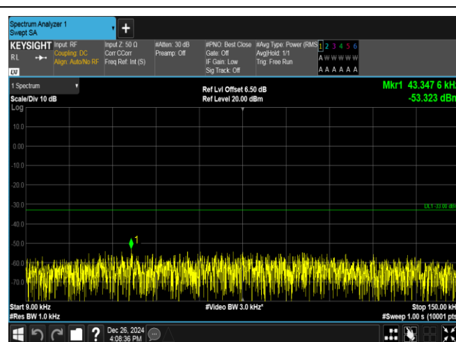
GPRS850-251-5-0.009~0.15MHz-PASS
