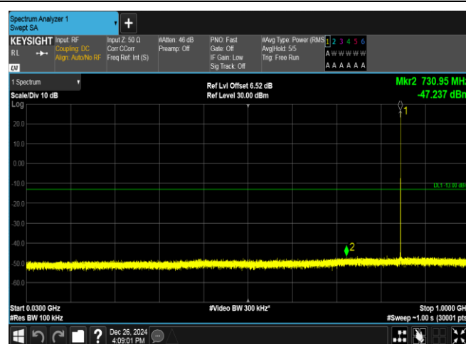
GPRS850-251-5-30~1000MHz-PASS
