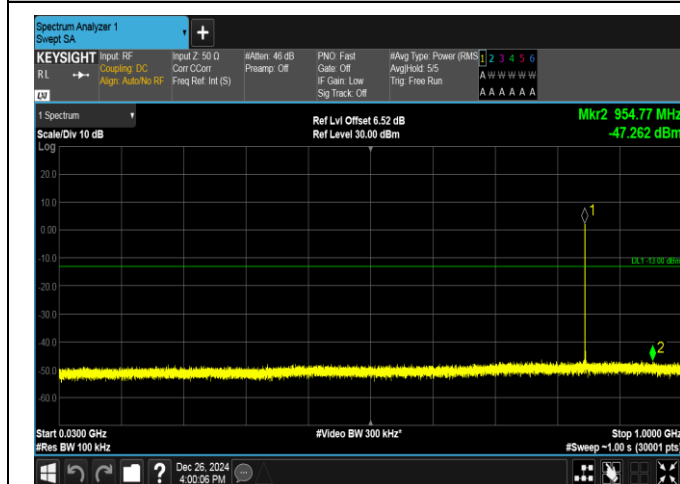
GSM850-251-5-30~1000MHz-PASS
