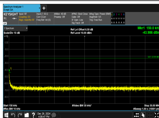
GPRS850-251-5-0.15~30MHz-PASS
