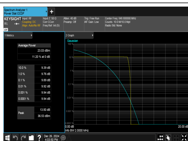
GPRS850-251-5-PASS
