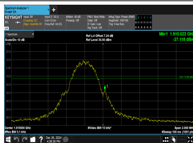
GSM1900-810-0-PASS
