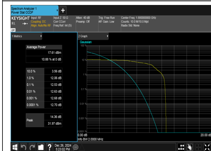
EGPRS1900-661-2-PASS
