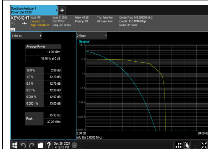
EGPRS850-251-8-PASS
