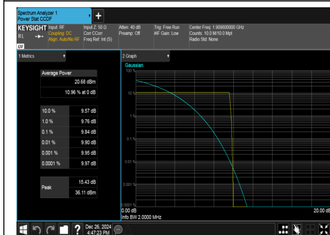
GPRS1900-810-0-PASS
