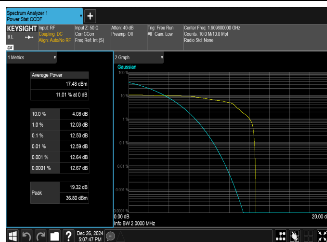
EGPRS1900-810-2-PASS
