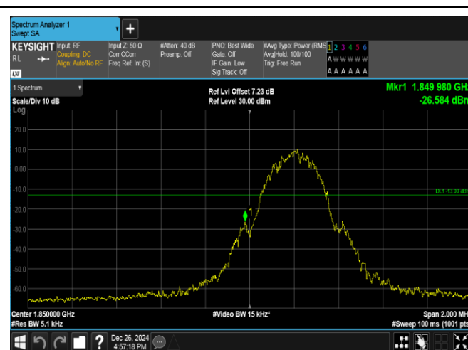
GPRS1900-512-0-PASS
