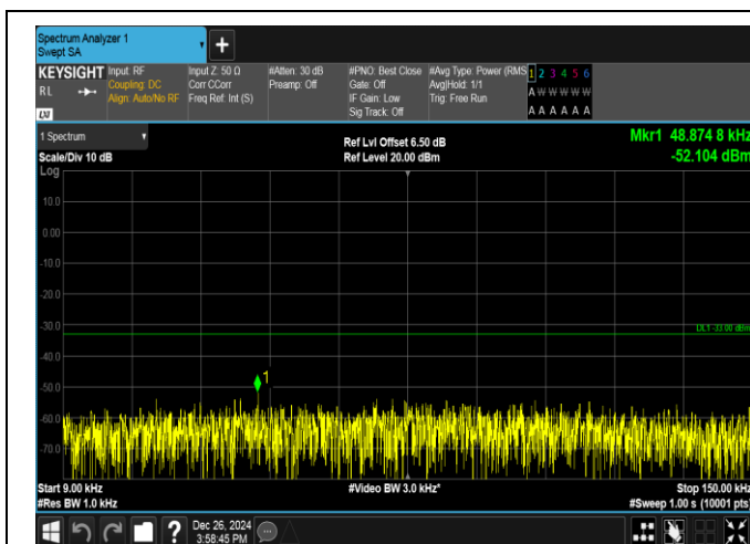
GSM850-190-5-0.009~0.15MHz-PASS
