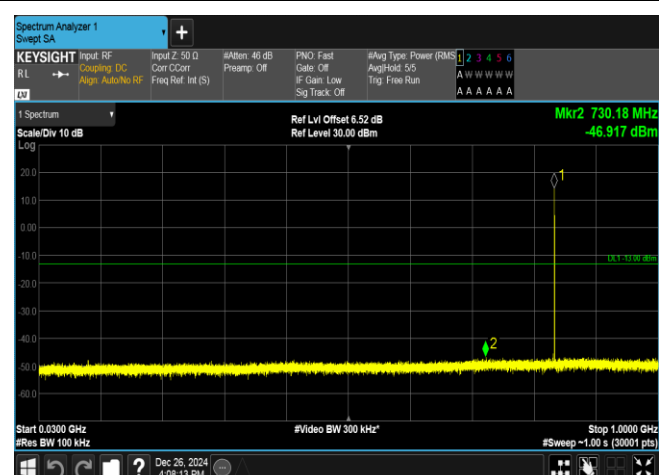
GPRS850-190-5-30~1000MHz-PASS
