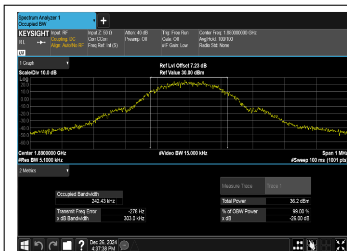
GSM1900-661-0-PASS
