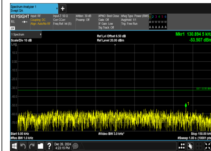
EGPRS850-190-8-0.009~0.15MHz-PASS
