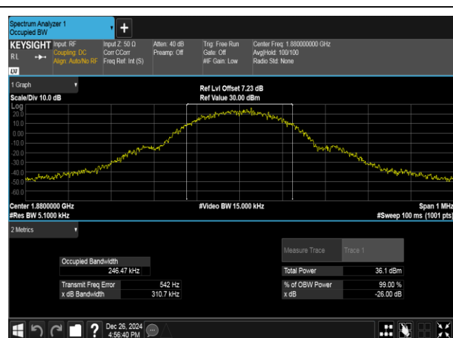
GPRS1900-661-0-PASS
