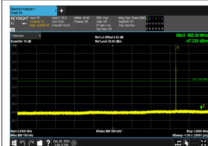
GSM850-190-5-30~1000MHz-PASS
