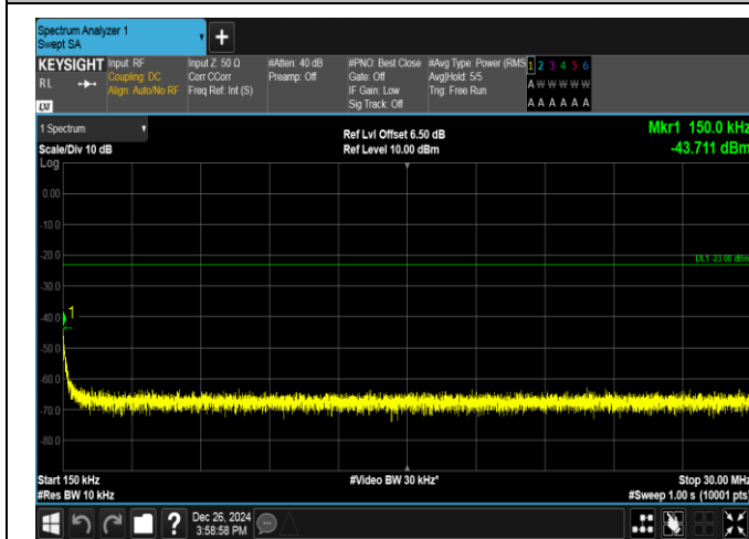
GSM850-190-5-0.15~30MHz-PASS
