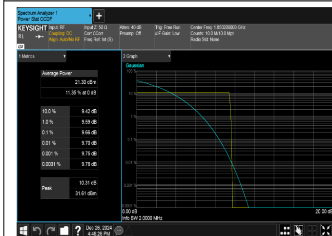
GPRS1900-512-0-PASS
