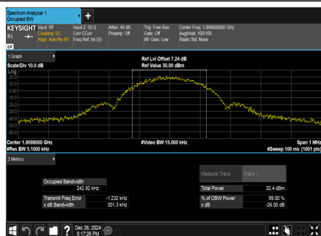
EGPRS1900-810-2-PASS
