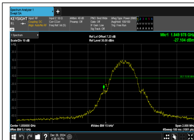
GSM1900-512-0-PASS
