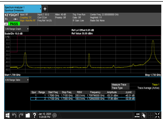
Band66-20MHz-QPSK-132072-1RB#99-PASS
