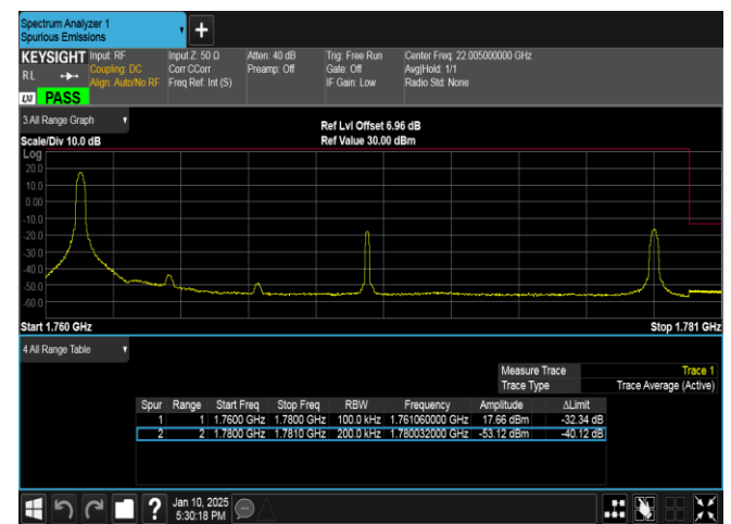
Band66-20MHz-QPSK-132572-1RB#0-PASS
