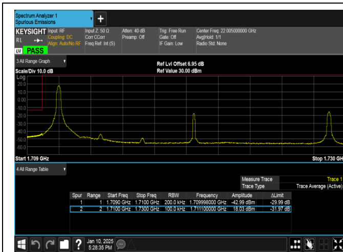
Band66-20MHz-QPSK-132072-1RB#0-PASS
