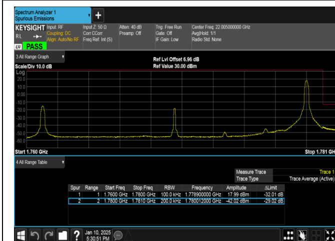
Band66-20MHz-QPSK-132572-1RB#99-PASS
