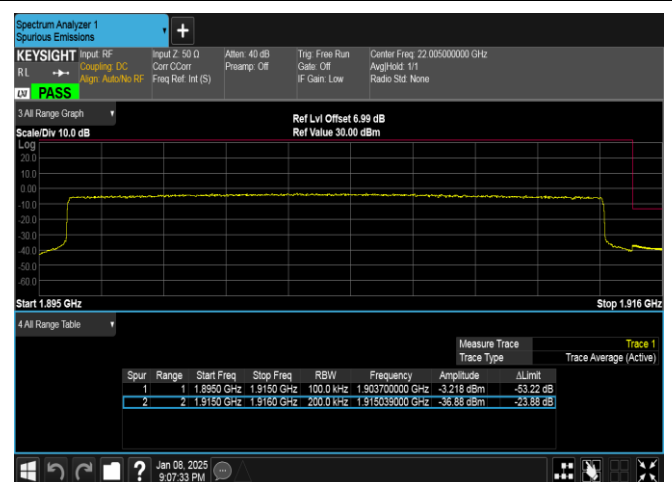
Band25-20MHz-QPSK-26590-100RB#0-PASS
