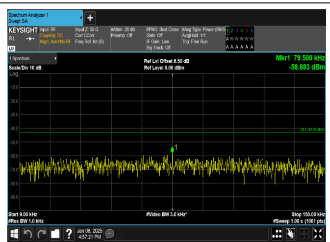
Band25-1.4MHz-QPSK-26365-6RB#0-0.009~0.15-PASS
