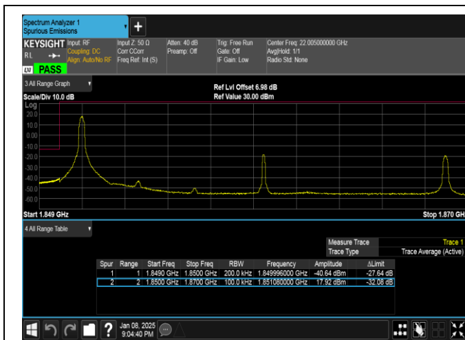
Band25-20MHz-QPSK-26140-1RB#0-PASS
