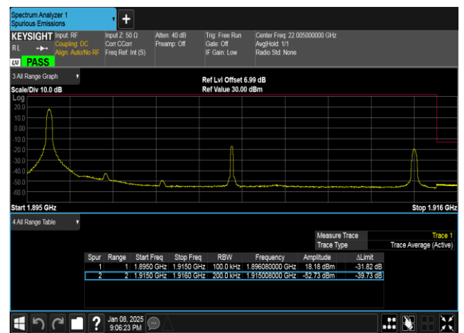
Band25-20MHz-QPSK-26590-1RB#0-PASS
