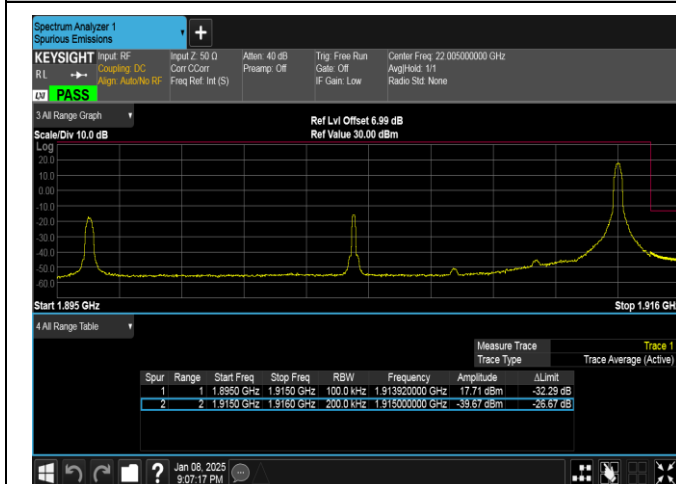
Band25-20MHz-16QAM-26590-1RB#99-PASS
