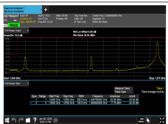
Band25-20MHz-QPSK-26140-1RB#99-PASS
