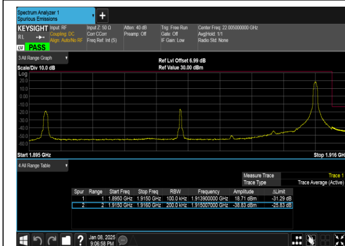
Band25-20MHz-QPSK-26590-1RB#99-PASS
