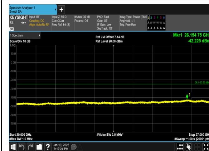
Band41-15MHz-16QAM-41515-1RB#74-20000~27000-PASS
