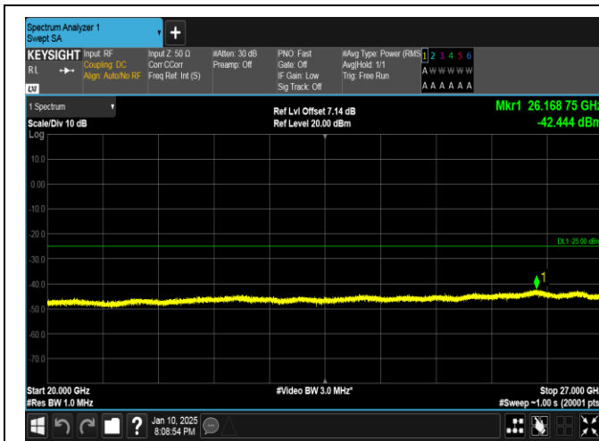
Band41-10MHz-QPSK-41540-50RB#0-20000~27000-PASS
