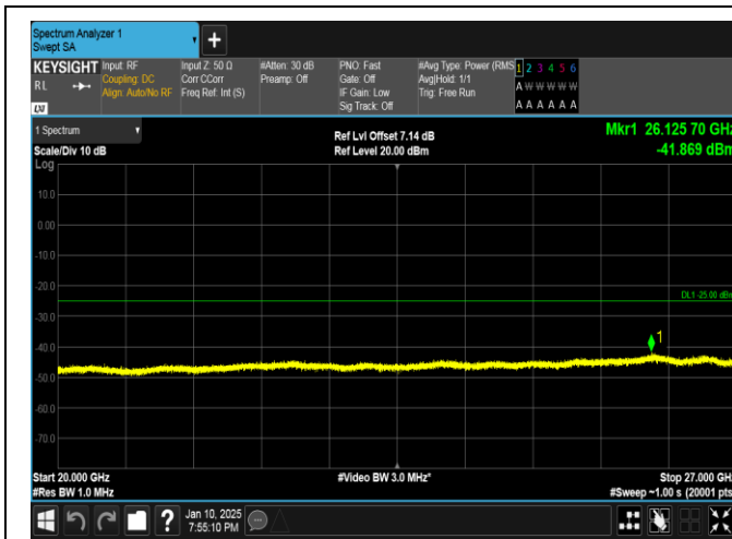
Band41-10MHz-QPSK-39700-50RB#0-20000~27000-PASS
