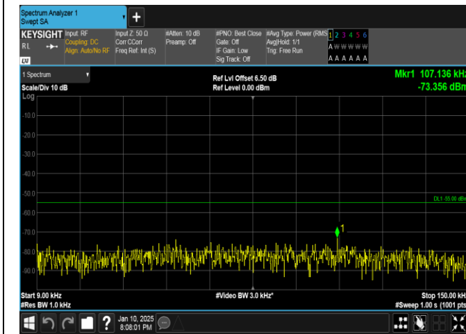
Band41-10MHz-QPSK-41540-50RB#0-0.009~0.15-PASS
