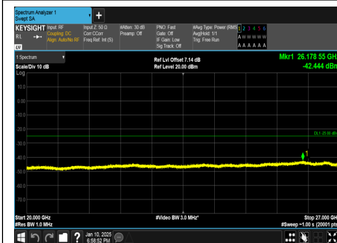
Band41-5MHz-16QAM-41565-1RB#24-20000~27000-PASS
