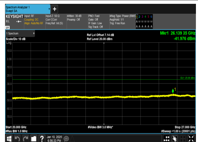
Band41-5MHz-16QAM-41565-1RB#0-20000~27000-PASS
