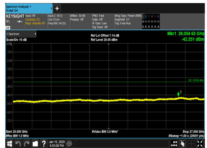
Band41-5MHz-QPSK-40620-25RB#0-20000~27000-PASS
