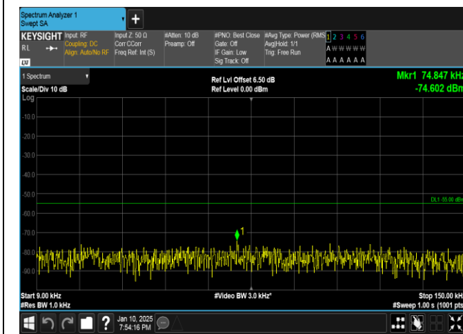
Band41-10MHz-QPSK-39700-50RB#0-0.009~0.15-PASS
