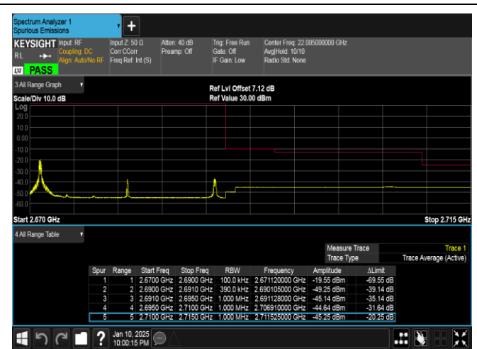
Band41-20MHz-QPSK-41490-1RB#0-PASS
