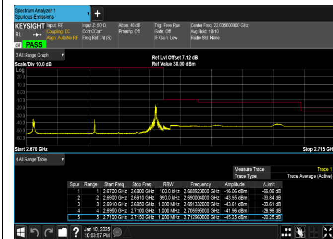
Band41-20MHz-QPSK-41490-1RB#99-PASS
