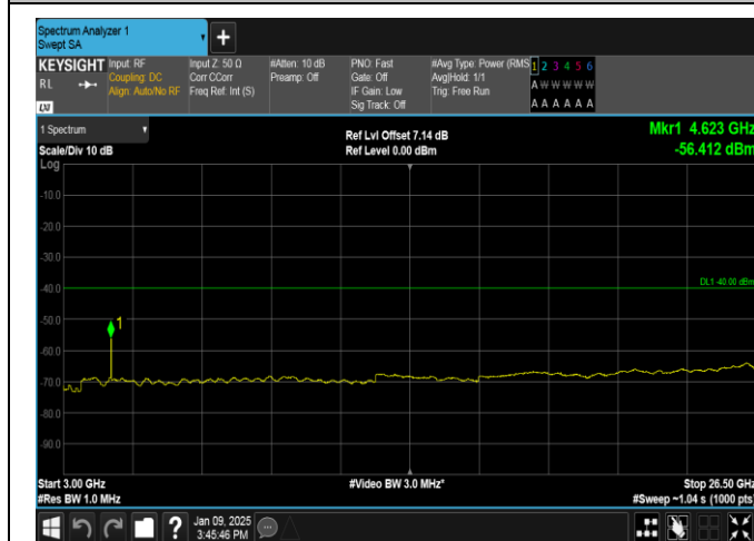
Band40(2305-2315)-10MHz-QPSK-38750-50RB#0-3000~26500-PASS
