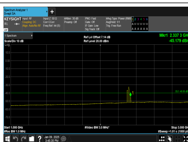
Band40(2305-2315)-10MHz-QPSK-38750-50RB#0-1000~3000-PASS
