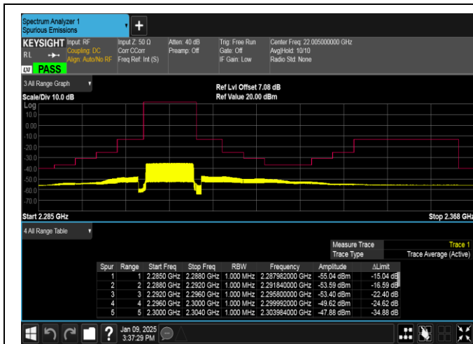
Band40(2305-2315)-10MHz-QPSK-38750-50RB#0-PASS
