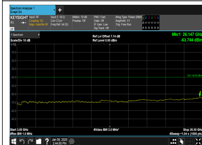
Band40(2305-2315)-5MHz-QPSK-38725-25RB#0-3000~26500-PASS
