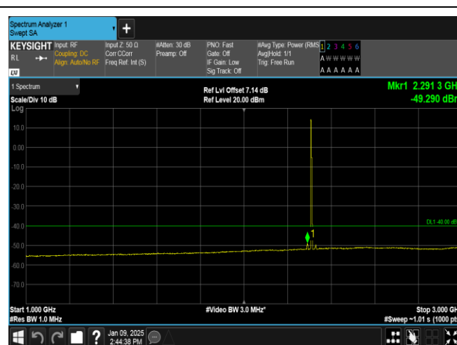
Band40(2305-2315)-5MHz-QPSK-38725-25RB#0-1000~3000-PASS
