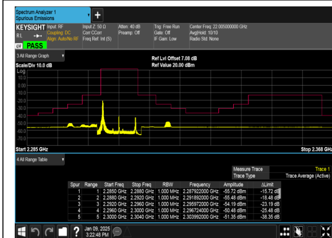
Band40(2305-2315)-10MHz-QPSK-38750-1RB#0-PASS
