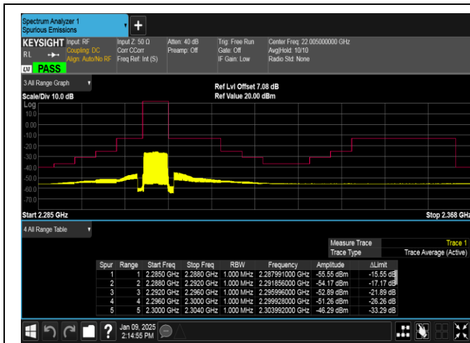
Band40(2305-2315)-5MHz-QPSK-38725-25RB#0-PASS
