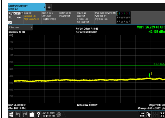
Band38-20MHz-QPSK-38150-1RB#0-20000~27000-PASS
